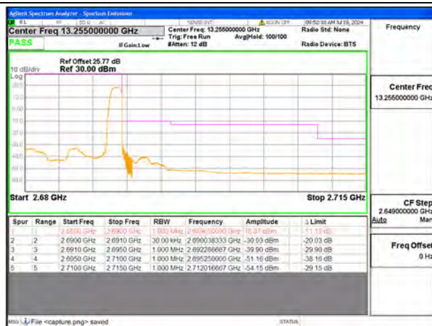
B41 / 10MHz / High CH / QPSK / 1 RB
