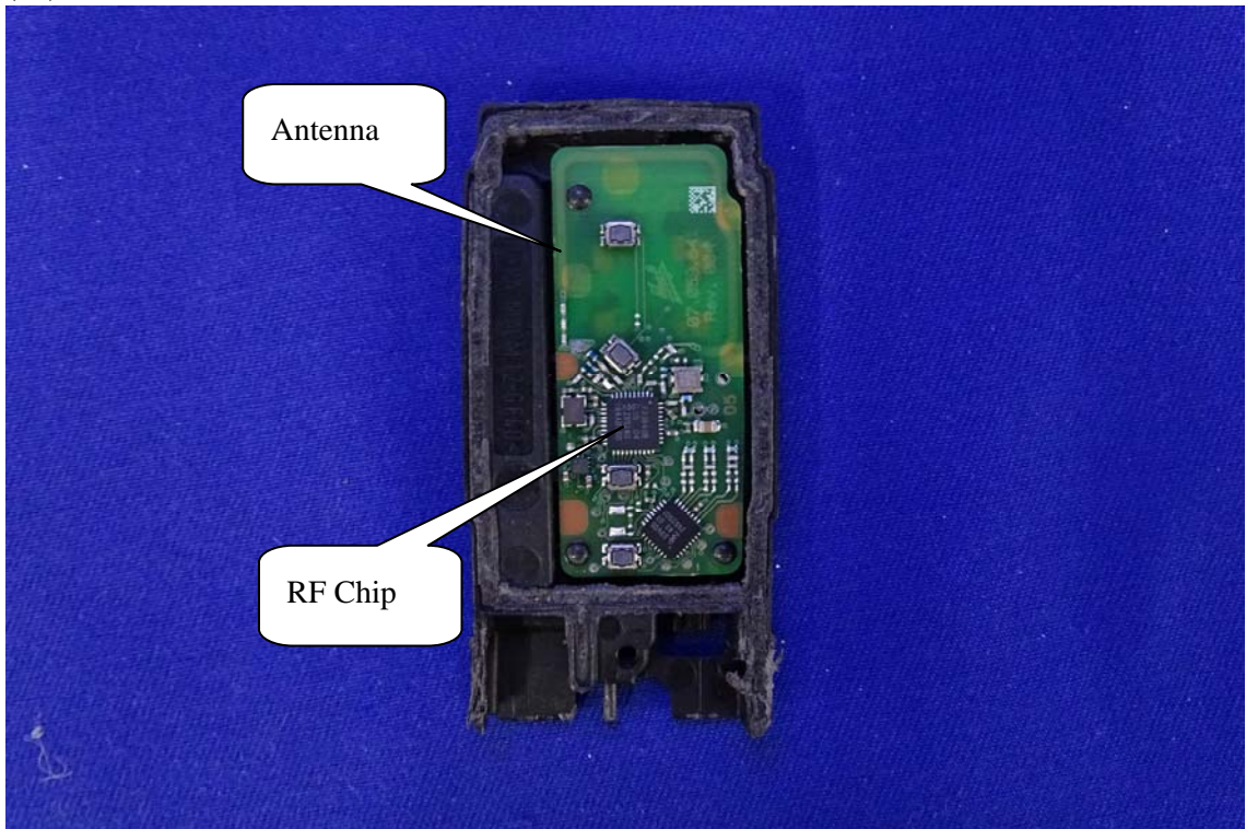
(20) EUT Photo
