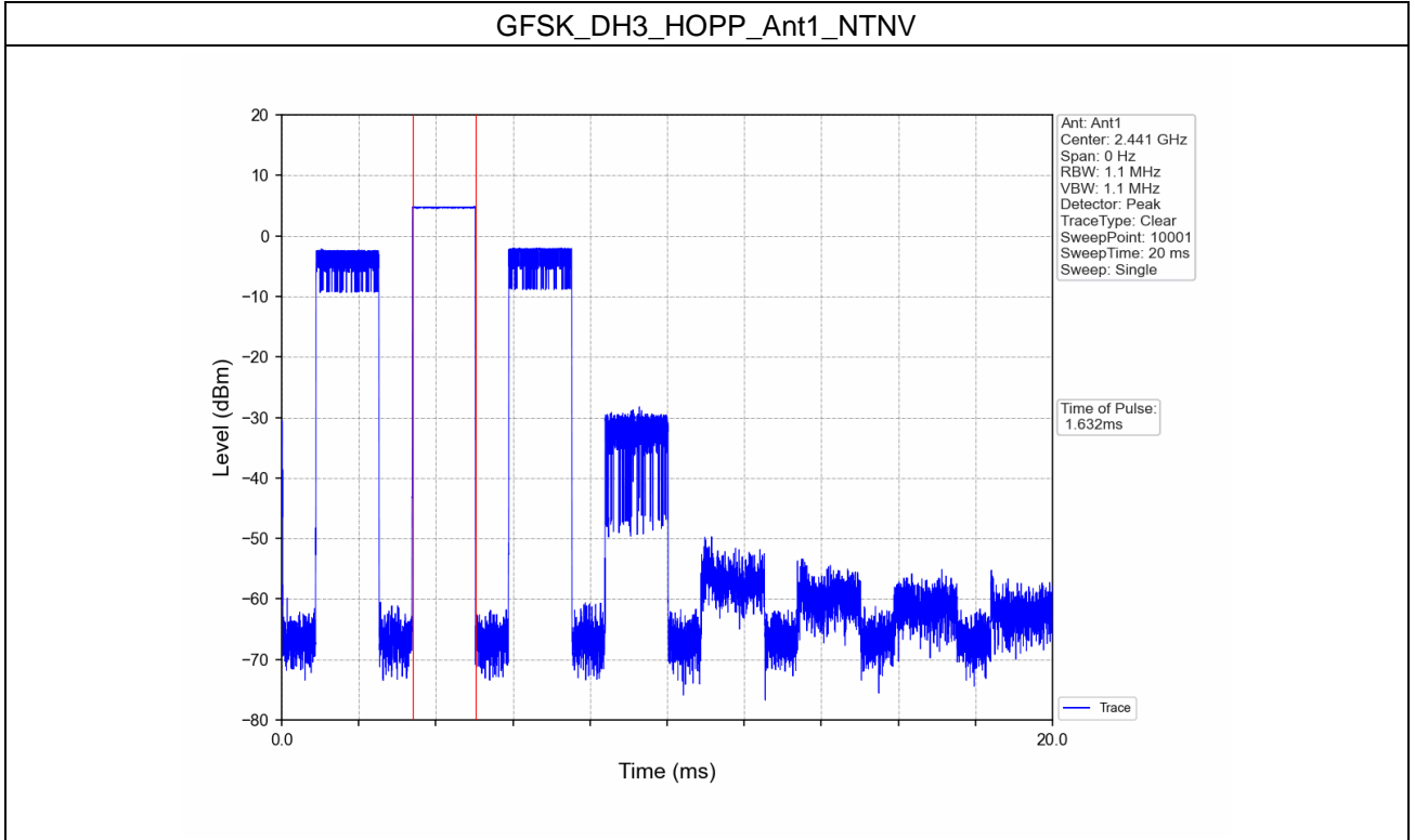
GFSK_DH3_HOPP_Ant1_NTNV
