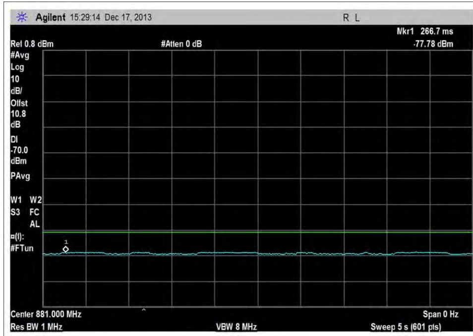
DL_869-894MHz_Single_-70dBm
