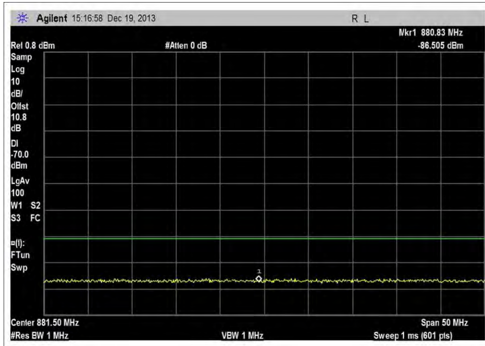
DL_869-894MHz_MNC260
