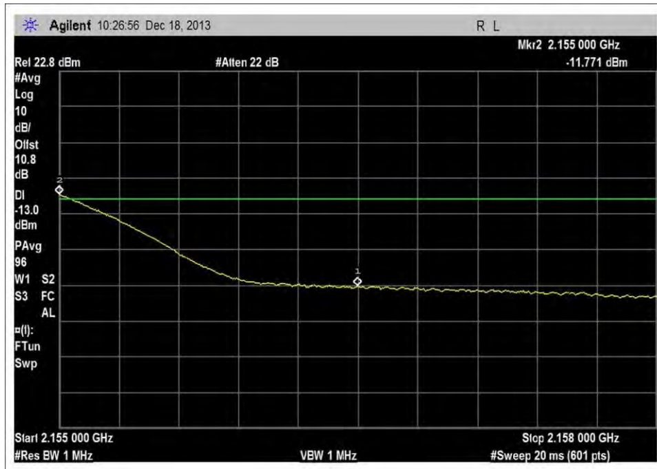
DL_2110-2155MHz_H_-20dBm
