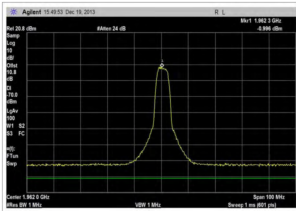
DL_1930-1995MHz_MNC410
