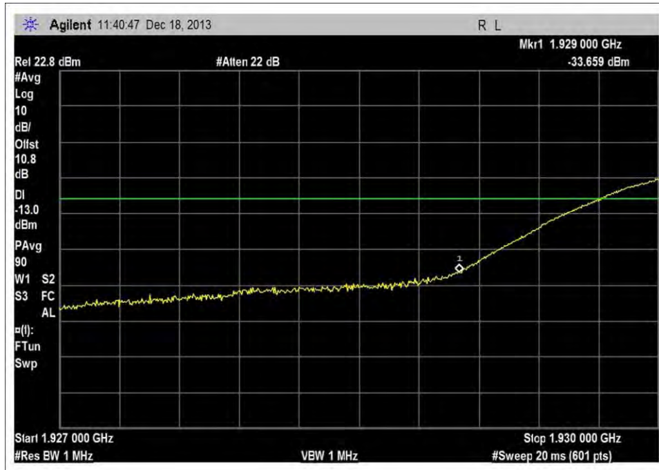
DL_1930-1995MHz_L_-90dBm
