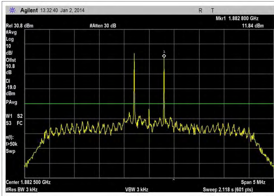
UL_1850-1915MHz_-60dBm
