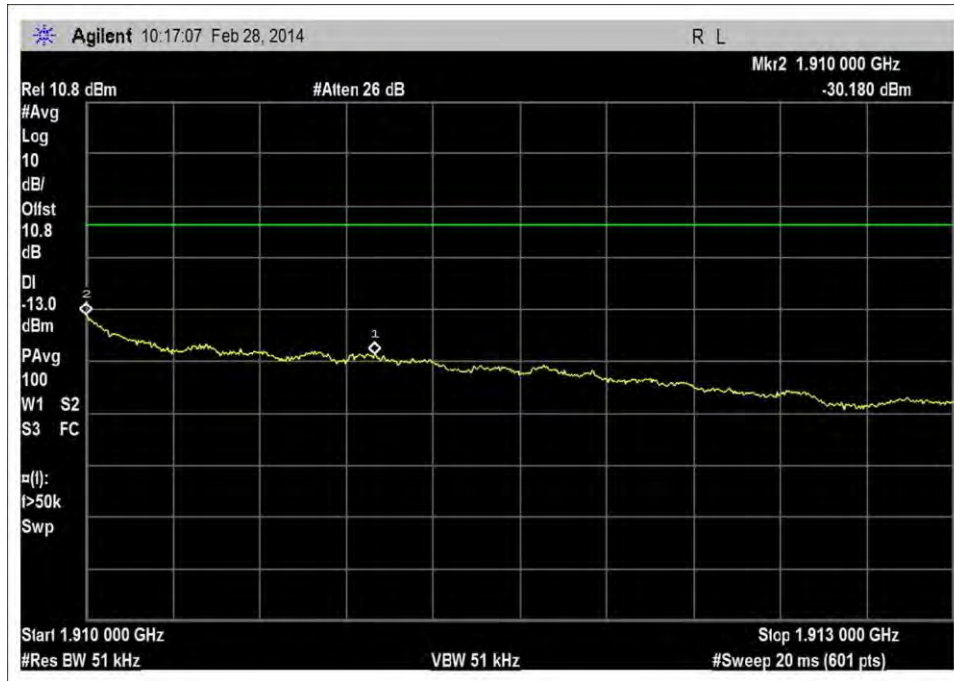
UL_1850-1915MHz_H_RFin -78dBm_rbw=51kHz
