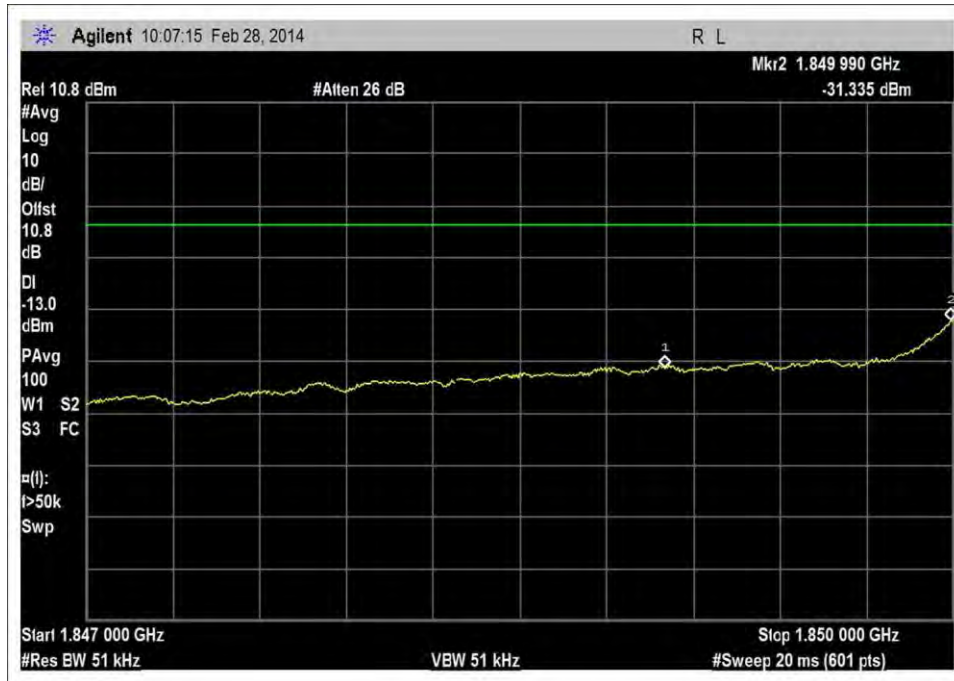
UL_1850-1915MHz_L_RFin -78dBm_rbw=51kHz
