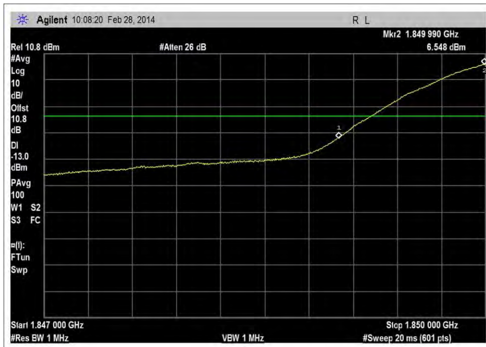
UL_1850-1915MHz_L_RFin OdBm_rbw=1MHz
