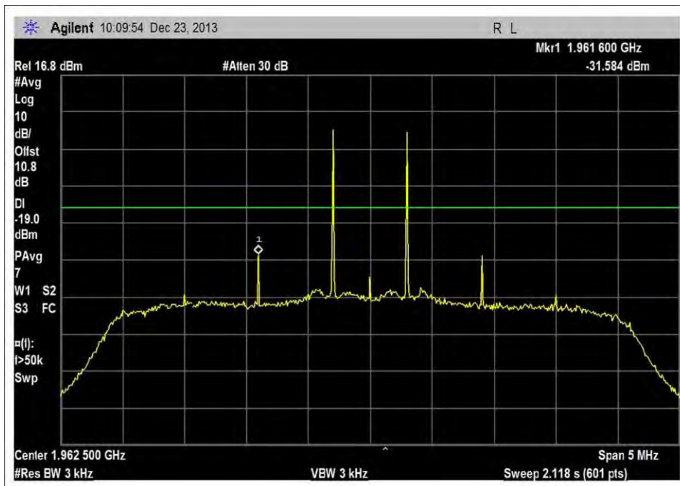
DL_1930-1995MHz_-75dBm
