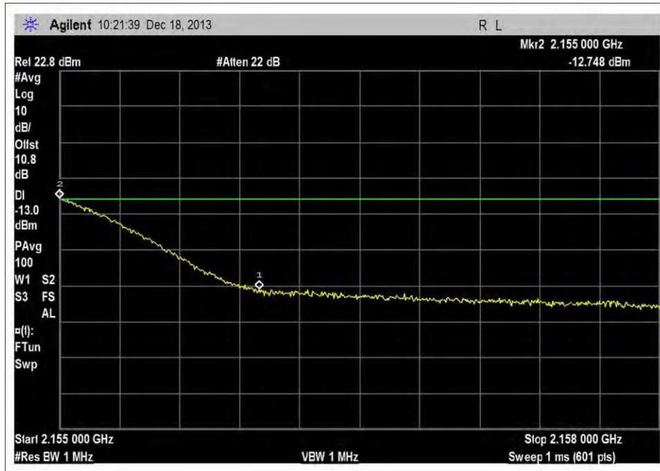
DL_2110-2155MHz_H_-90dBm
