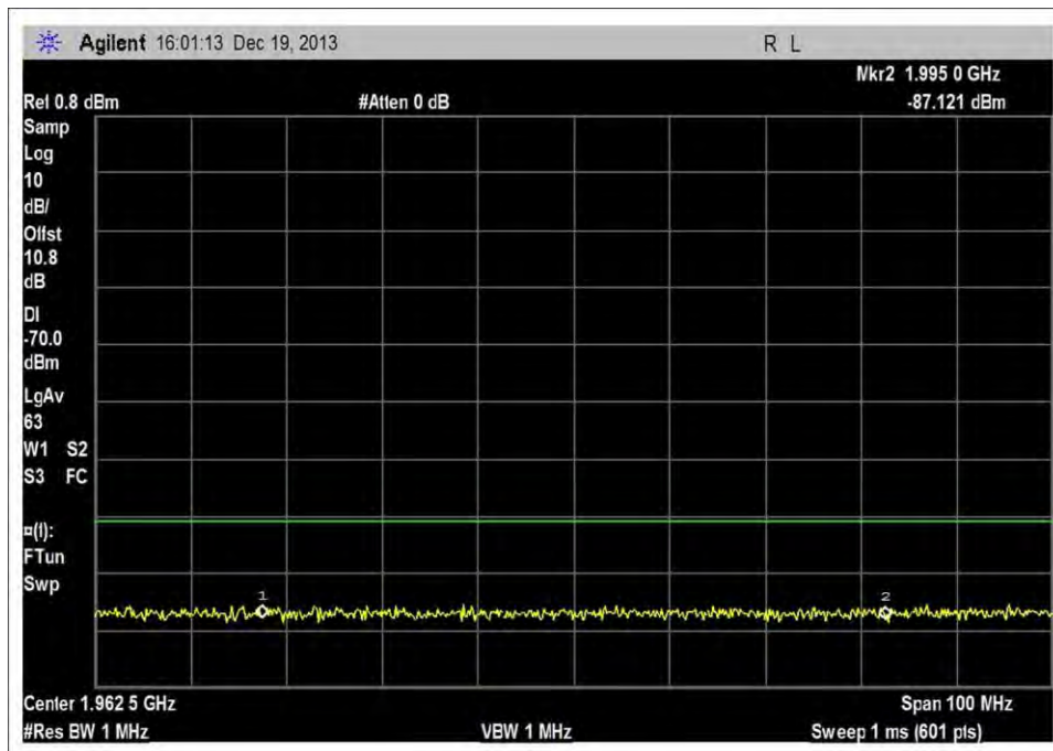
DL_1930-1995MHz_MNC260
