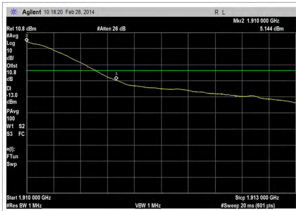
UL_1850-1915MHz_H_RFin_0dBm_rbw=1MHz
