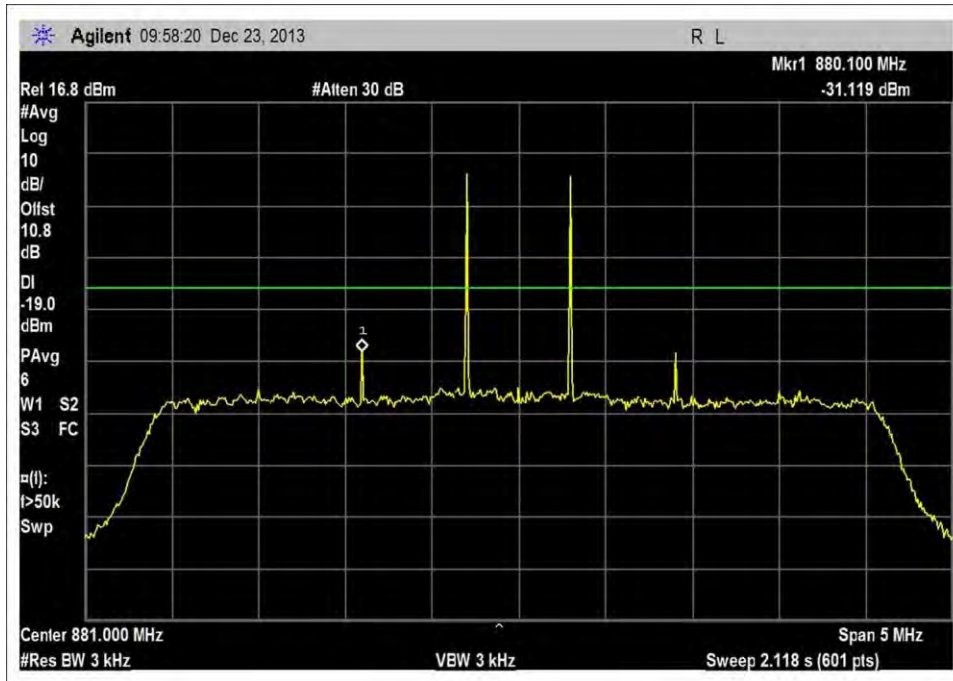
DL_869-894MHz_-85dBm
