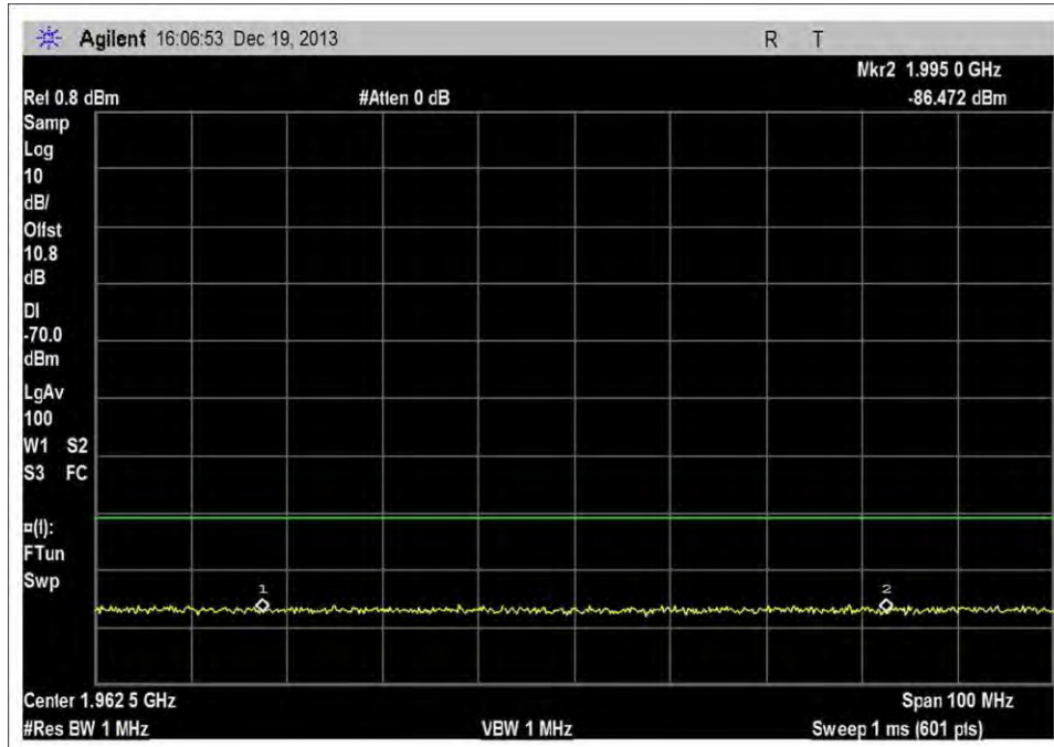
DL_1930-1995MHz_MNC005
