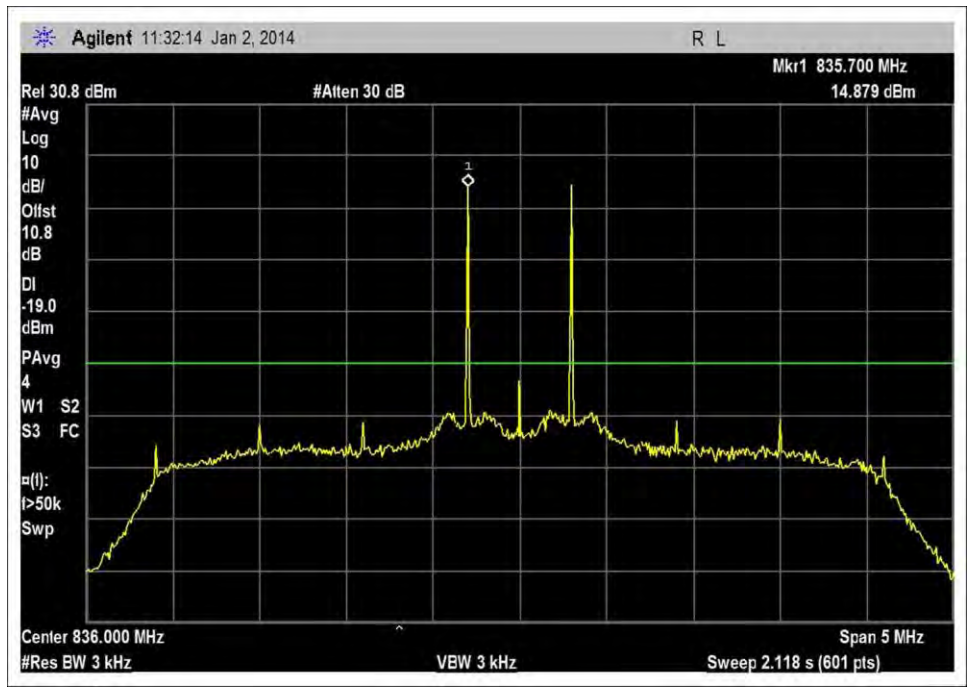
UL_824-849MHz_-50dBm
