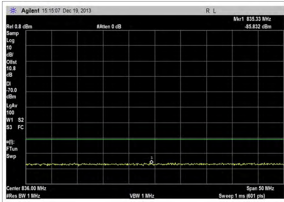
UL_824-849MHz_MNC260
