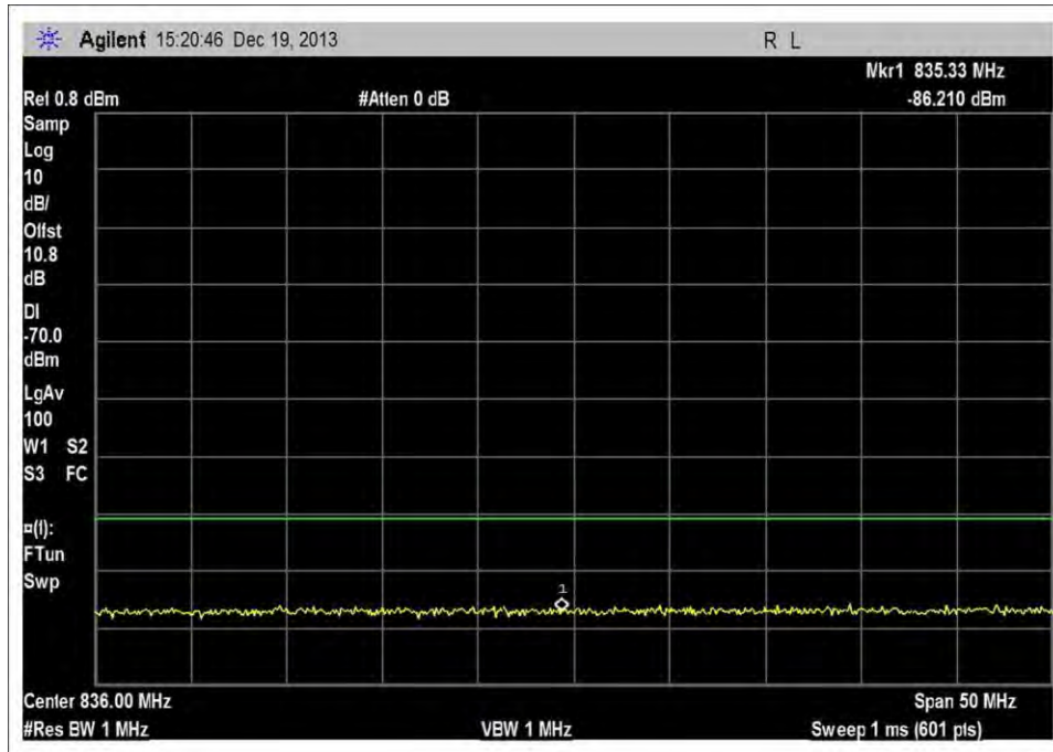
UL_824-849MHz_MNC005
