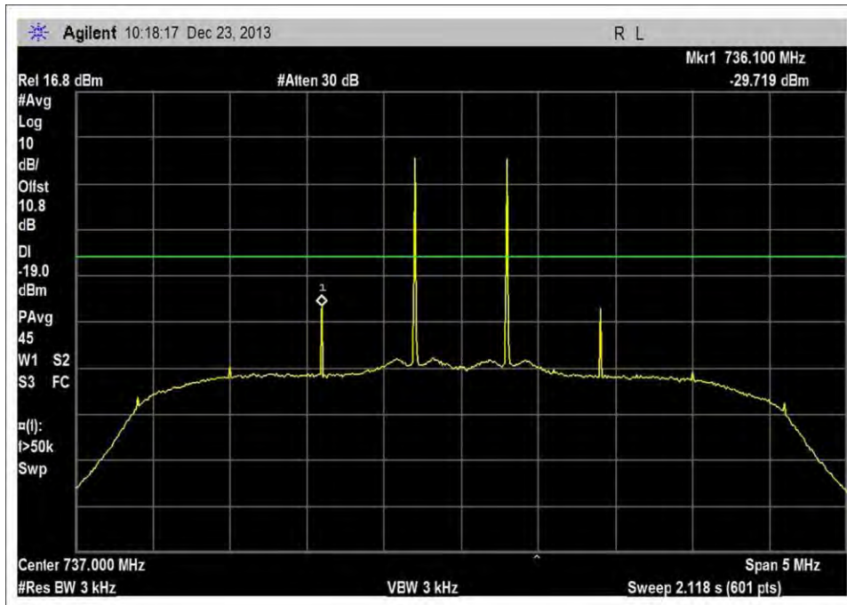
DL_716-746MHz_-75dBm
