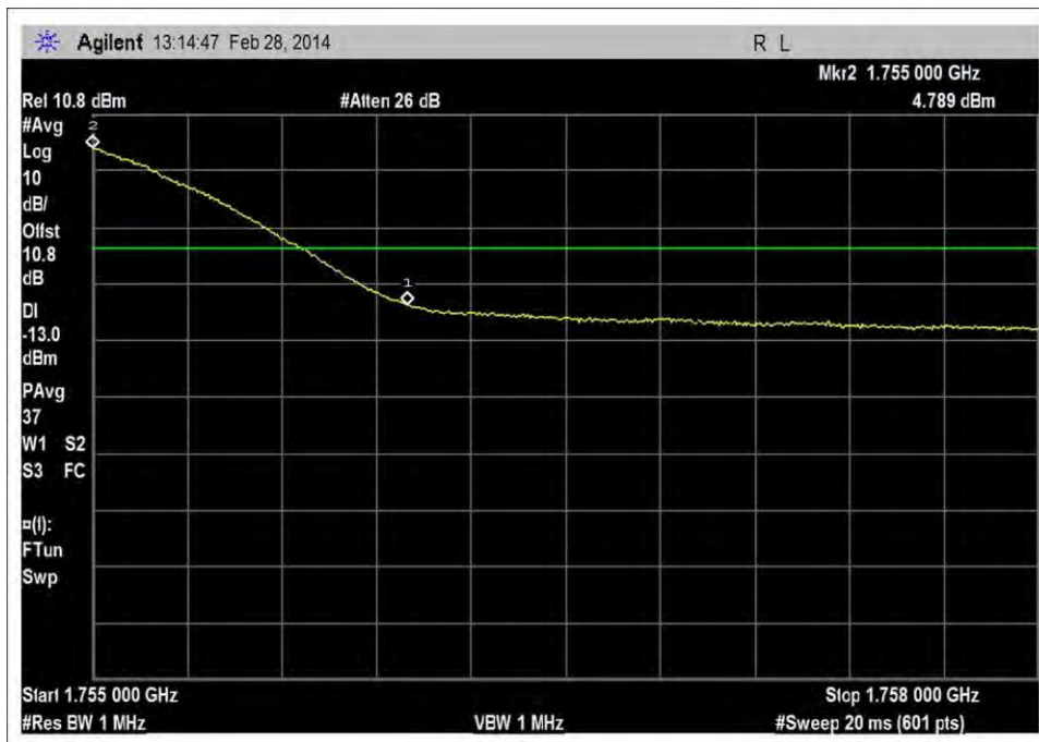
UL_1710-1755MHz_H_RFin_OdBm_rbw=1MHz
