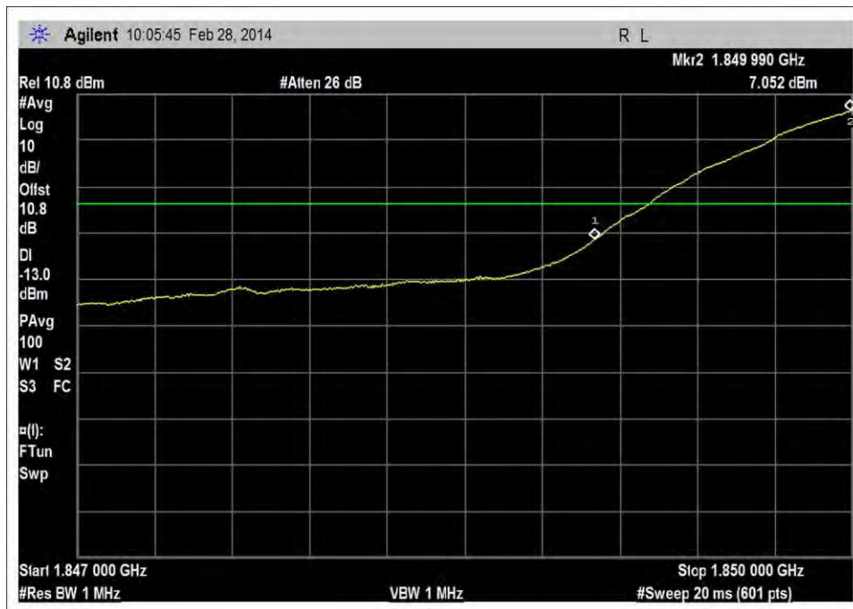
UL_1850-1915MHz_L_RFin -78dBm_rbw=1MHz
