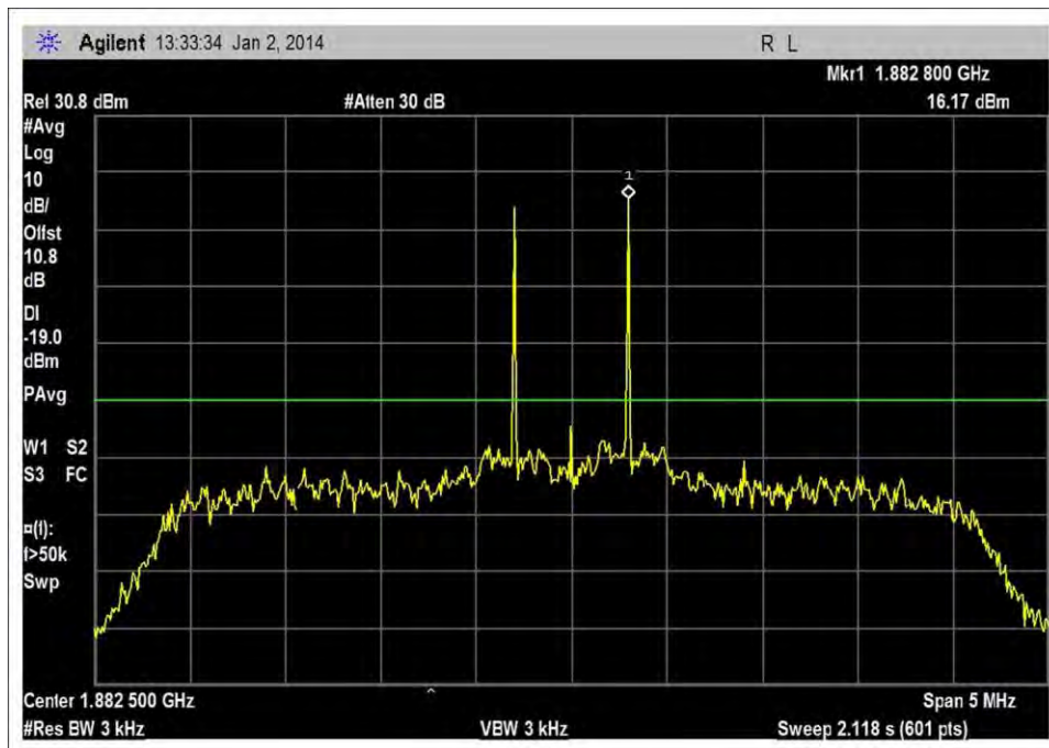
UL_1850-1915MHz_-50dBm
