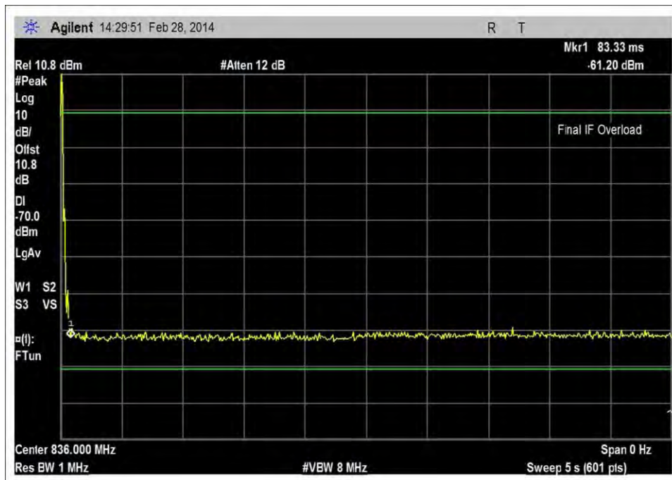
UL_824-849MHz_Single
