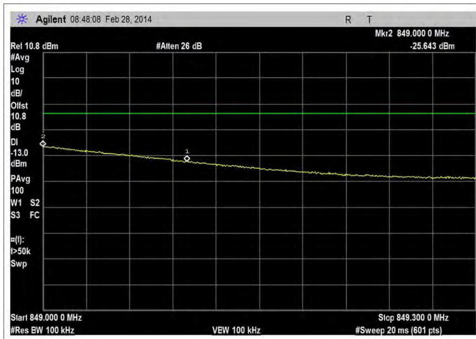
UL_824-849MHz_H_RFin 0dBm
