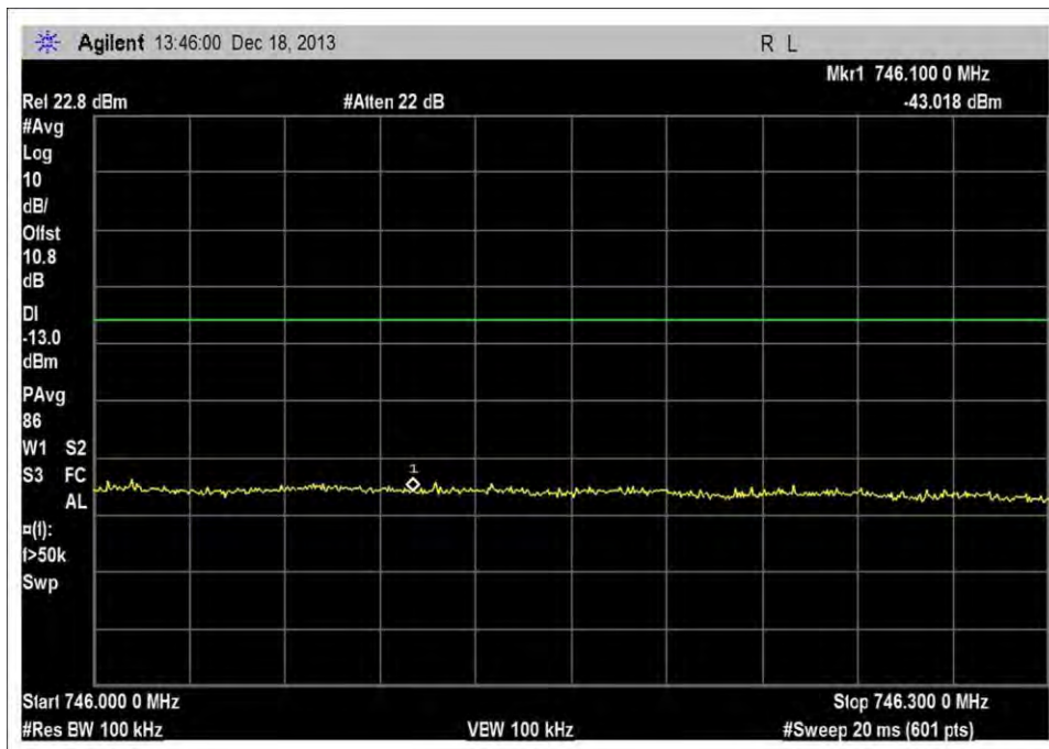
DL_716-746MHz_H_-90dBm
