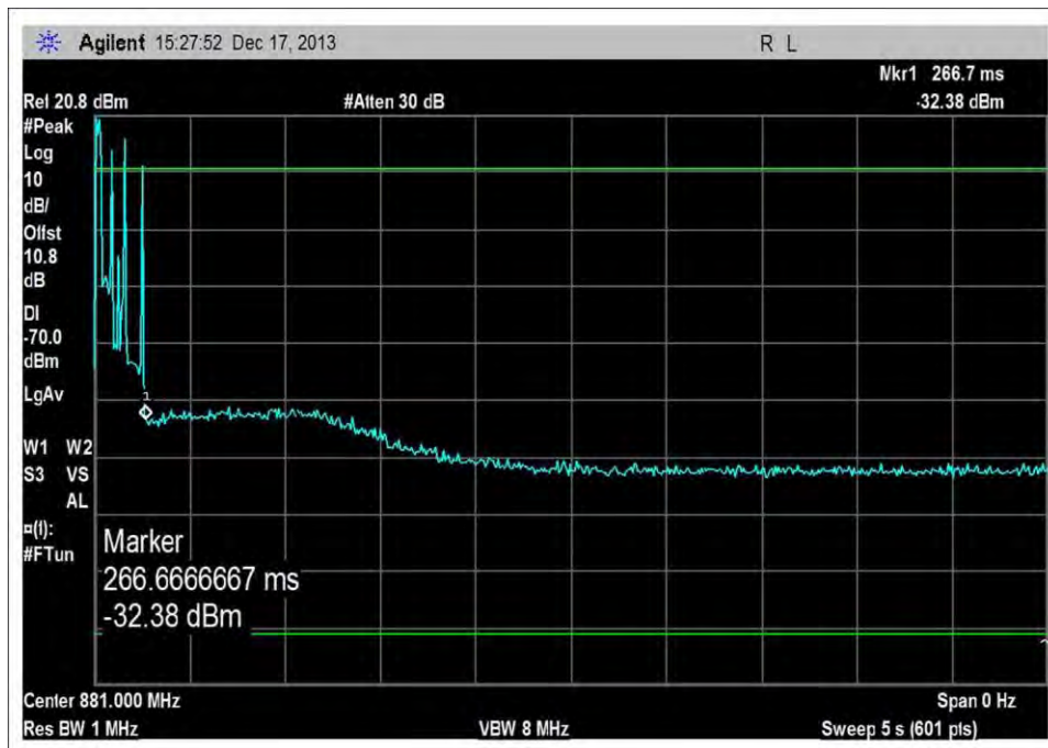
DL_869-894MHz_Single
