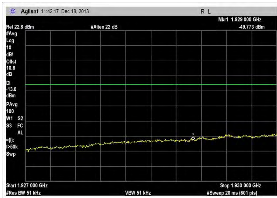
DL_1930-1995MHz_L_-90dBm_rbw50k
