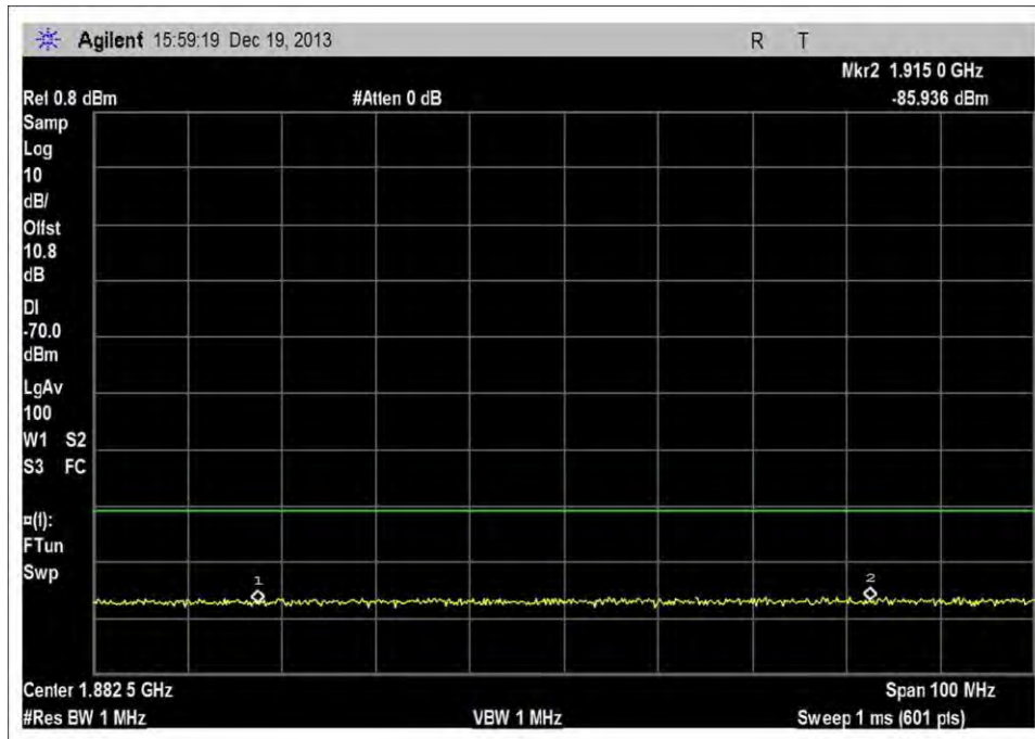
UL_1850-1915MHz_MNC260
