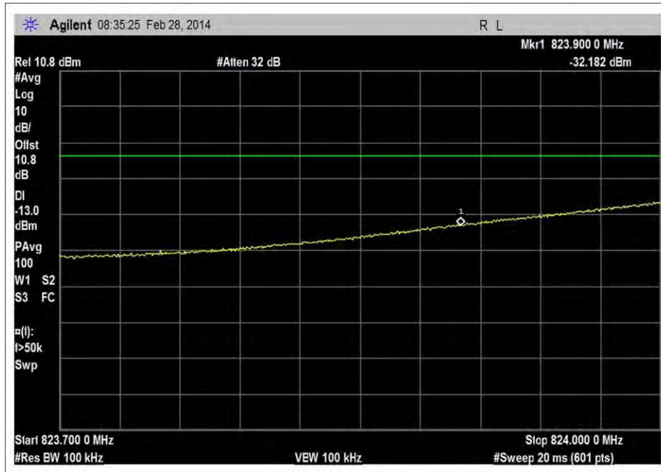
UL_824-849MHz_L_RFin -78dBm
