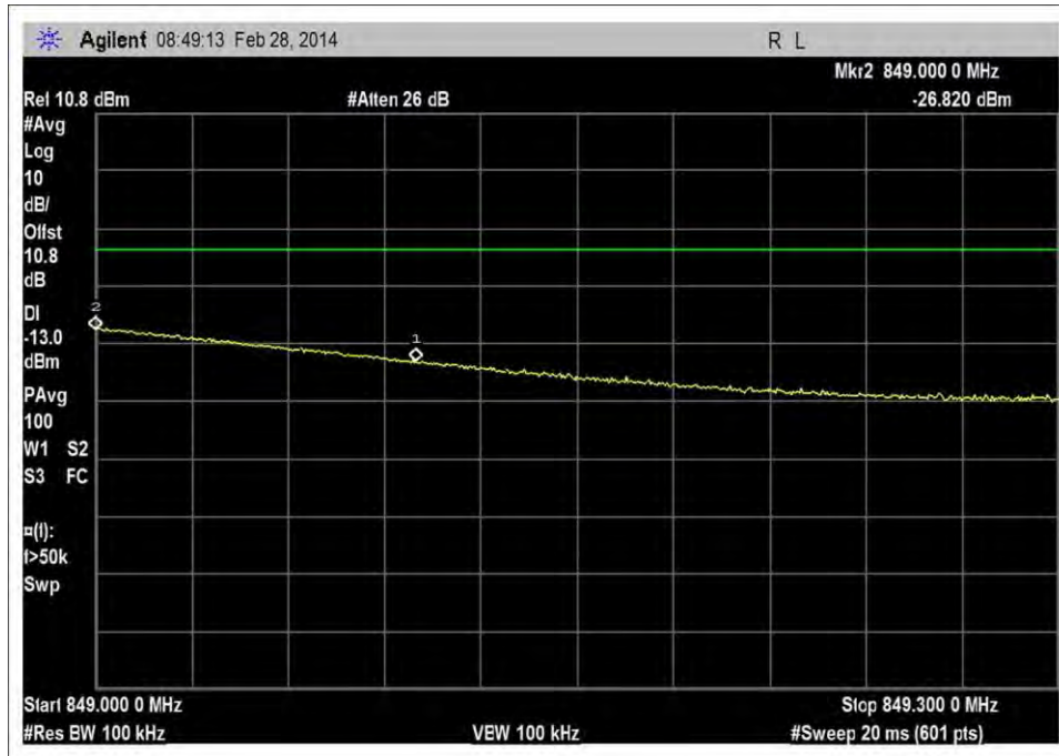
UL_824-849MHz_H_RFin -78dBm
