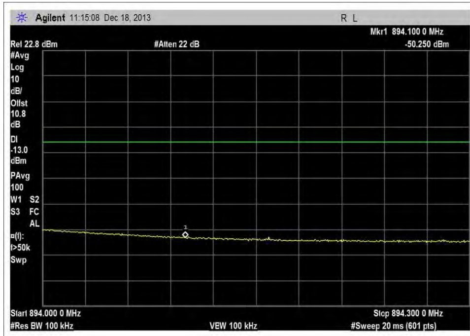
DL_869-894MHz_H_-20dBm
