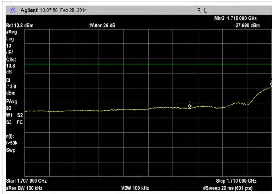
UL_1710-1755MHz_L_RFin_0dBm_rbw=100kHz
