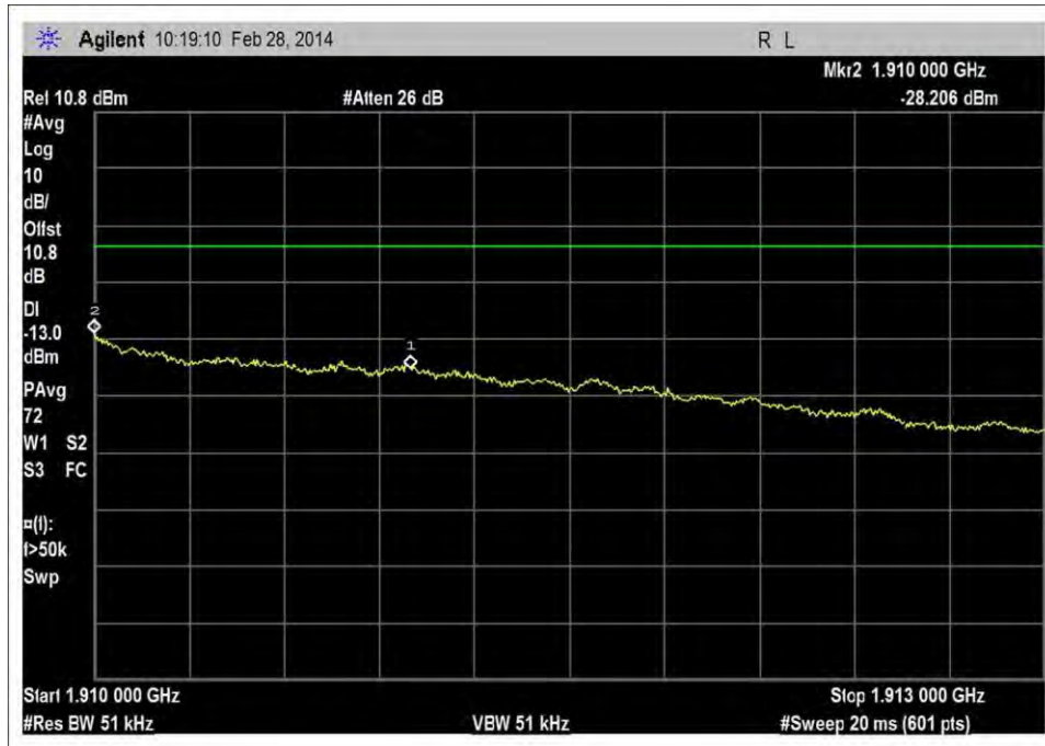
UL_1850-1915MHz_H_RFin_0dBm_rbw=50kHz
