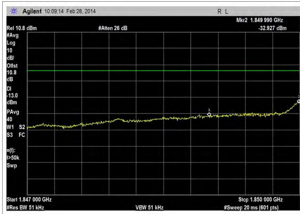
UL_1850-1915MHz_L_RFin OdBm_rbw=51kHz
