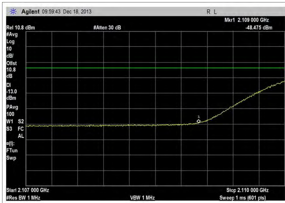
DL_2110-2155MHz_L_-90dBm
