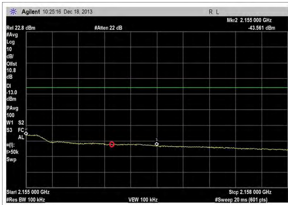
DL_2110-2155MHz_H_-90dBm_rbw100kHz
