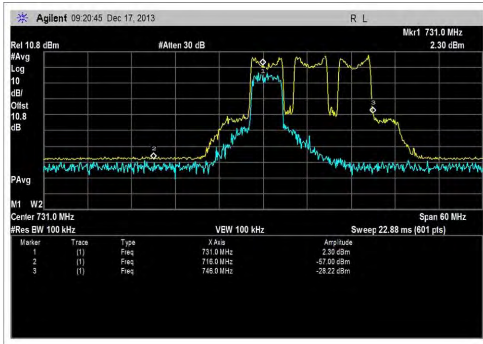
DL_716-746MHz
