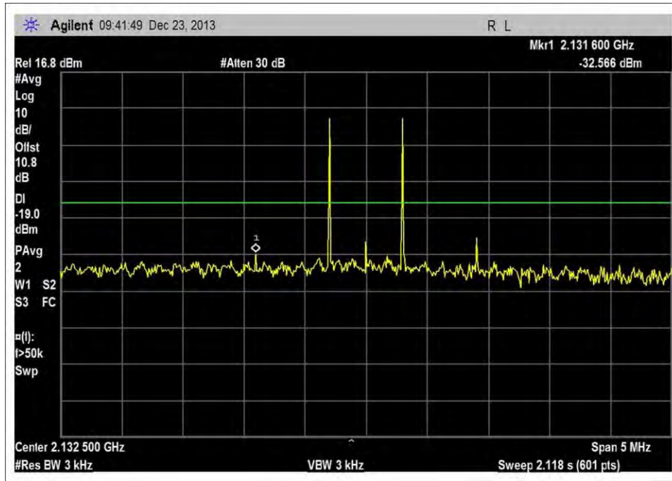
DL_2110-2155MHz_-85dBm
