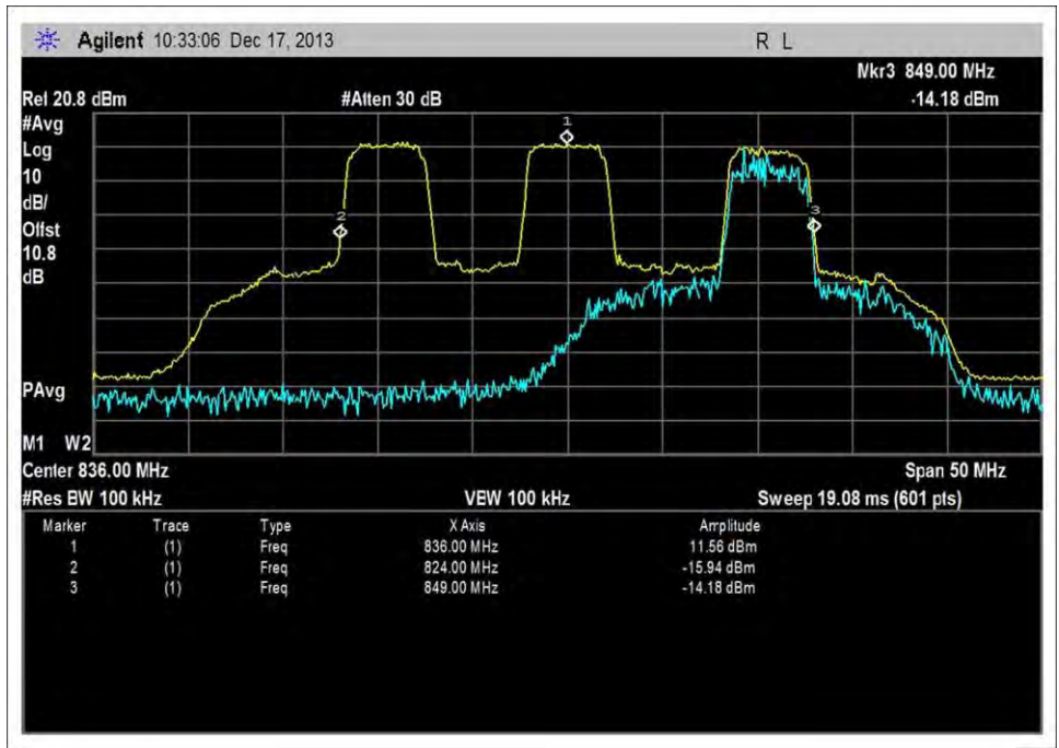
UL_824-849MHz
