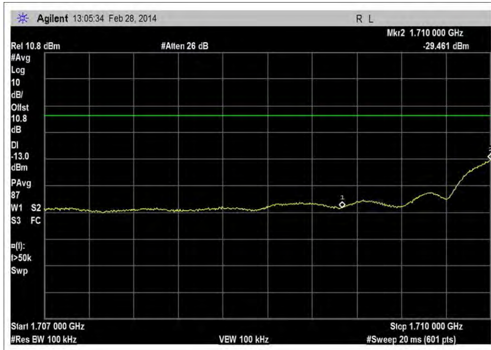
UL_1710-1755MHz_L_RFin -78dBm_rbw=100kHz
