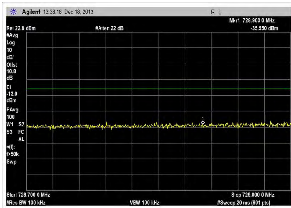
DL_716-746MHz_L_-90dBm
