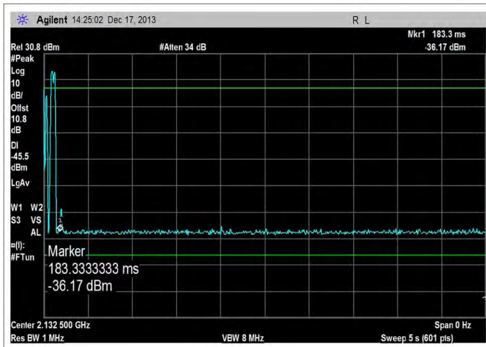
DL_2110-2155MHz_Single
