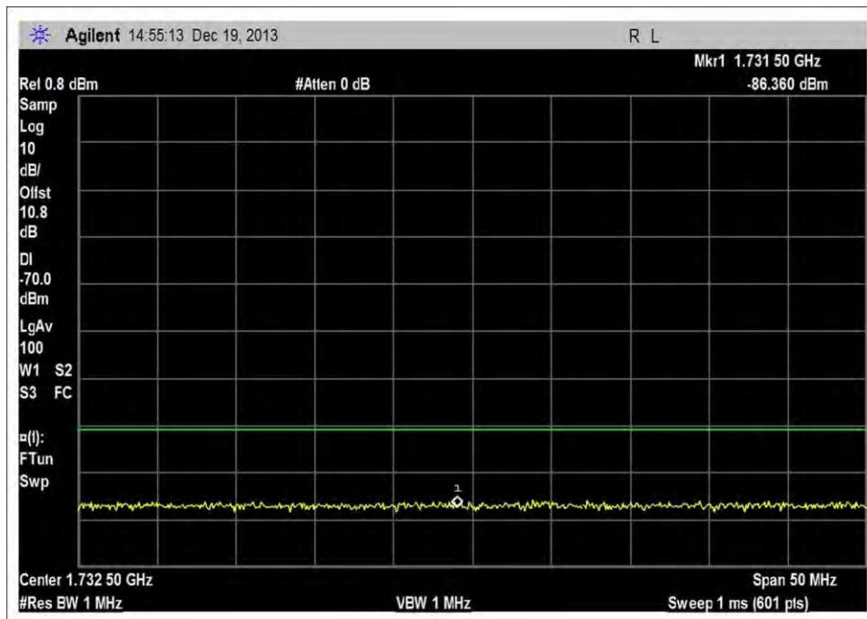
UL_1710-1755MHz_MNC005
