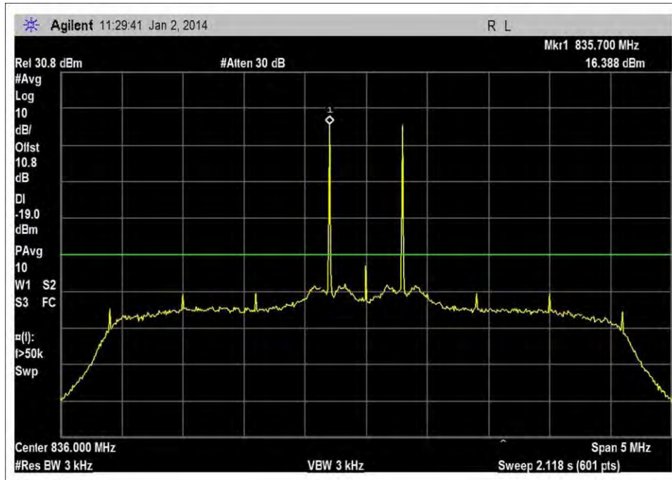
UL_824-849MHz_-60dBm
