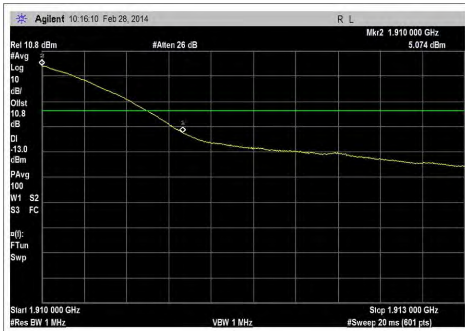
UL_1850-1915MHz_H_RFin -78dBm_rbw=1MHz
