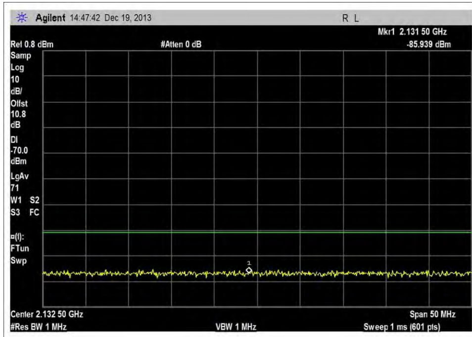
DL_2110-2155MHz_MNC260
