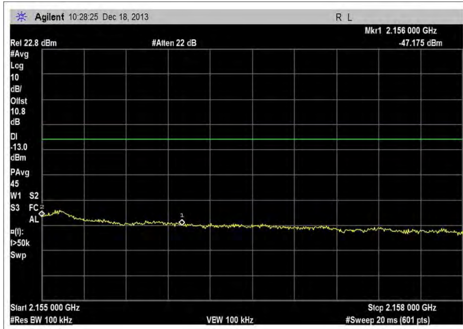
DL_2110-2155MHz_H_-20dBm_rbw100kHz
