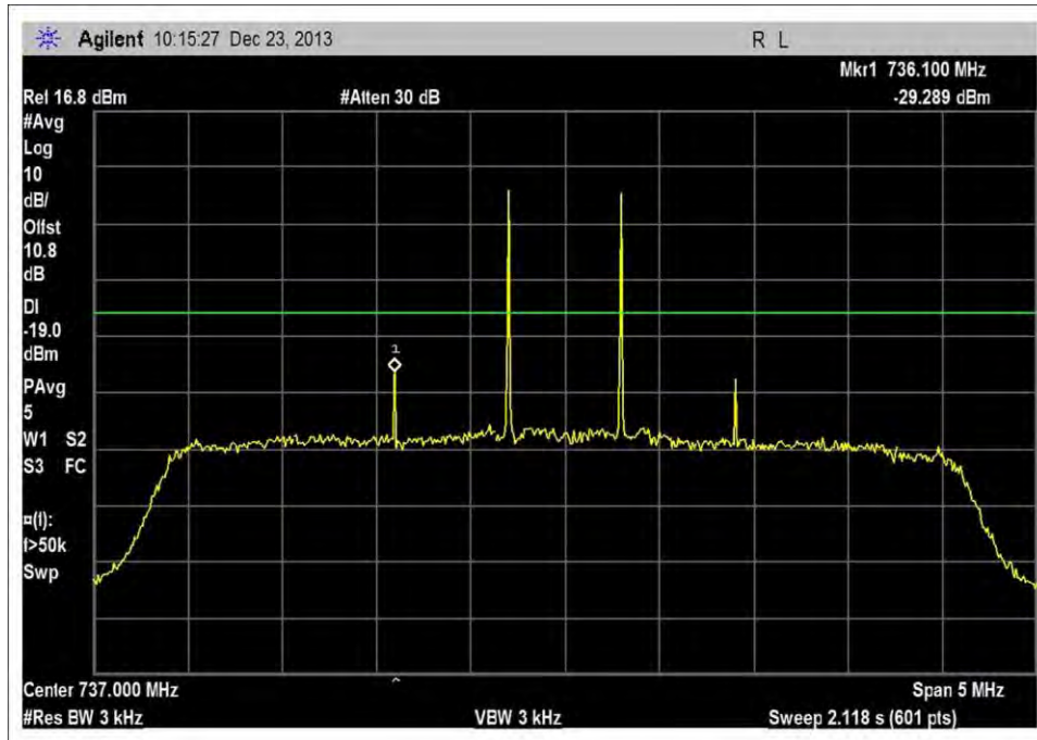
DL_716-746MHz_-85dBm
