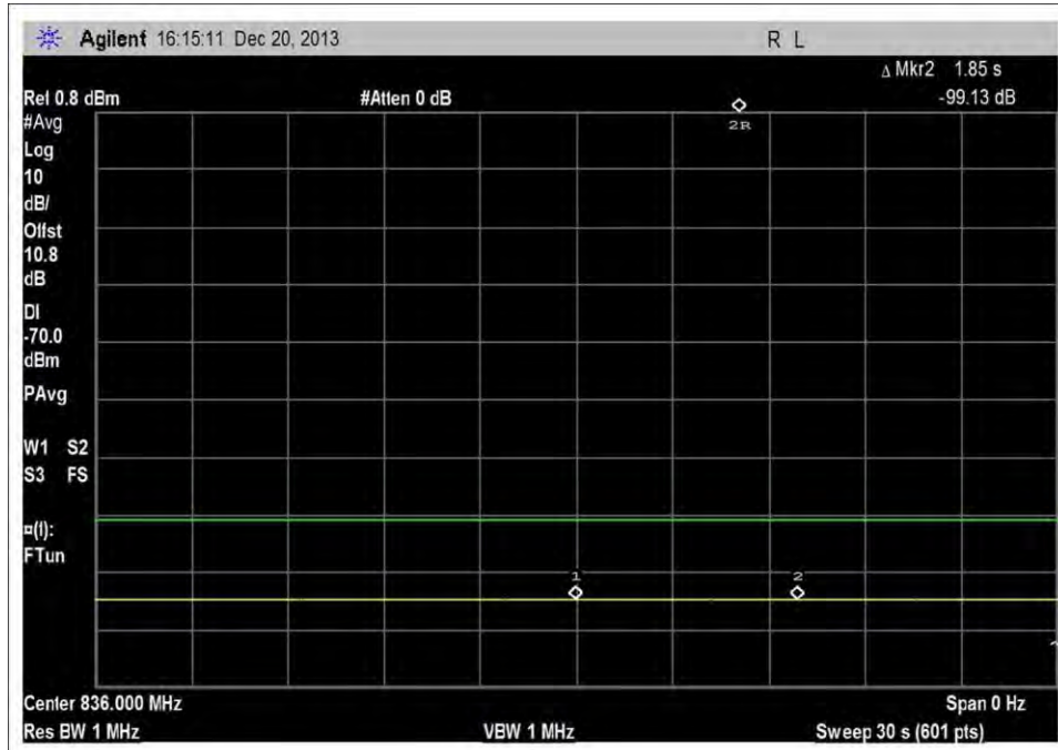
UL_824-849MHz_-70dBm
