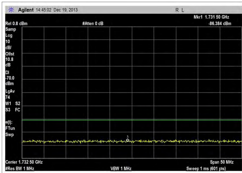
UL_1710-1755MHz_MNC260
