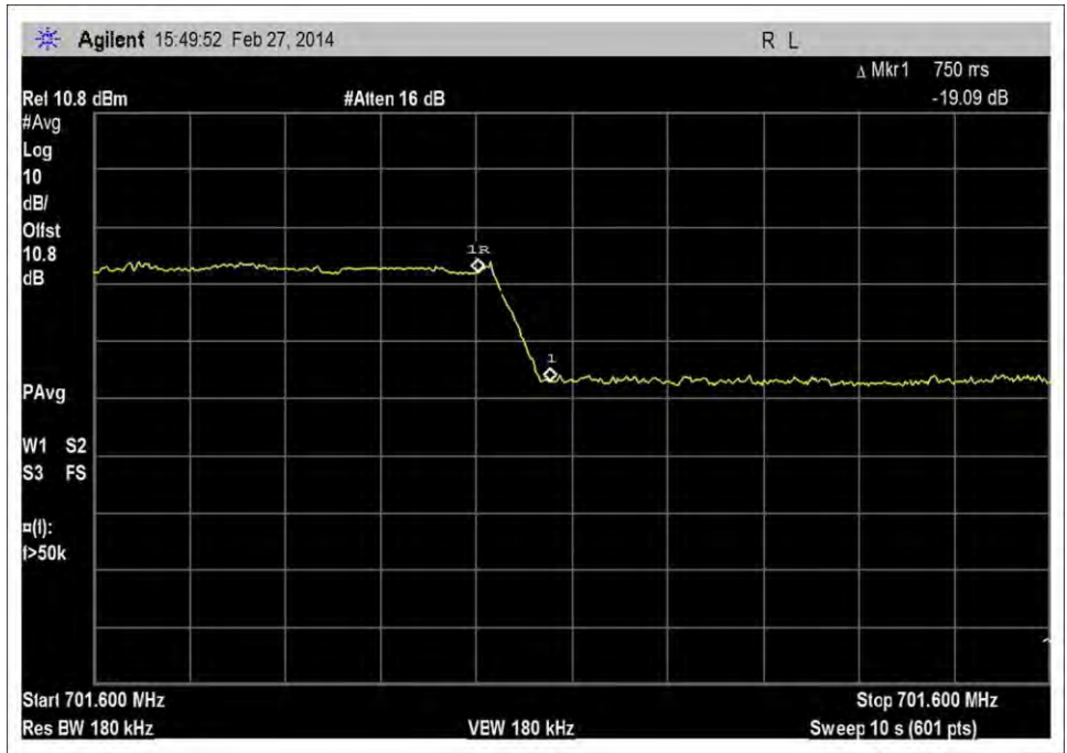
UL_698-716MHz
