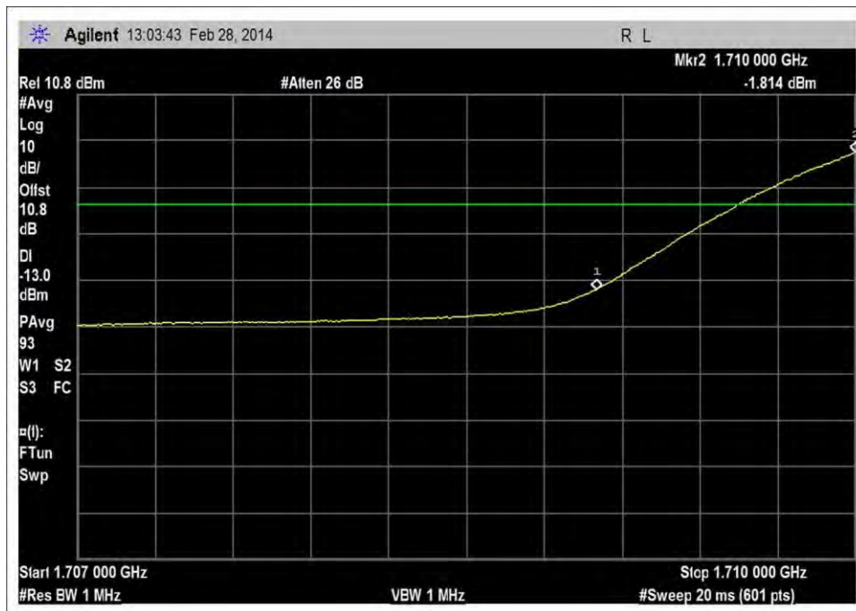
UL_1710-1755MHz_L_RFin -78dBm_rbw=1MHz
