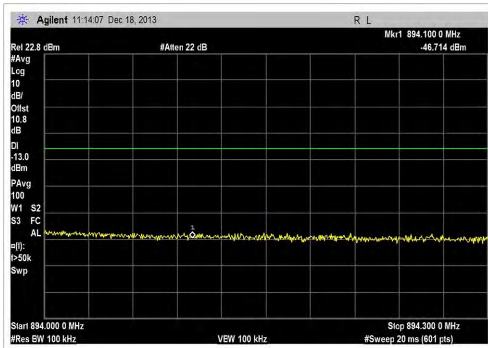
DL_869-894MHz_H_-90dBm
