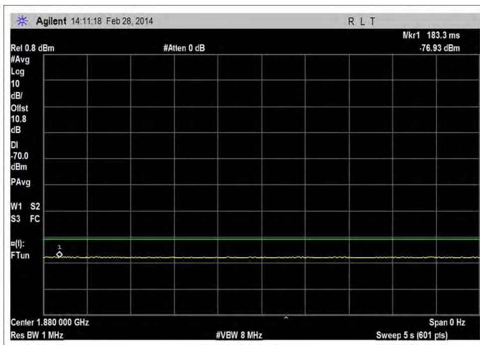
UL_1850-1915MHz_-70dBm
