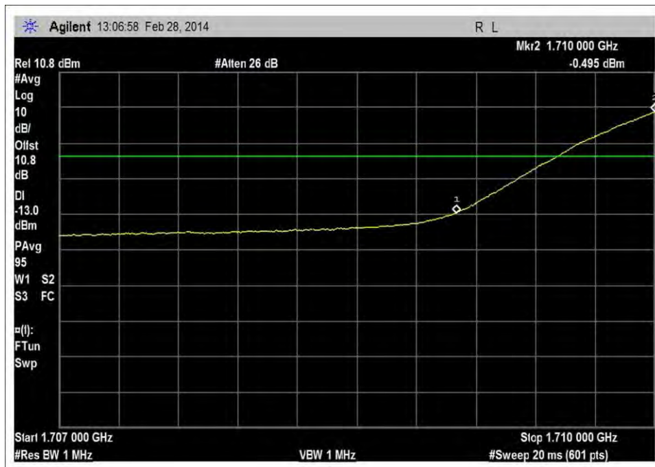
UL_1710-1755MHz_L_RFin_0dBm_rbw=1MHz
