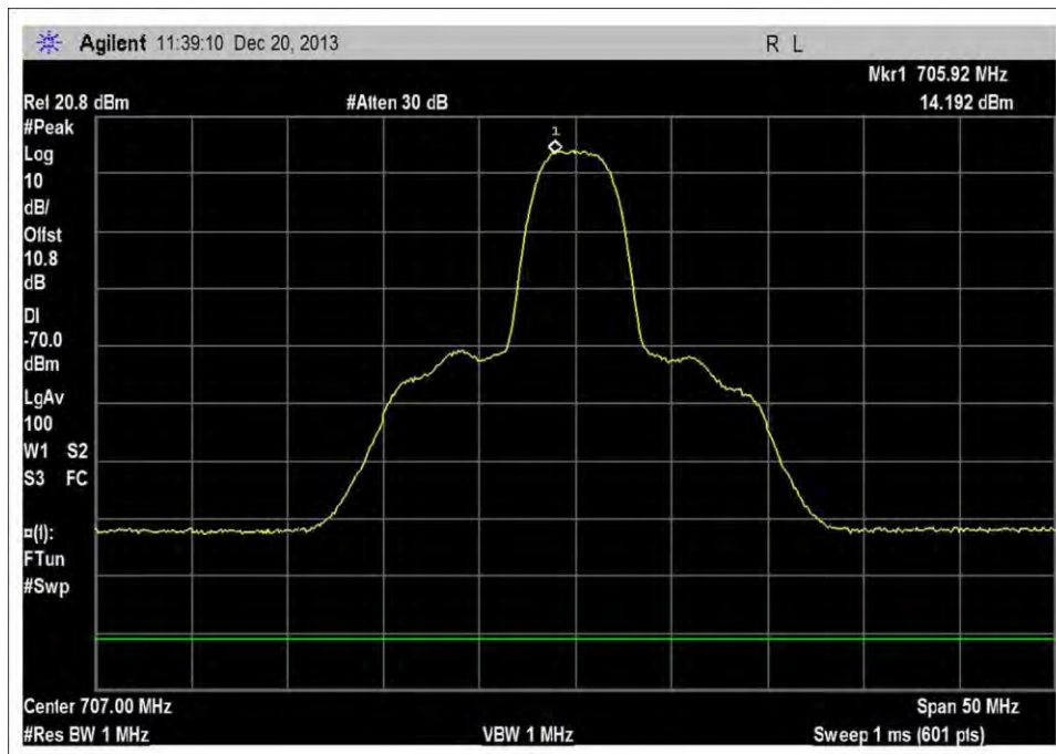
UL_698-716MHz_MNC410
