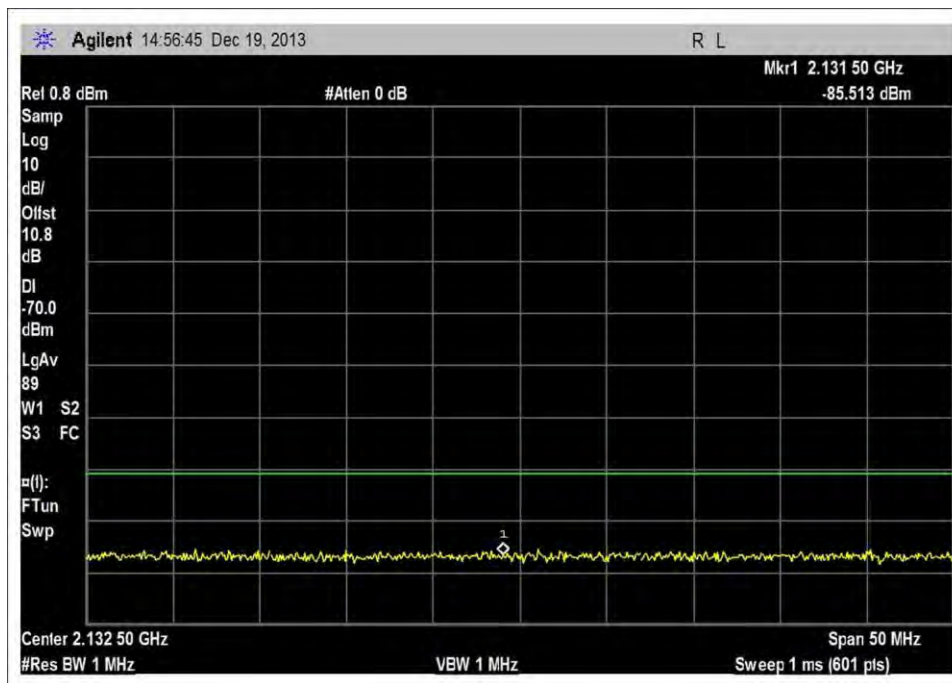
DL_2110-2155MHz_MNC005
