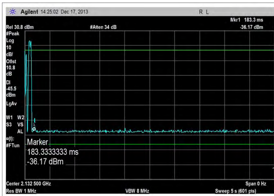
DL_2110-2155MHz_Single
