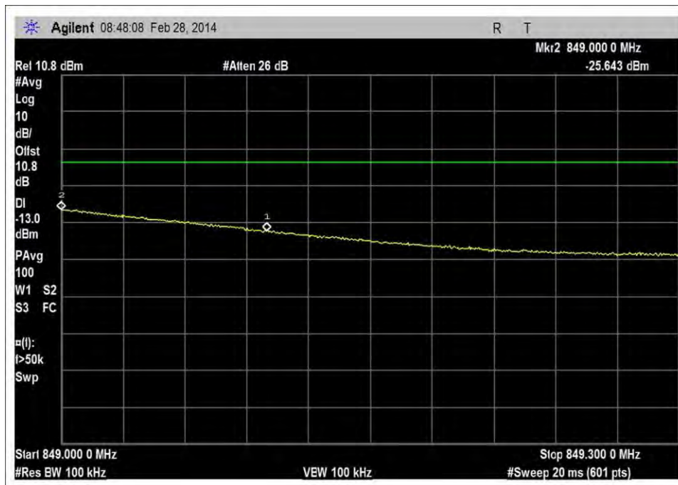
UL_824-849MHz_H_RFin 0dBm
