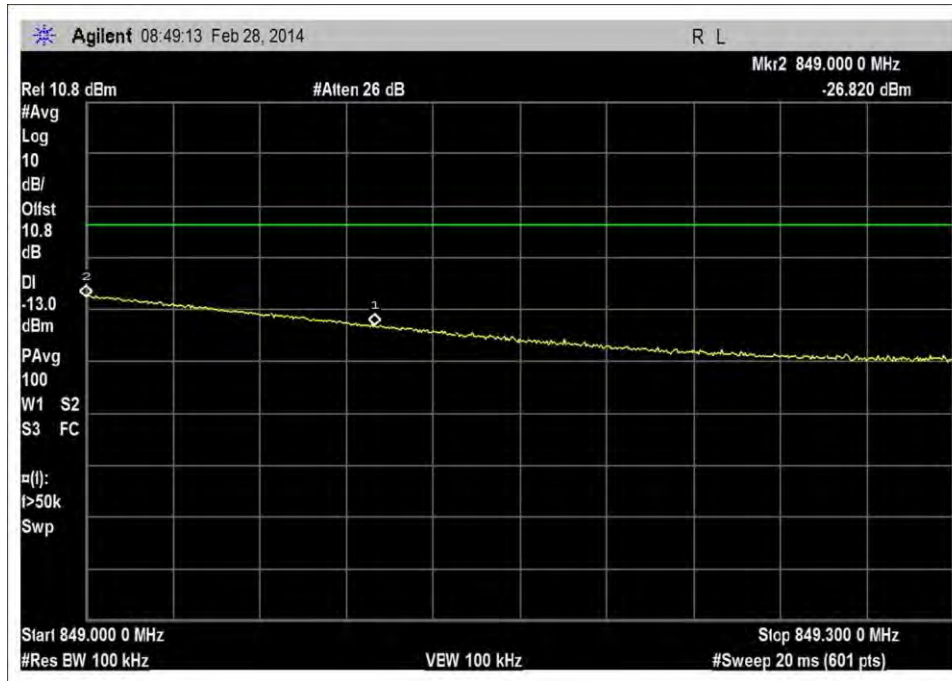
UL_824-849MHz_H_RFin -78dBm
