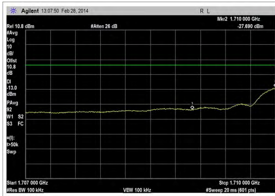
UL_1710-1755MHz_L_RFin_0dBm_rbw=100kHz
