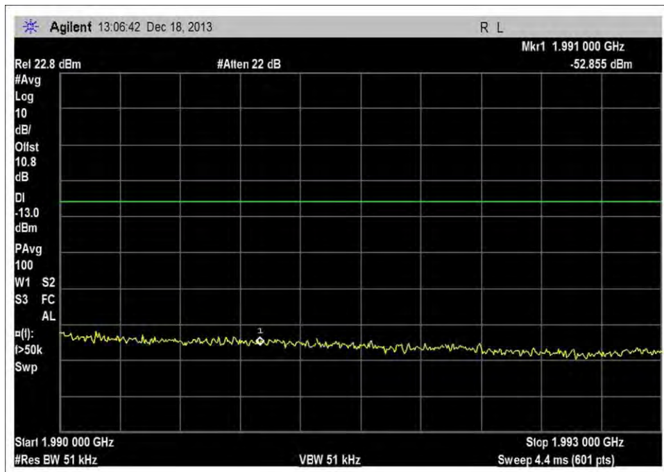
DL_1930-1995MHz_H_-20dBm_rbw51k
