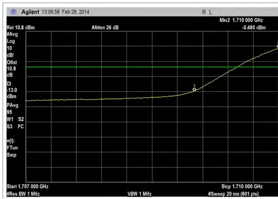
UL_1710-1755MHz_L_RFin_0dBm_rbw=1MHz
