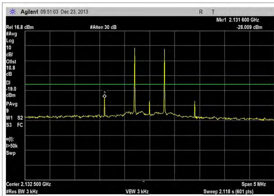
DL_2110-2155MHz_-75dBm
