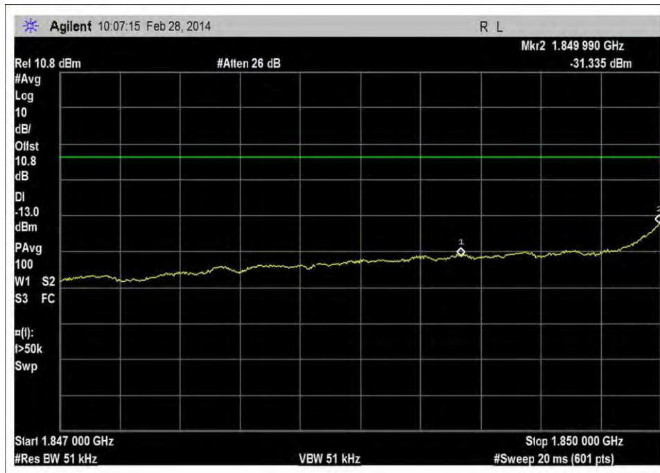
UL_1850-1915MHz_L_RFin -78dBm_rbw=51kHz
