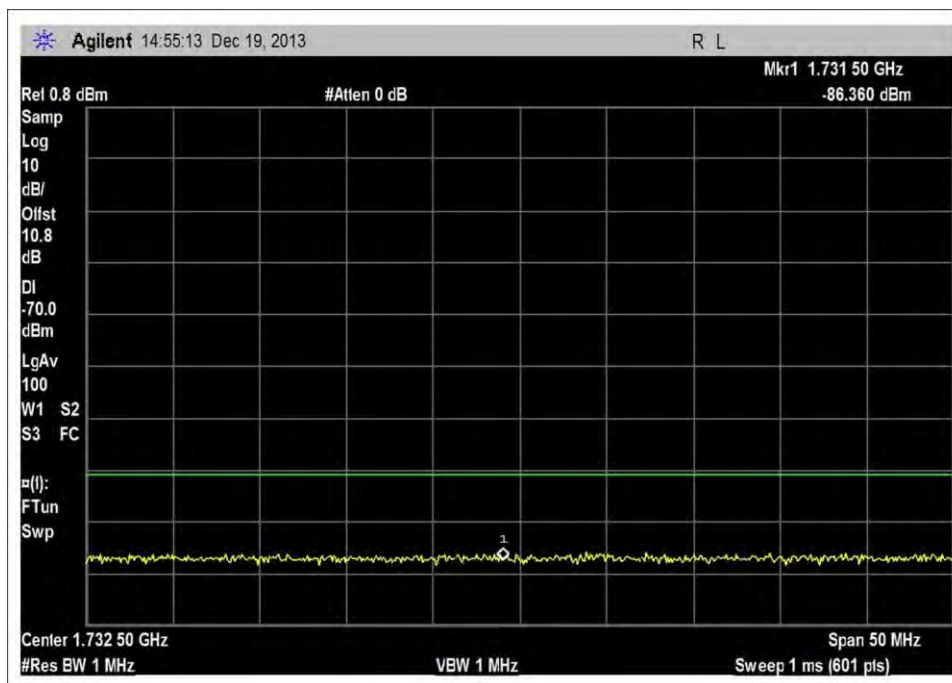
UL_1710-1755MHz_MNC005
