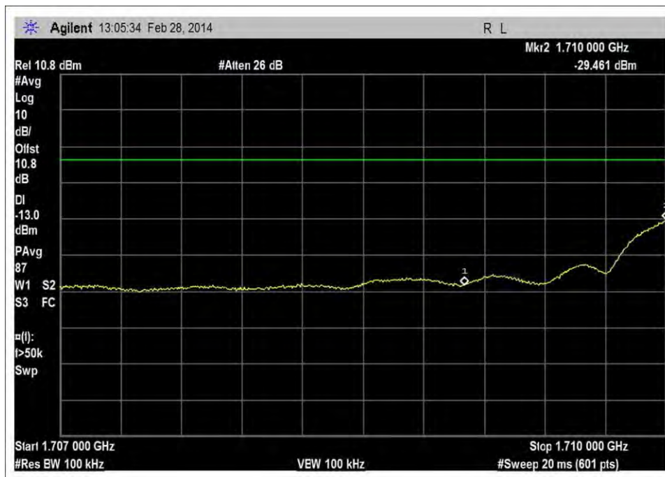
UL_1710-1755MHz_L_RFin -78dBm_rbw=100kHz
