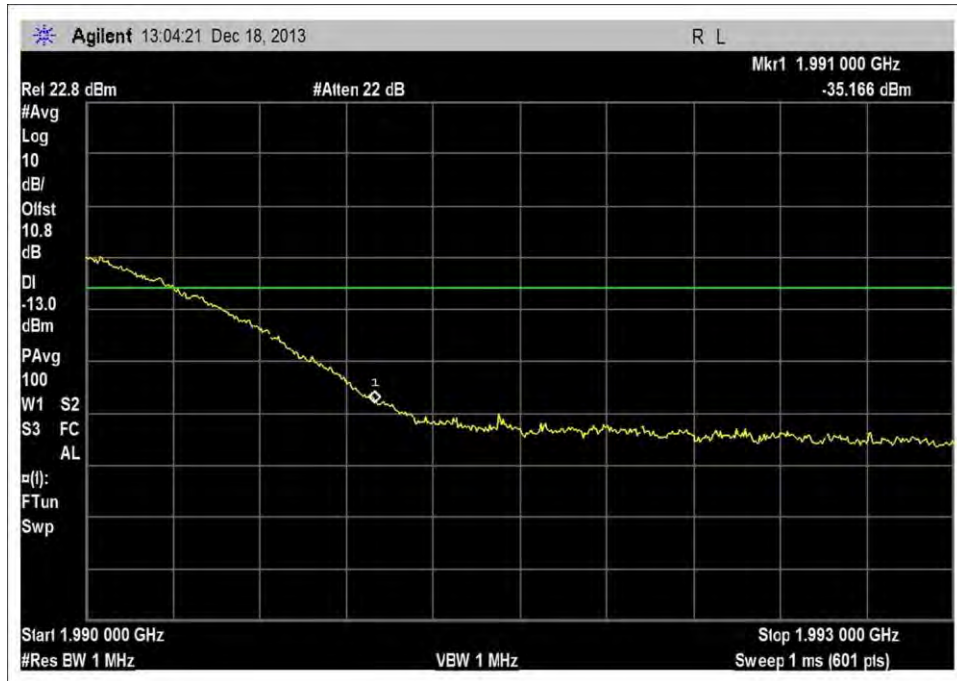
DL_1930-1995MHz_H_-20dBm
