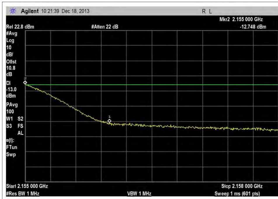
DL_2110-2155MHz_H_-90dBm
