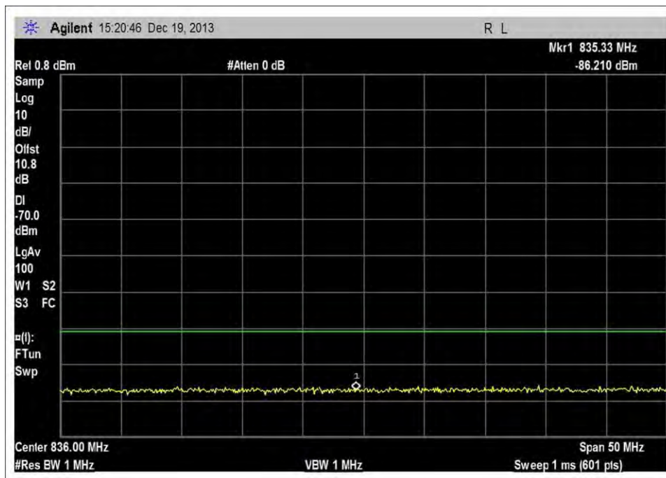
UL_824-849MHz_MNC005
