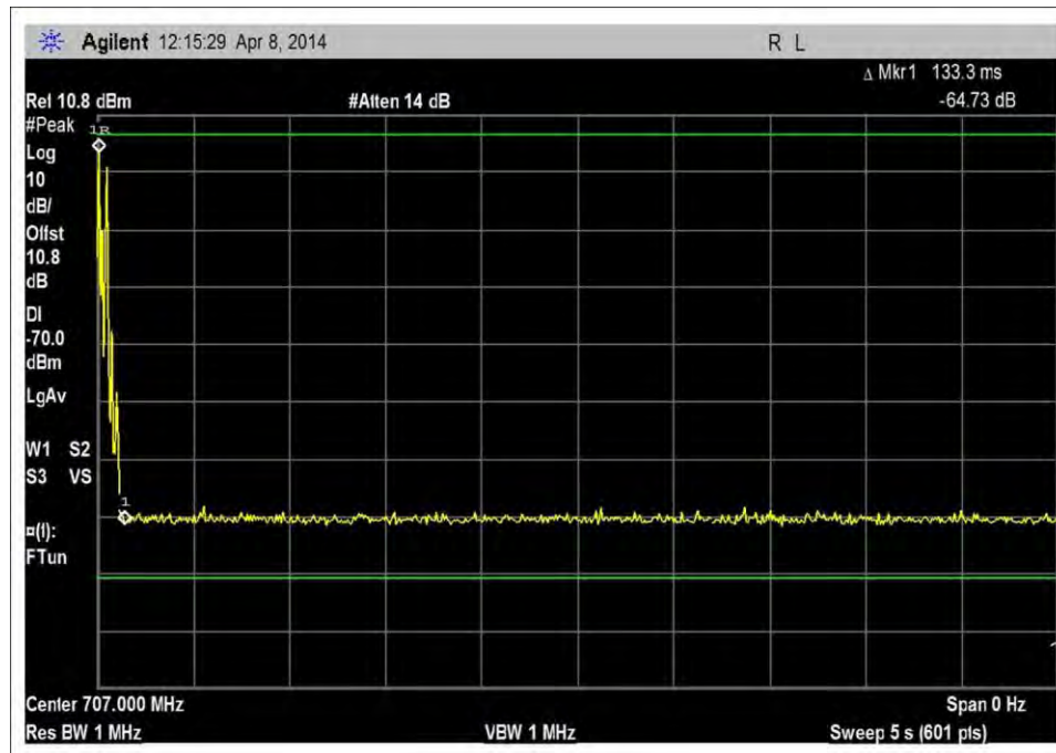
UL_698-716MHz_Single
