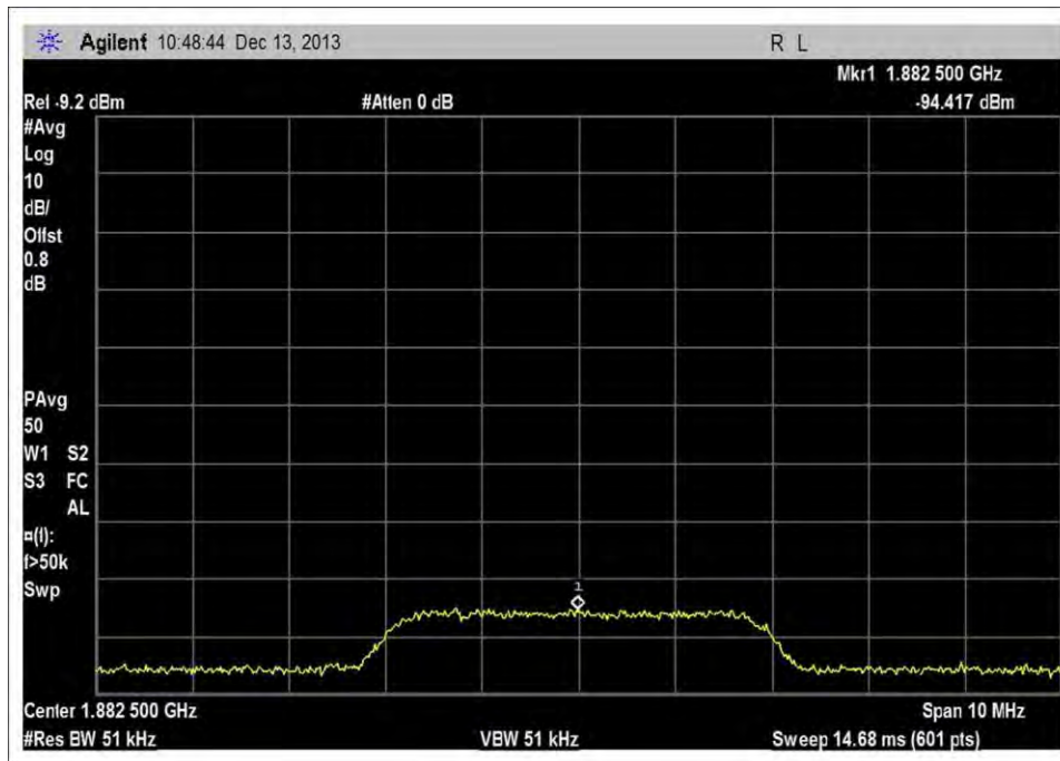
UL_1850-1915MHz_Input
