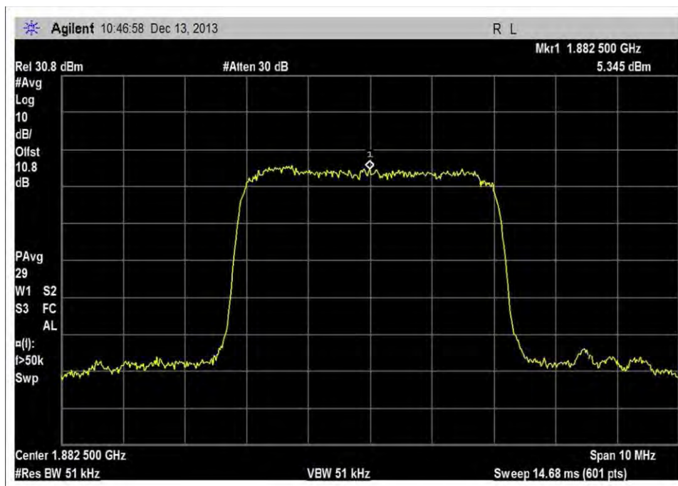
UL_1850-1915MHz_Output
