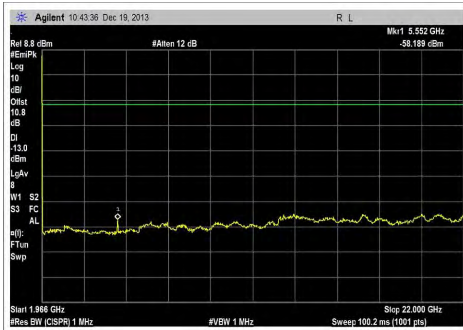
DL_1930-1995MHz_M_4.1AWGN_2
