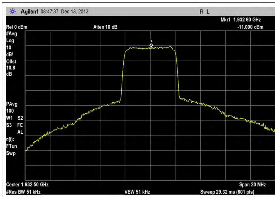
DL_1930-1995MHz_Output
