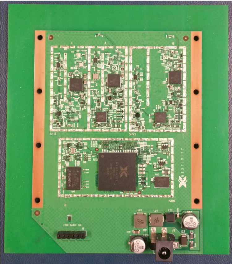
PCB Side_2_no shield - NU
