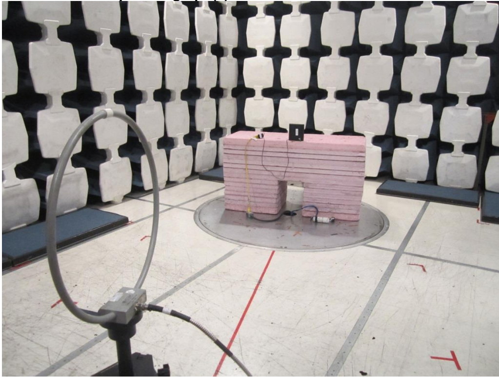
9kHz-1MHz
