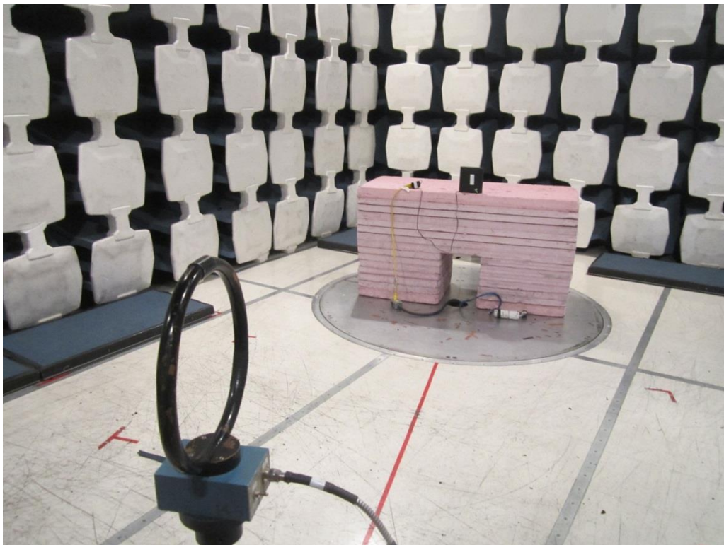
1-30MHz
