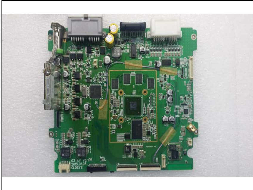
AV board (Top)
