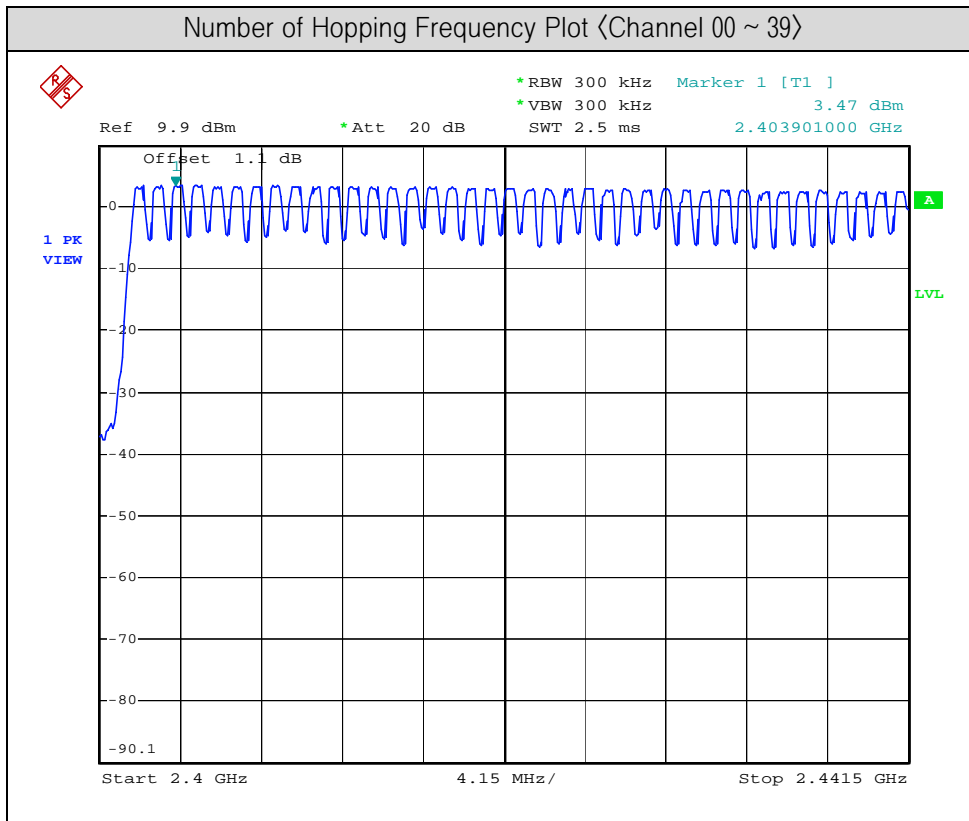
<2 400 MHz ~ 2 441.5 MHz>
