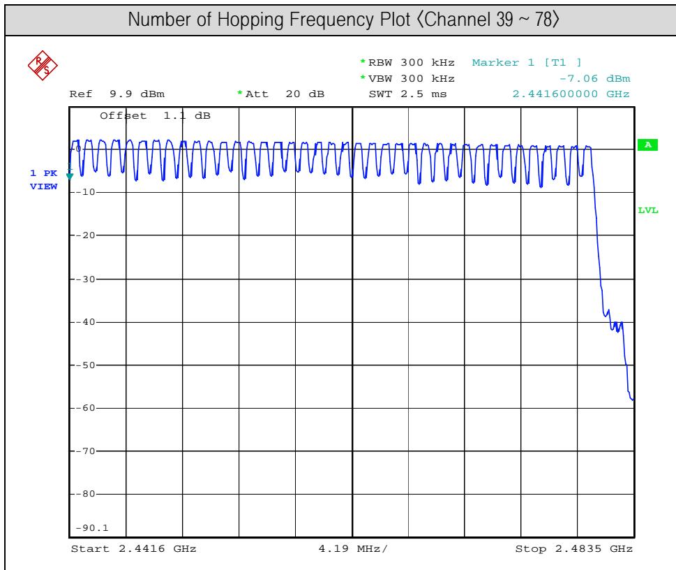
<2 441.5 MHz ~ 2 483.5 MHz>
