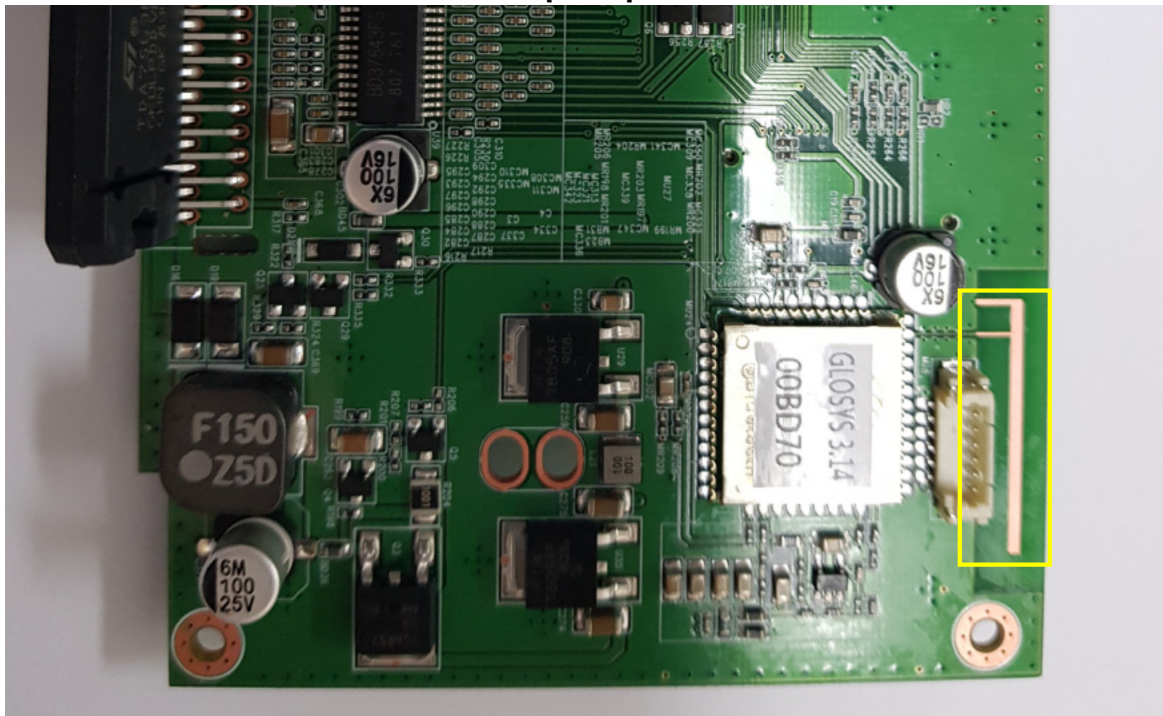
[Antenna]
