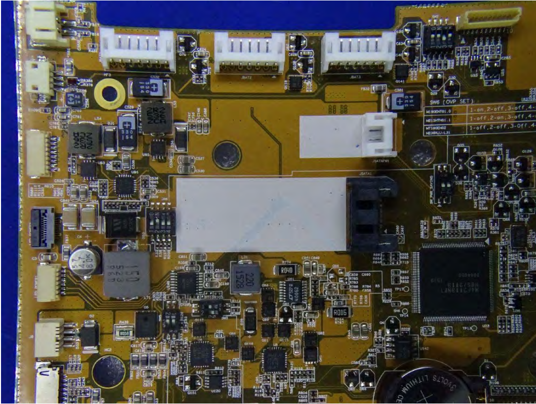
(180) EUT Photo
