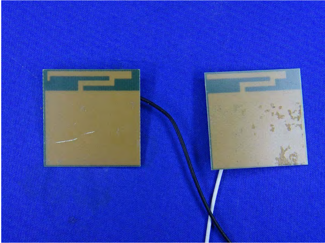
(214) EUT Photo
