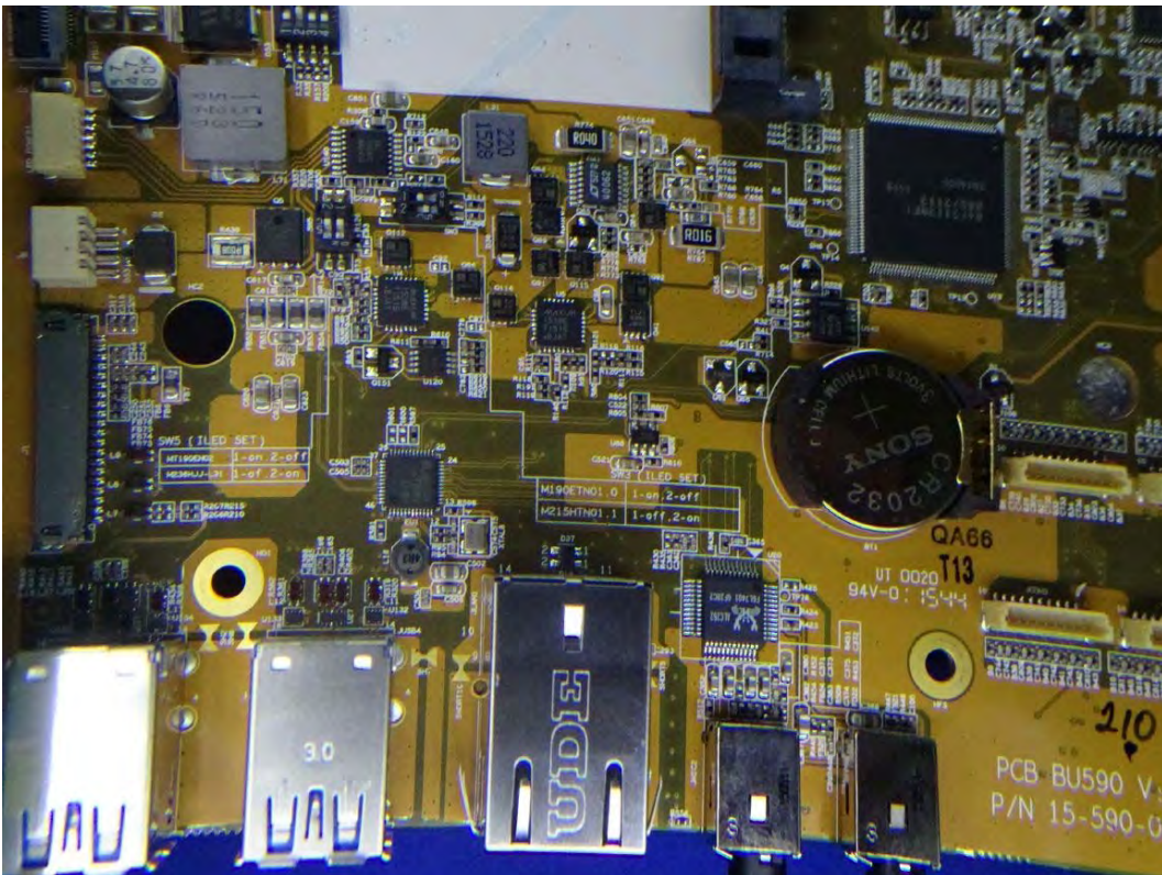
(181) EUT Photo
