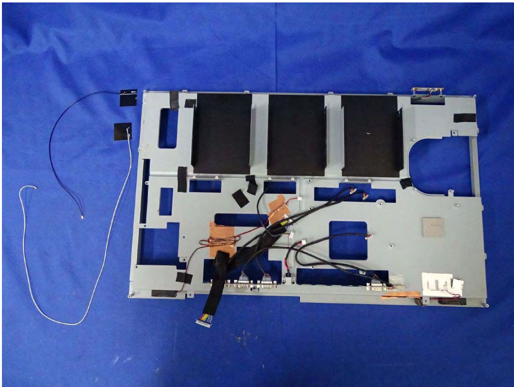
(211) EUT Photo
