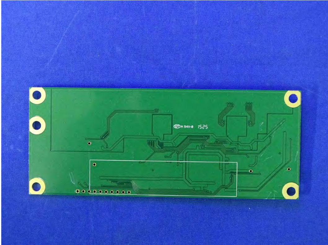
(200) EUT Photo
