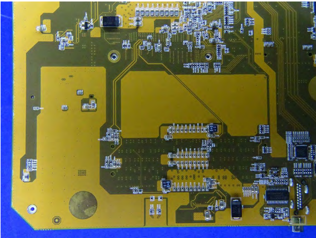
(187) EUT Photo
