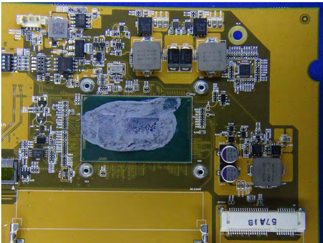
(183) EUT Photo
