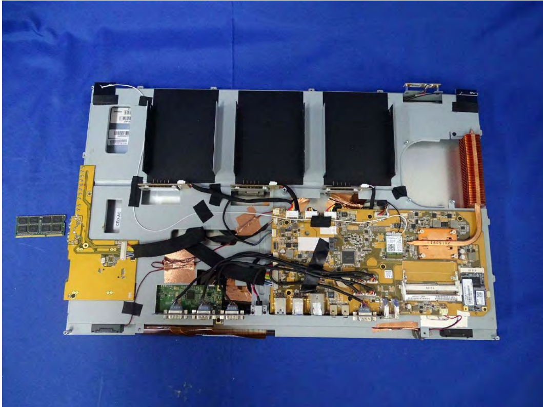
(168) EUT Photo
