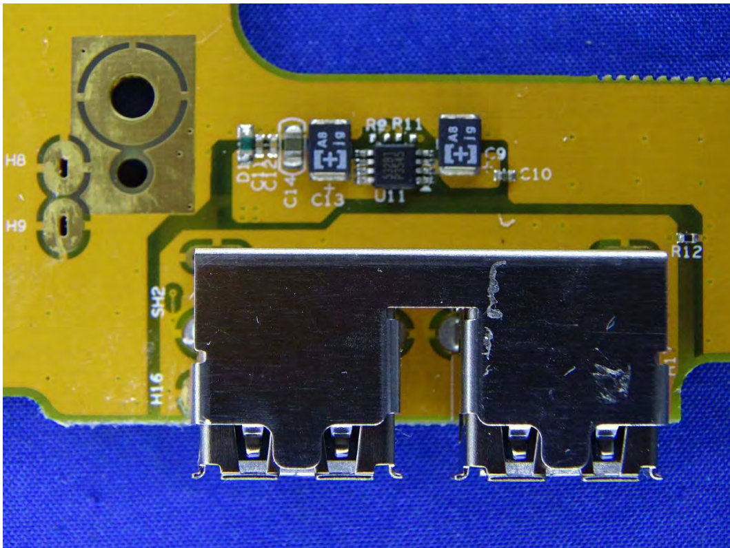
(167) EUT Photo
