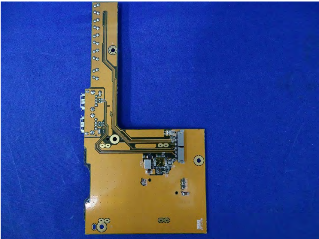
(163) EUT Photo
