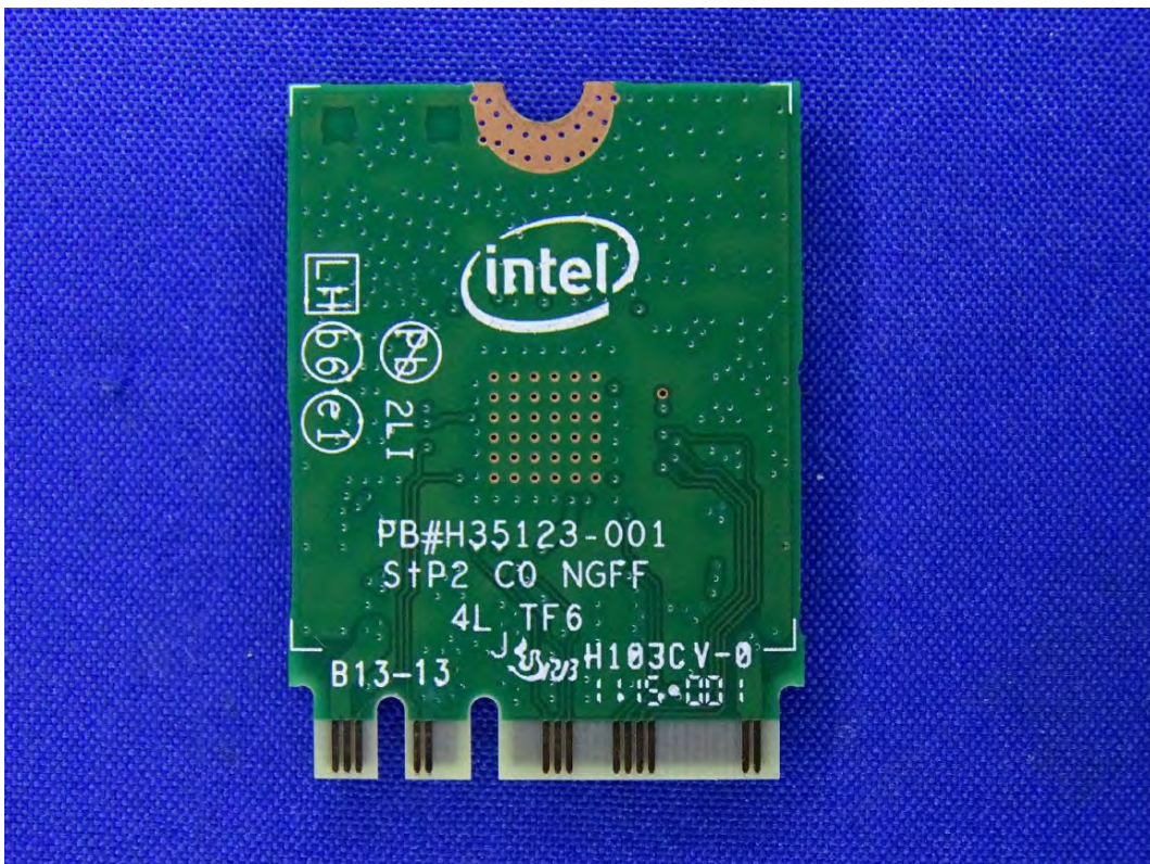
(177) EUT Photo
