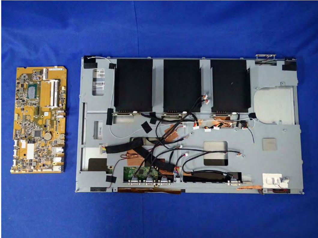
(178) EUT Photo
