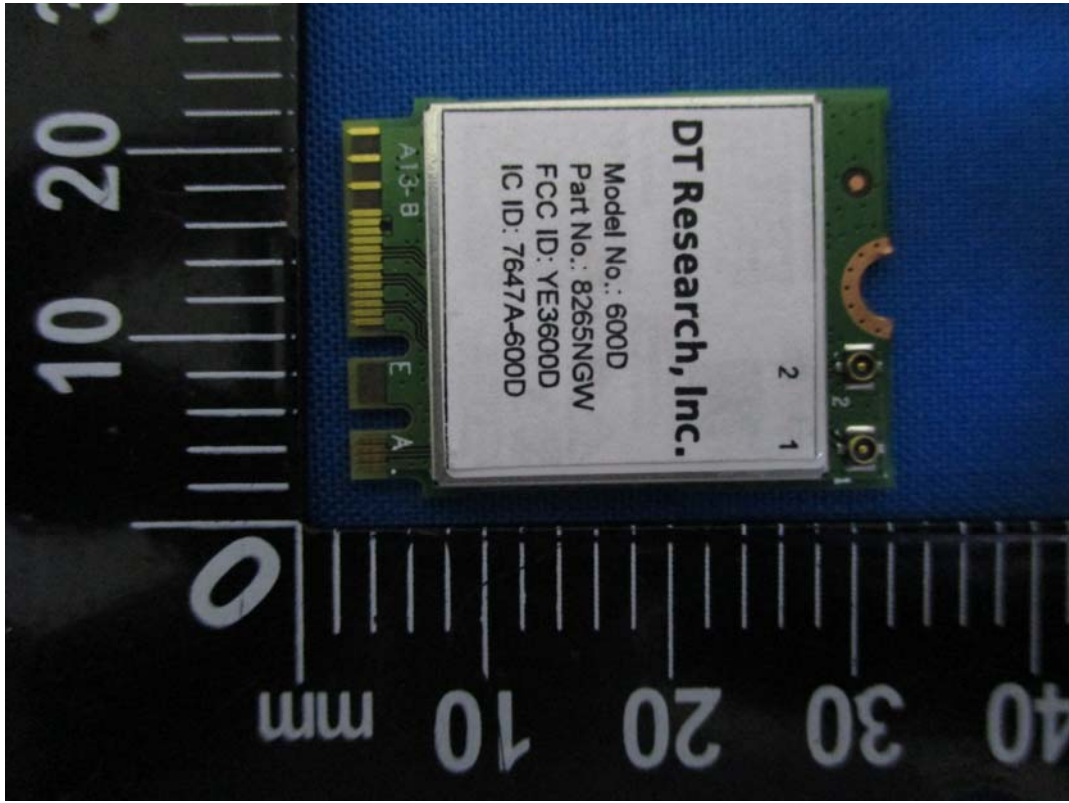
WIFI Module
