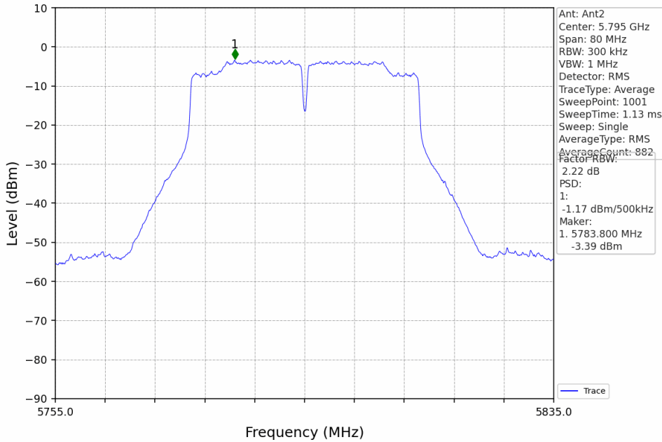
802.11n(HT40)_HCH_5795MHz_MIMO_NTNV
