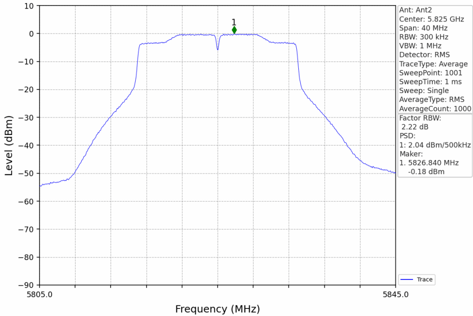
802.11n(HT20)_HCH_5825MHz_MIMO_NTNV
