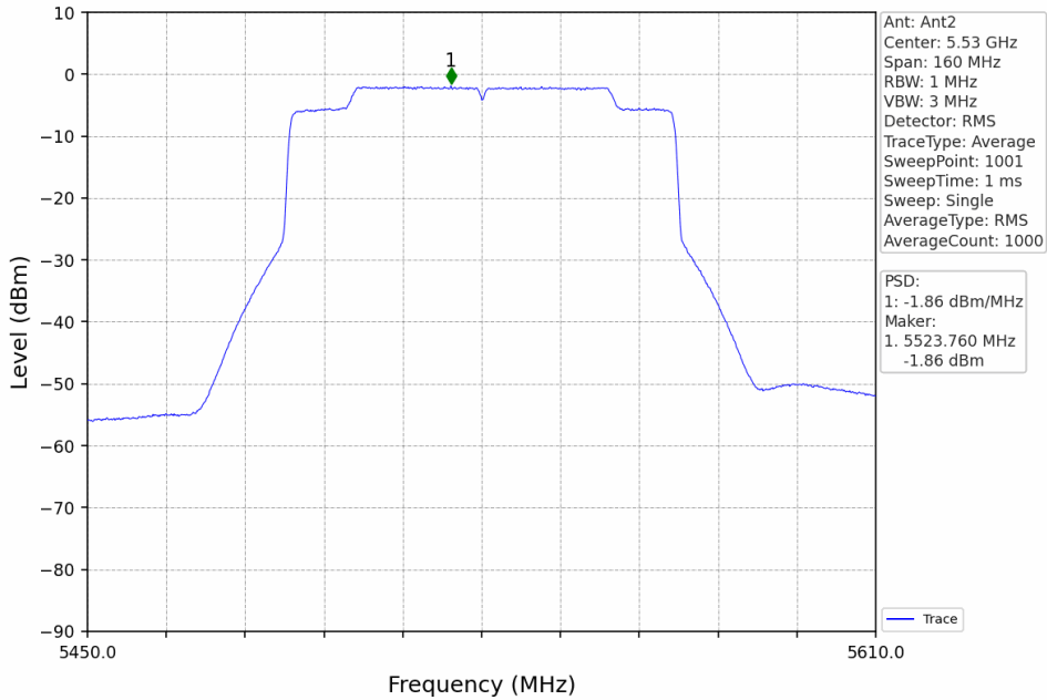
802.11ax(HEW80)_LCH_5530MHz_RU996_Left_MIMO_NTNV
