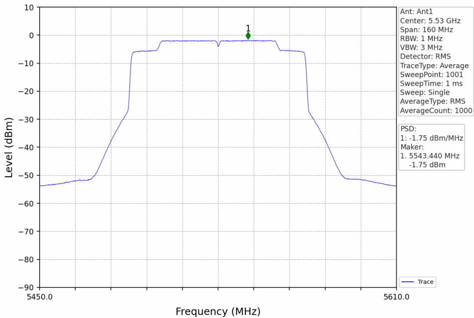
802.11ax(HEW80)_LCH_5530MHz_RU996_Left_Ant1_NTNV
