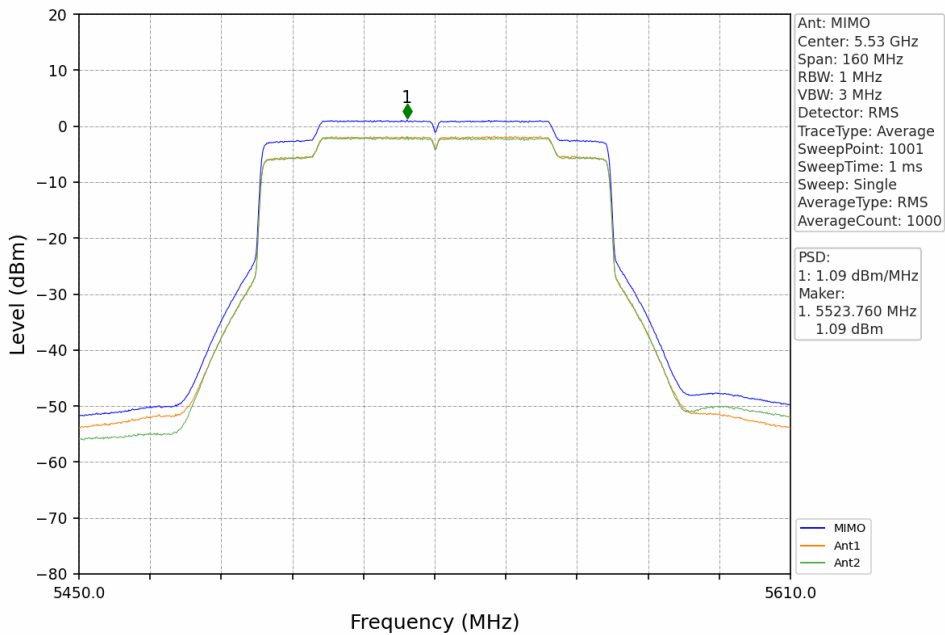
802.11ax(HEW80)_LCH_5530MHz_RU996_Left_MIMO_NTNV
