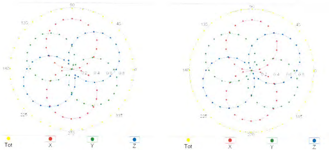
f=1800 MHz,R22
