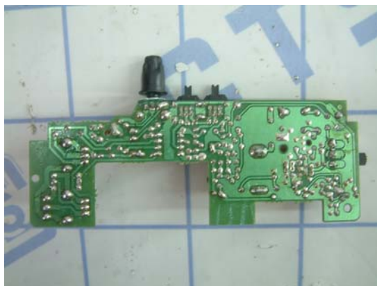
PCB Layout-2
