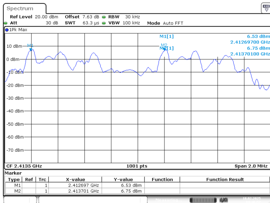
CFS NVNT GFSK 2413MHz Ant1
