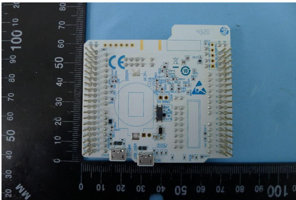
(6) EUT Photo
