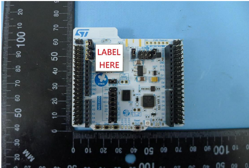
(2) EUT Photo
