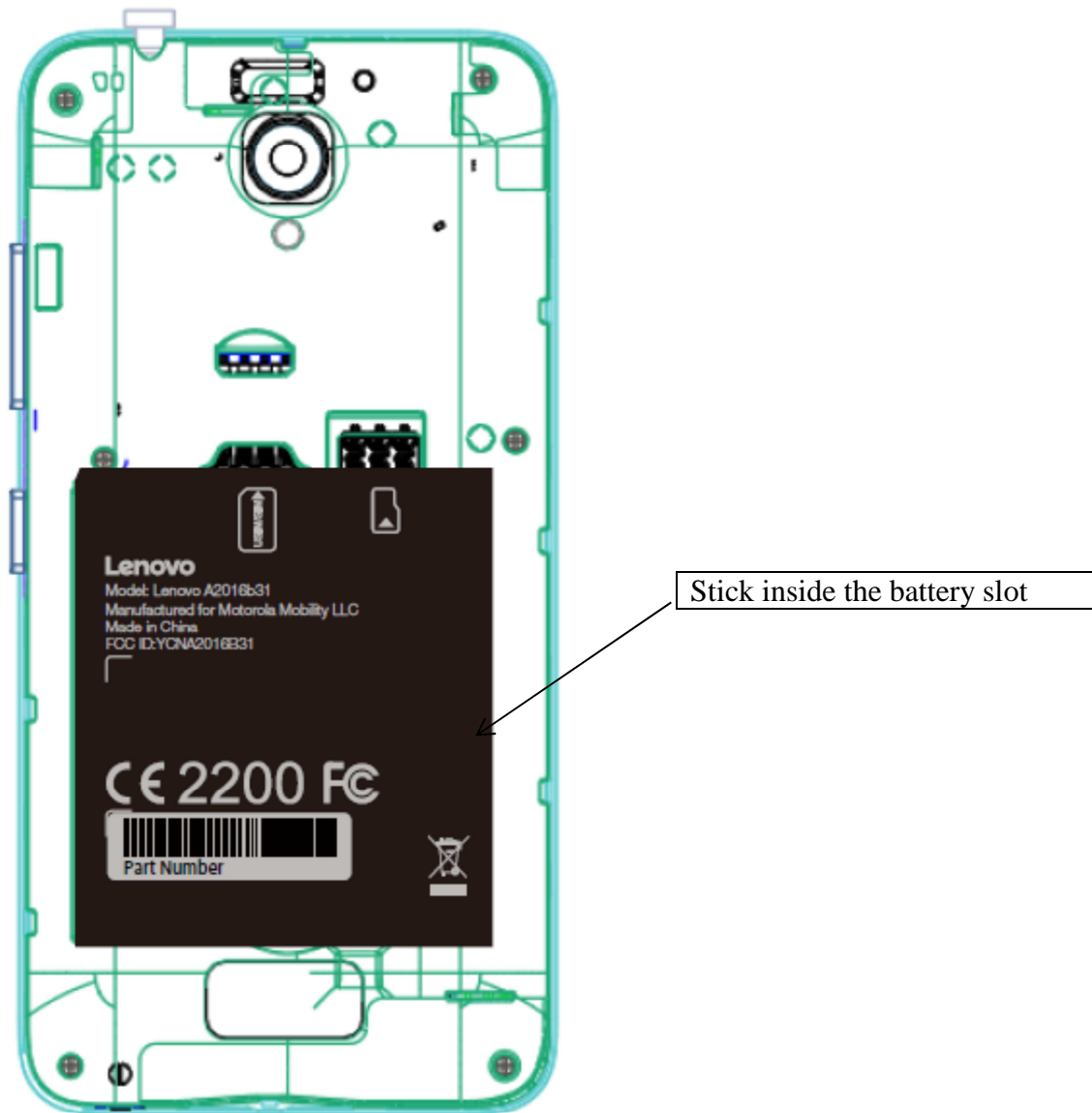
ZAL732 LA 单卡 电池仓标签粘贴位置示意
