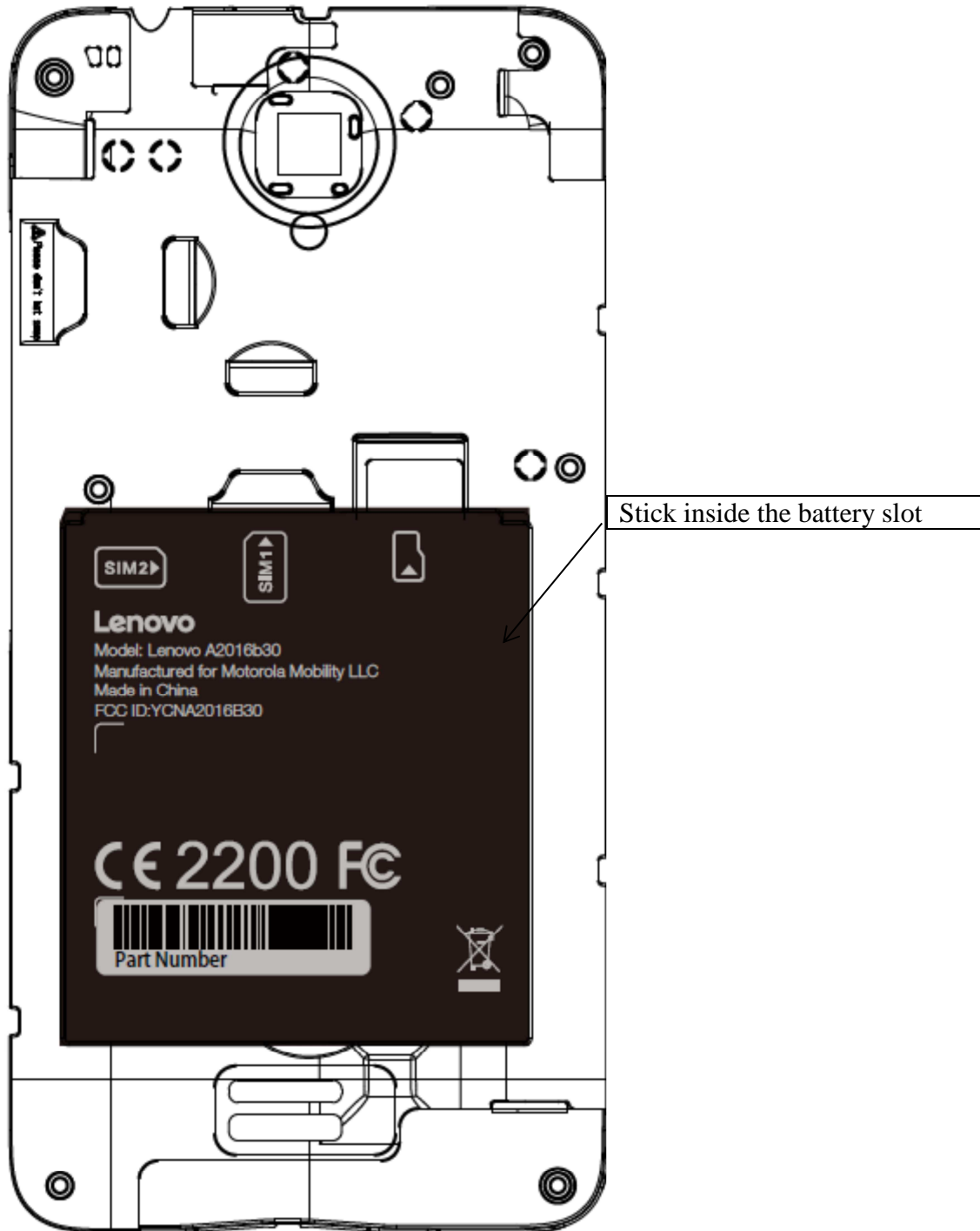
ZAL732 LA 双卡 电池仓标签粘贴位置示意
