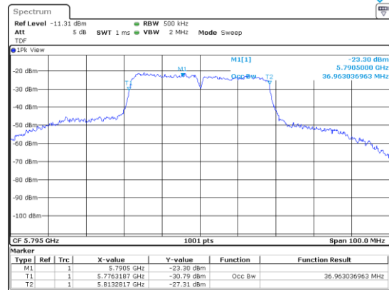
UNII-3 / 802.ac(VHT40)/ 5 795 MHz
