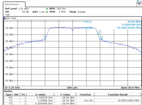
UNII-2A / 802.11ac(VHT20)/ 5 320 MHz
