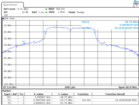
UNII-2C / 802.11ac(VHT20)/ 5 600 MHz
