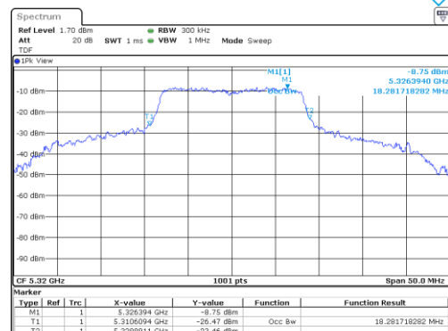
UNII-2A / 802.11a / 5 320 MHz
