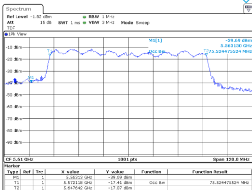
UNII-2C / 802.ac(VHT80)/ 5 610 MHz
