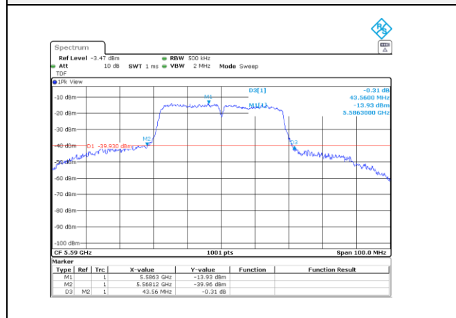
UNII-2C / 802.ac(VHT40)/ 5 590 MHz
