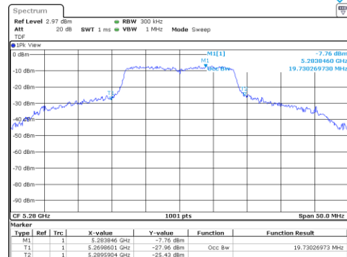
UNII-2A / 802.11a / 5 280 MHz
