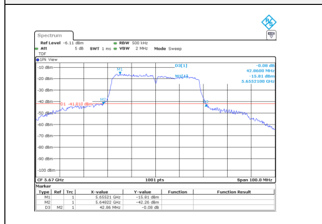
UNII-2C / 802.ac(VHT40)/ 5 670 MHz
