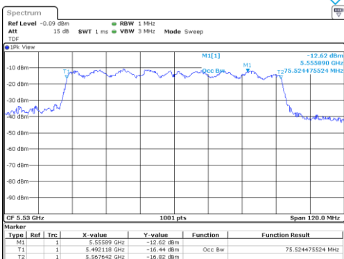
UNII-2C / 802.ac(VHT80)/ 5 530 MHz
