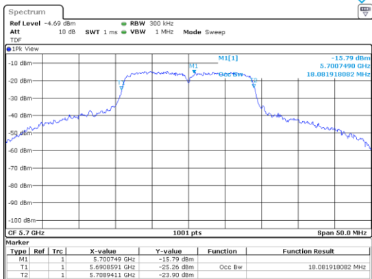
UNII-2C / 802.11ac(VHT20)/ 5 700 MHz
