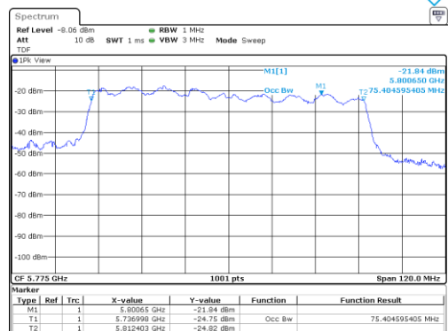
UNII-3 / 802.ac(VHT80)/ 5 775 MHz
