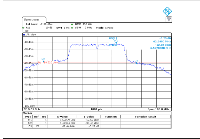
UNII-2C / 802.ac(VHT40)/ 5 510 MHz
