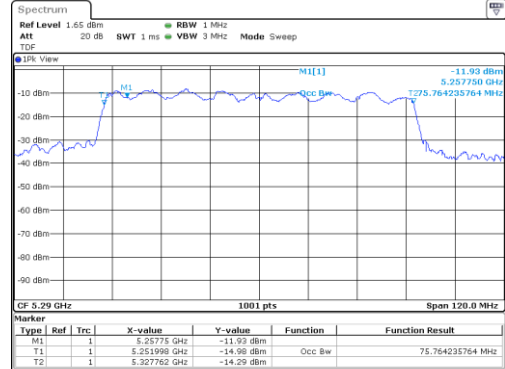
UNII-2A / 802.ac(VHT80)/ 5 290 MHz
