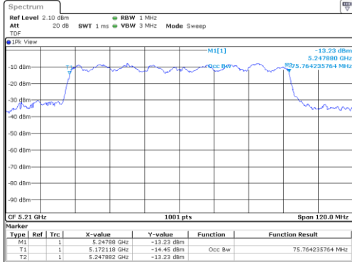
UNII-1 / 802.ac(VHT80)/ 5 210 MHz
