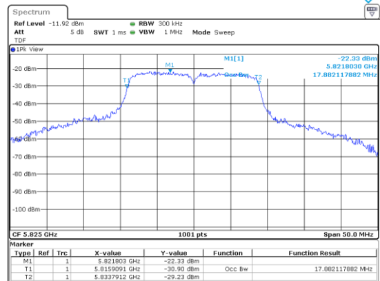
UNII-3 / 802.11ac(VHT20)/ 5 825 MHz
