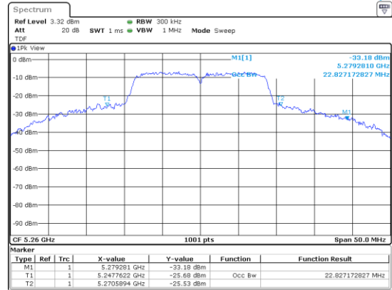
UNII-2A / 802.11ac(VHT20)/ 5 260 MHz
