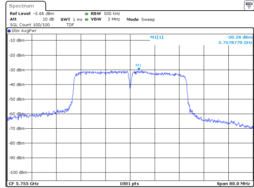
UNII-3 / 802.11ac(VHT40)/ 5 755 MHz
