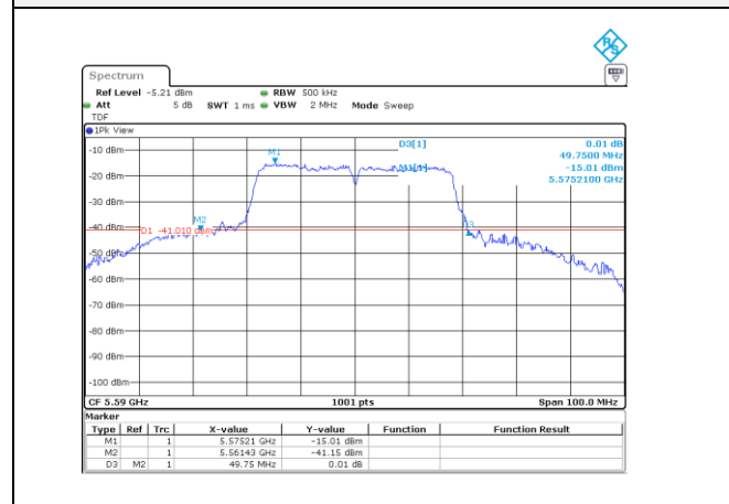
UNII-2C / 802.11n(HT40)/ 5 590 MHz
