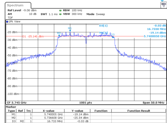
UNII-3 / 802.11ac(VHT20) / 5 745 MHz
