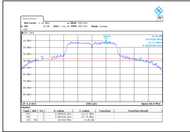
UNII-2C / 802.11n(HT20)/ 5 500 MHz
