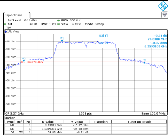
UNII-2A / 802.11n(HT40)/ 5 270 MHz
