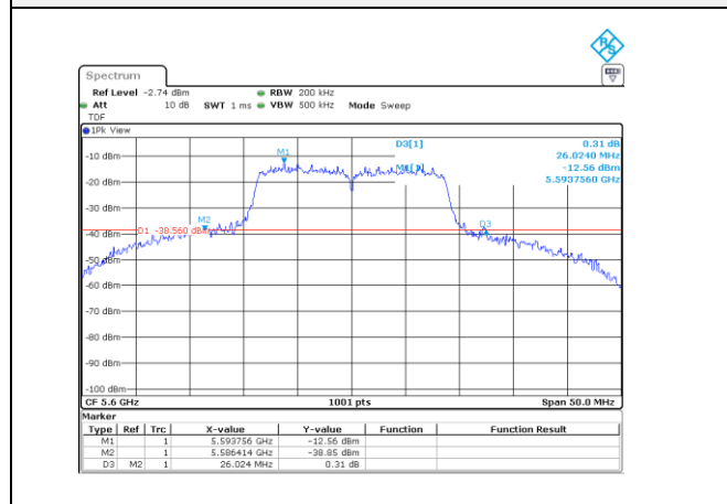
UNII-2C / 802.11n(HT20)/ 5 600 MHz
