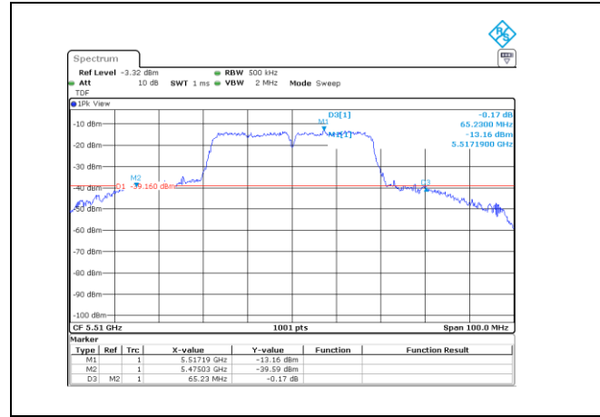
UNII-2C / 802.11n(HT40)/ 5 510 MHz
