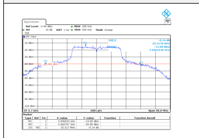
UNII-2C / 802.11a / 5 700 MHz
