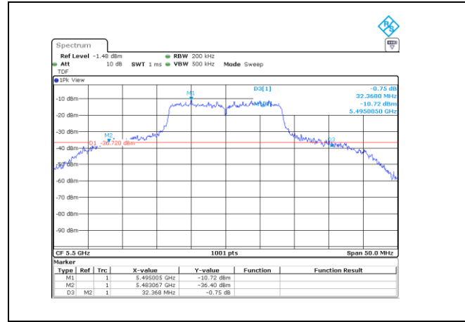
UNII-2C / 802.11a / 5 500 MHz
