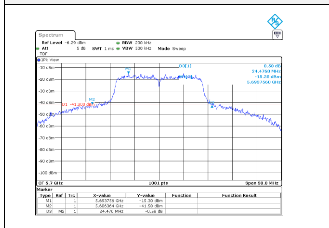
UNII-2C / 802.11n(HT20)/ 5 700 MHz
