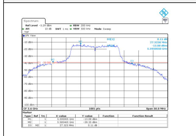
UNII-2C / 802.11a / 5 600 MHz
