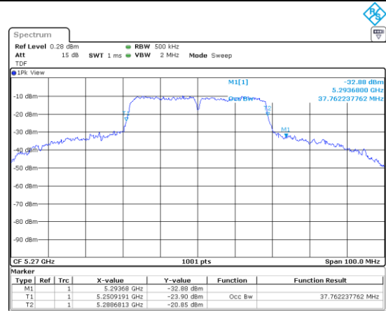
UNII-2A / 802.ac(VHT40)/ 5 270 MHz
