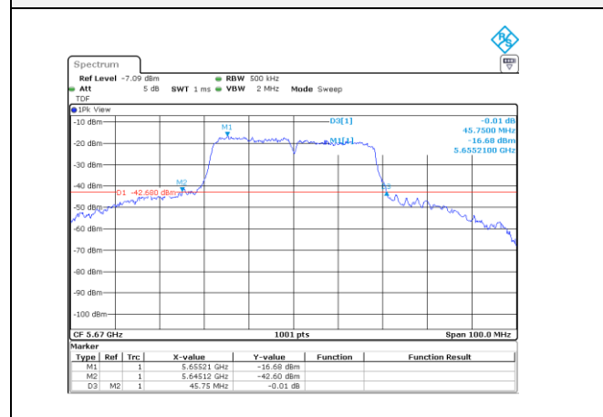
UNII-2C / 802.11n(HT40)/ 5 670 MHz
