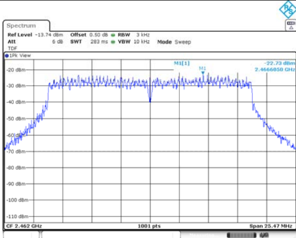
802.11n_HT20 / 2 462 MHz
