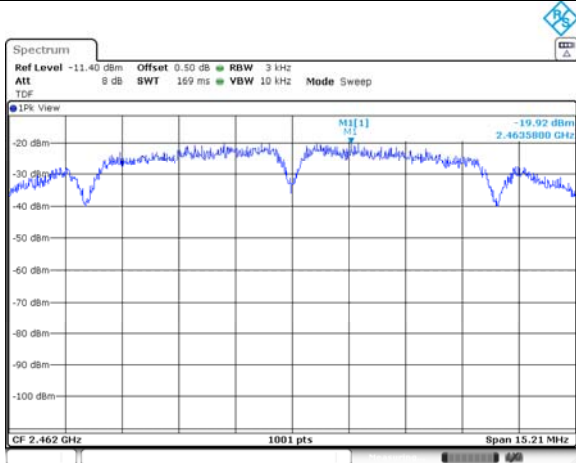
802.11b / 2 462 MHz
