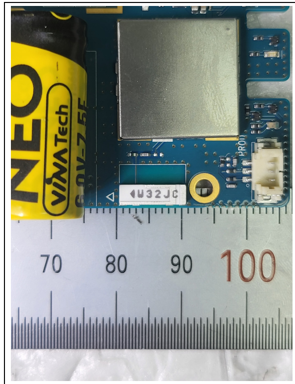
<WLAN Antenna>
