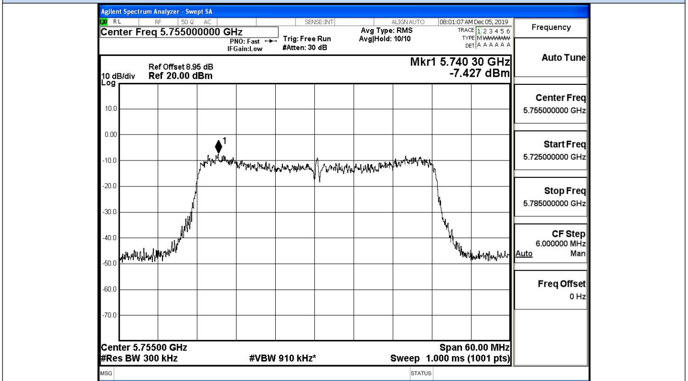
IEEE 802.11ac40 / Channel 151 / 5755MHz
