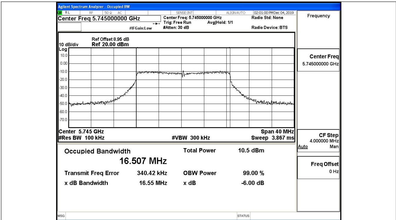
IEEE 802.11a / Channel 149 / 5745MHz
