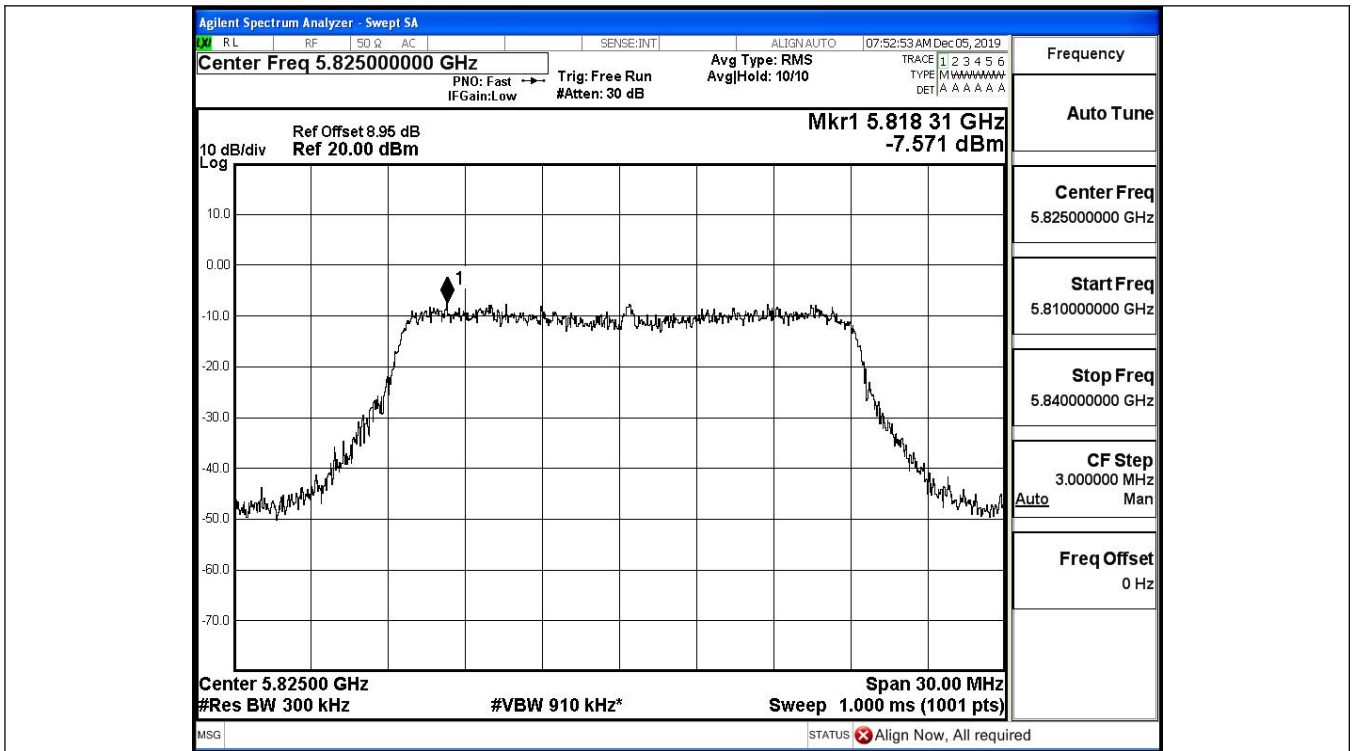
IEEE 802.11ac20 / Channel 165 / 5825MHz
