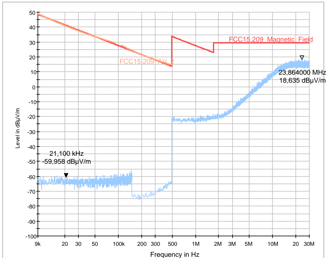
FCC15.209_magn hor+vert
