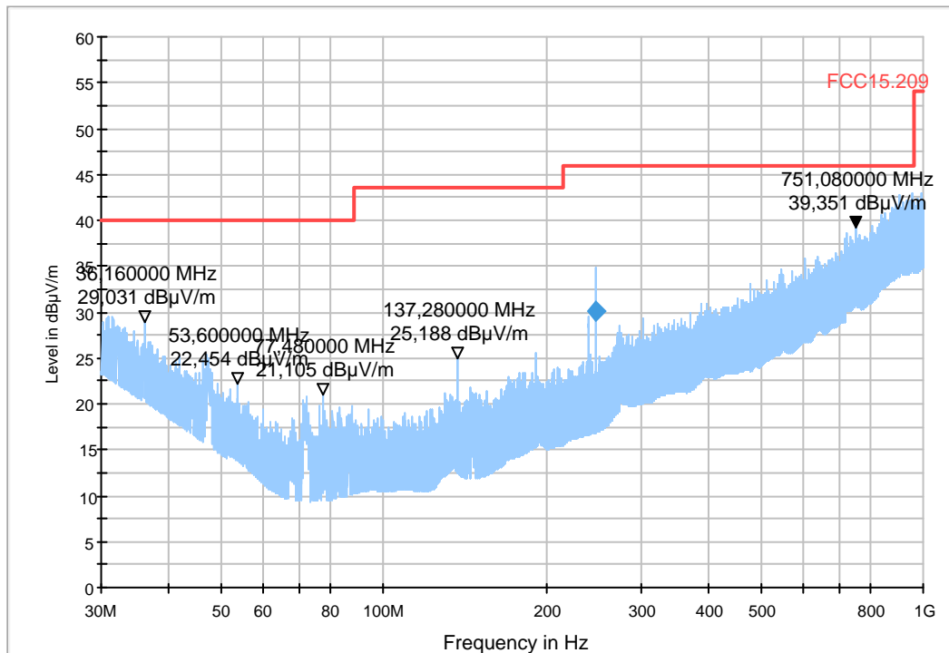
01_FCC15.209_hor+vert_KP0
