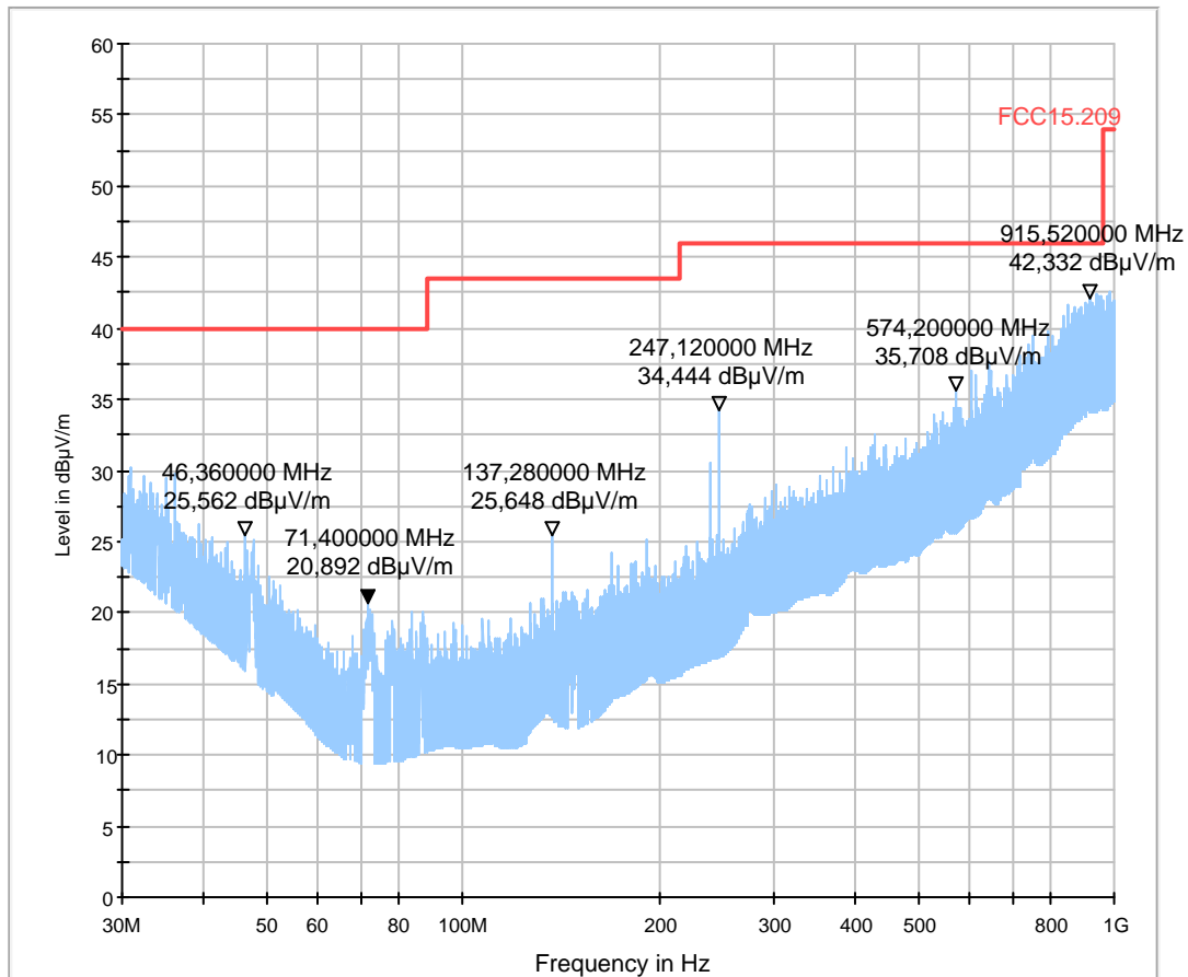
01_FCC15.209_hor+vert_KP0
