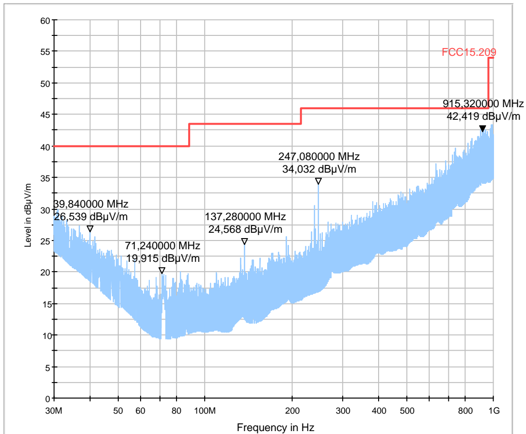
01_FCC15.209_hor+vert_KP0
