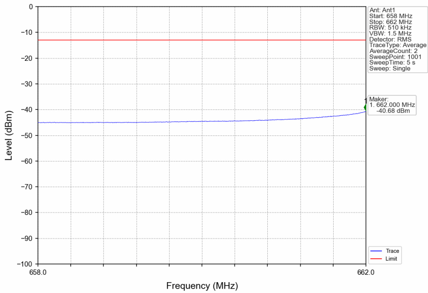
n71_15kHz_SISO_NTNV_15MHz_CP-OFDM QPSK_670.5MHz_Inner_1RB_Left
