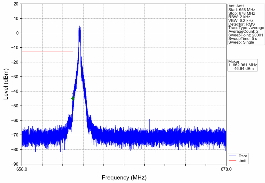
n71_15kHz_SISO_NTNV_15MHz_CP-OFDM QPSK_670.5MHz_Inner_1RB_Left
