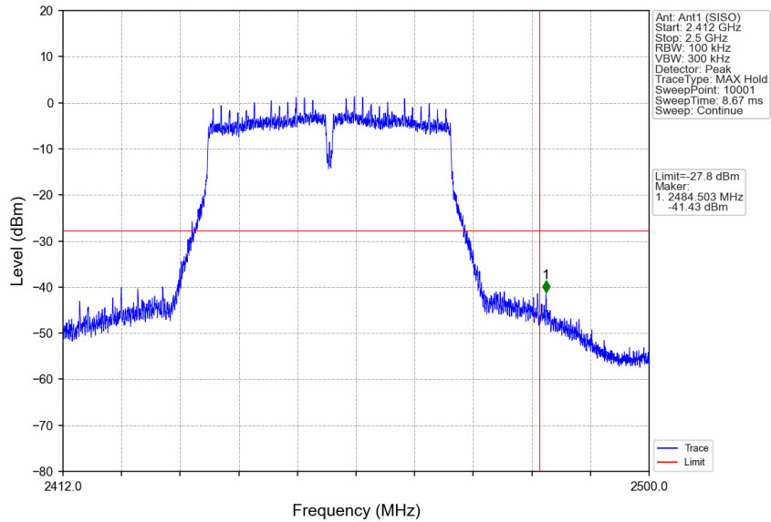
802.11n(HT40)_HCH_2452MHz_Ant1 (SISO)_NTNV
