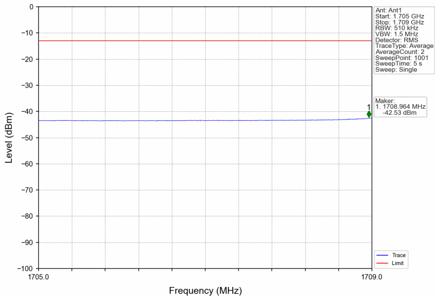
n66_15kHz_SISO_NTNV_20MHz_DFT-s-OFDM QPSK_1720MHz_Inner_1RB_Left
