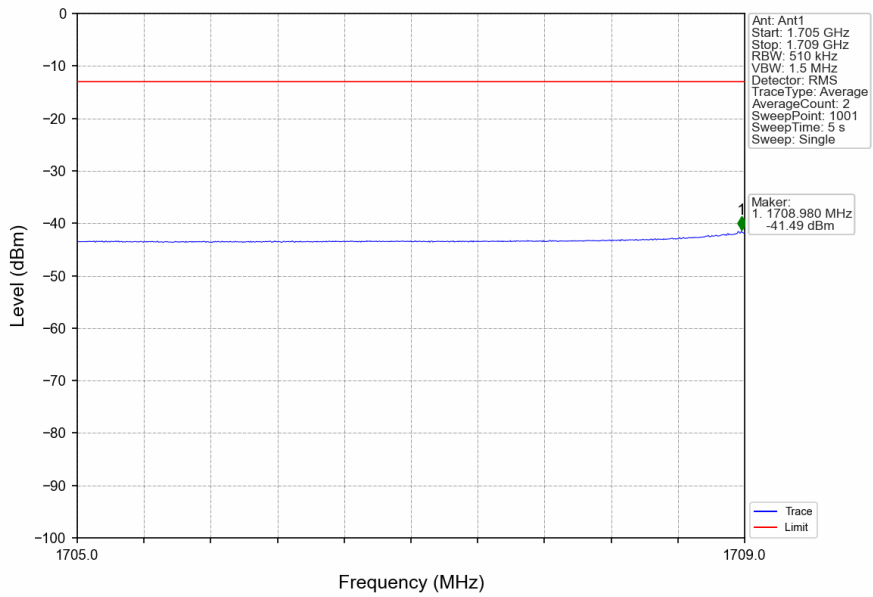
n66_15kHz_SISO_NTNV_20MHz_DFT-s-OFDM QPSK_1720MHz_Edge_1RB_Left
