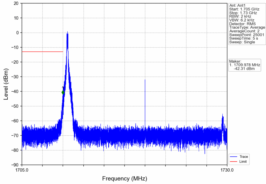
n66_15kHz_SISO_NTNV_20MHz_CP-OFDM QPSK_1720MHz_Edge_1RB_Left
