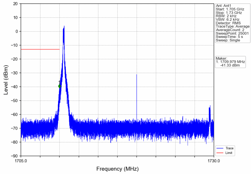
n66_15kHz_SISO_NTNV_20MHz_DFT-s-OFDM QPSK_1720MHz_Edge_1RB_Left
