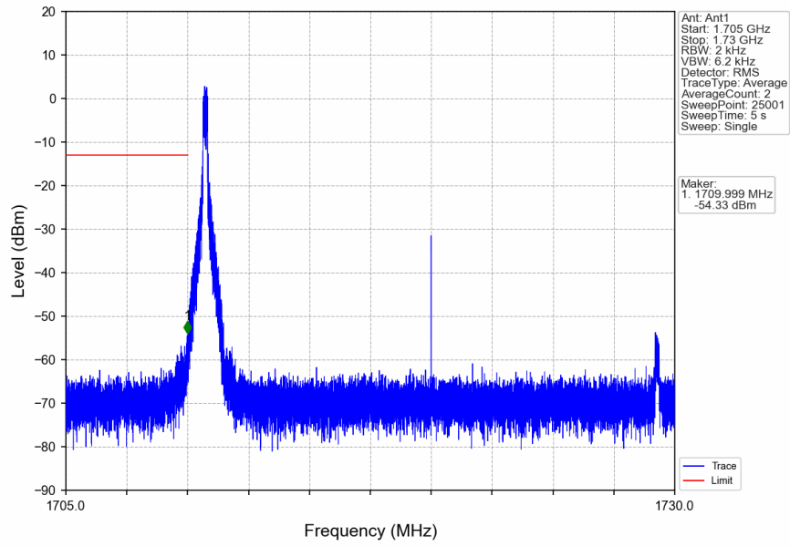
n66_15kHz_SISO_NTNV_20MHz_DFT-s-OFDM QPSK_1720MHz_Inner_1RB_Left
