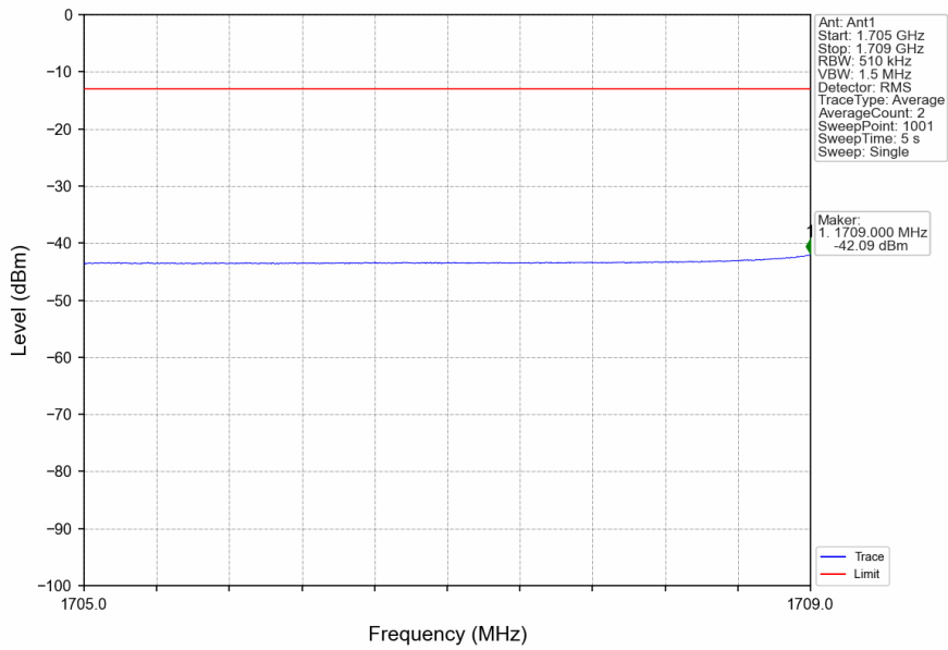
n66_15kHz_SISO_NTNV_20MHz_CP-OFDM QPSK_1720MHz_Edge_1RB_Left
