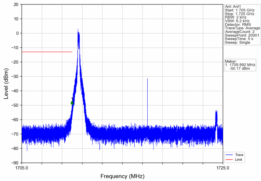
n66_15kHz_SISO_NTNV_15MHz_DFT-s-OFDM QPSK_1717.5MHz_Inner_1RB_Left
