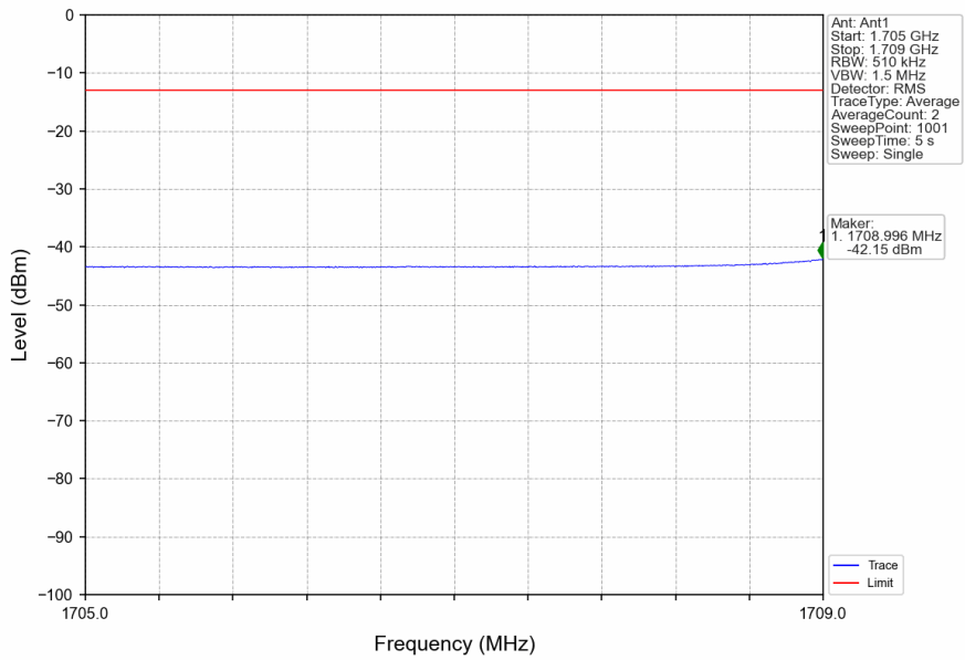
n66_15kHz_SISO_NTNV_15MHz_CP-OFDM QPSK_1717.5MHz_Inner_1RB_Left
