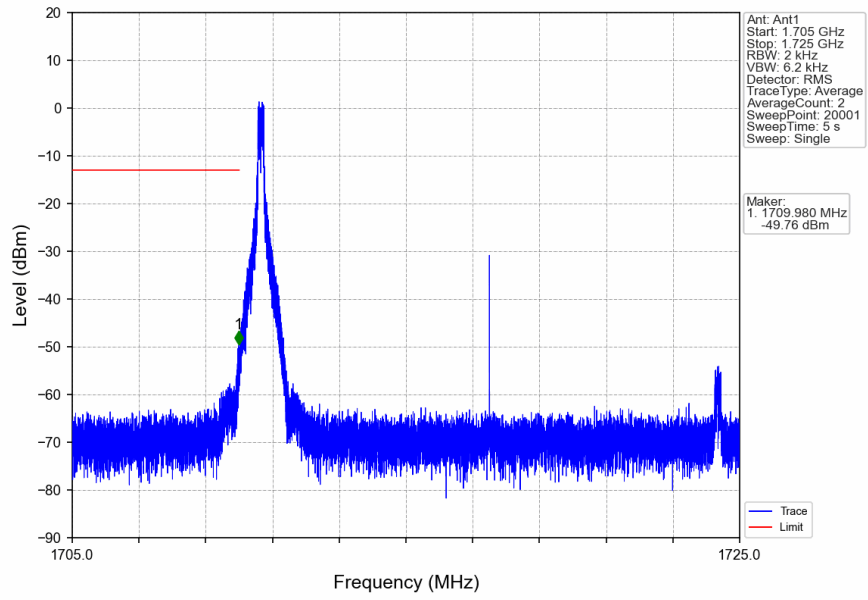
n66_15kHz_SISO_NTNV_15MHz_CP-OFDM QPSK_1717.5MHz_Inner_1RB_Left
