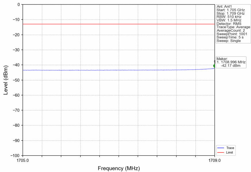
n66_15kHz_SISO_NTNV_15MHz_DFT-s-OFDM QPSK_1717.5MHz_Inner_1RB_Left
