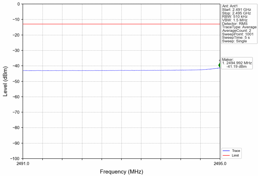
n41_30kHz_SISO_NTNV_90MHz_CP-OFDM QPSK_2541MHz_Inner_1RB_Left
