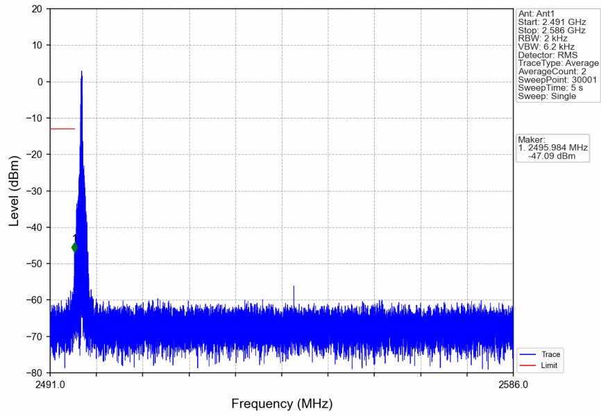
n41_30kHz_SISO_NTNV_90MHz_DFT-s-OFDM_QPSK_2541MHz_Inner_1RB_Left
