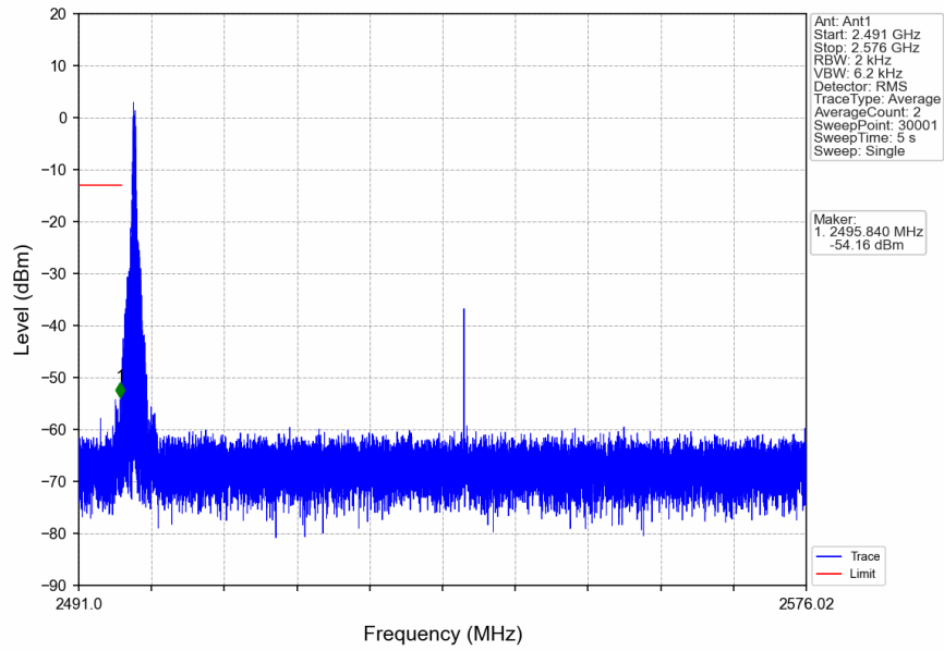
n41_30kHz_SISO_NTNV_80MHz_CP-OFDM QPSK_2536.02MHz_Inner_1RB_Left
