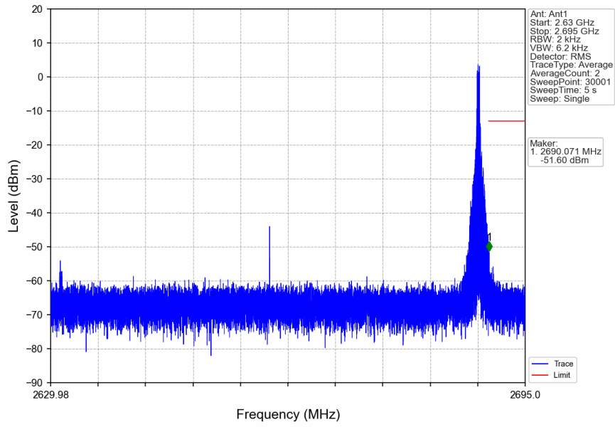
n41_30kHz_SISO_NTNV_60MHz_DFT-s-OFDM_QPSK_2659.98MHz_Inner_1RB_Right
