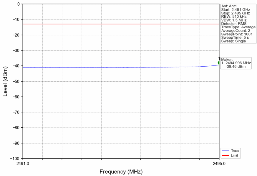
n41_30kHz_SISO_NTNV_60MHz_CP-OFDM QPSK_2526MHz_Inner_1RB_Left
