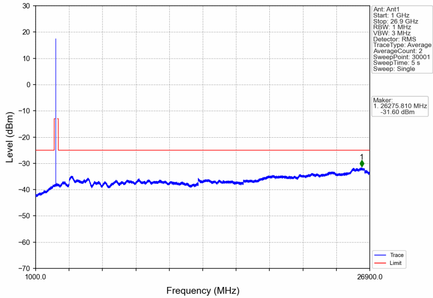
n41_30kHz_SISO_NTNV_60MHz_CP-OFDM QPSK_2592.99MHz_Edge_1RB_Left
