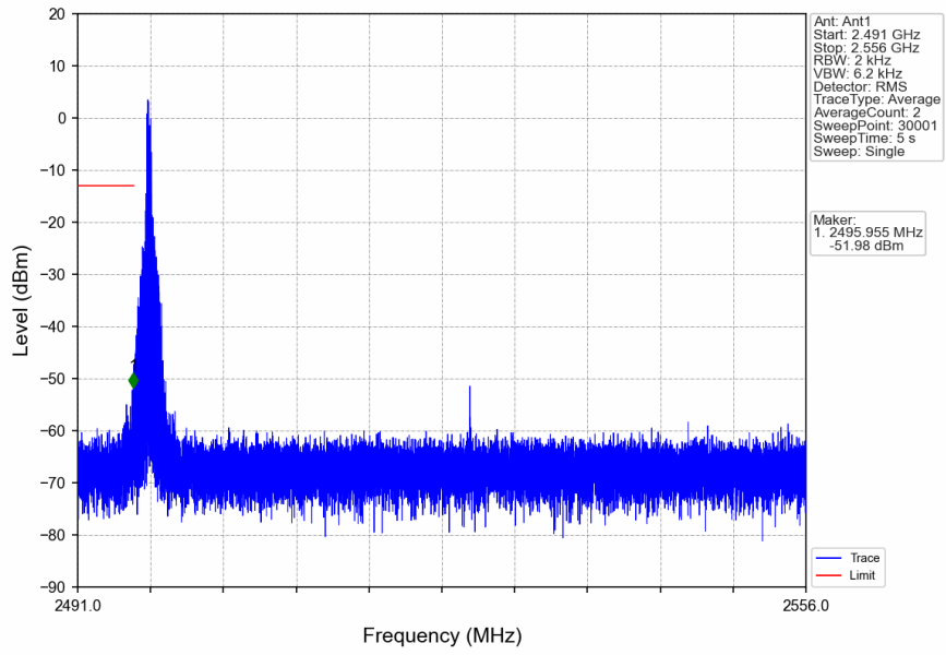
n41_30kHz_SISO_NTNV_60MHz_CP-OFDM QPSK_2526MHz_Inner_1RB_Left
