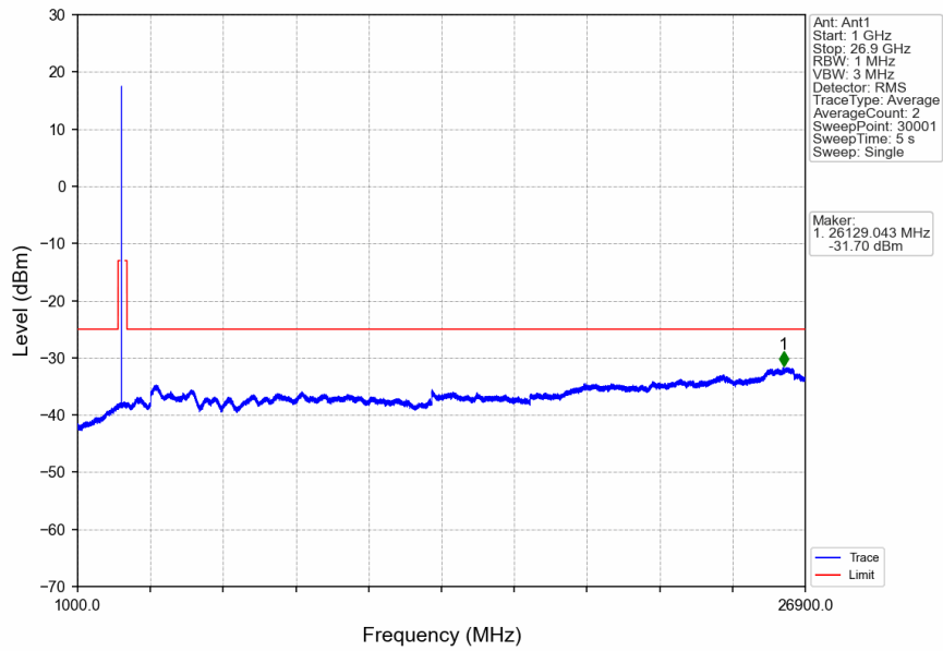
n41_30kHz_SISO_NTNV_60MHz_DFT-s-OFDM QPSK_2592.99MHz_Edge_1RB_Left
