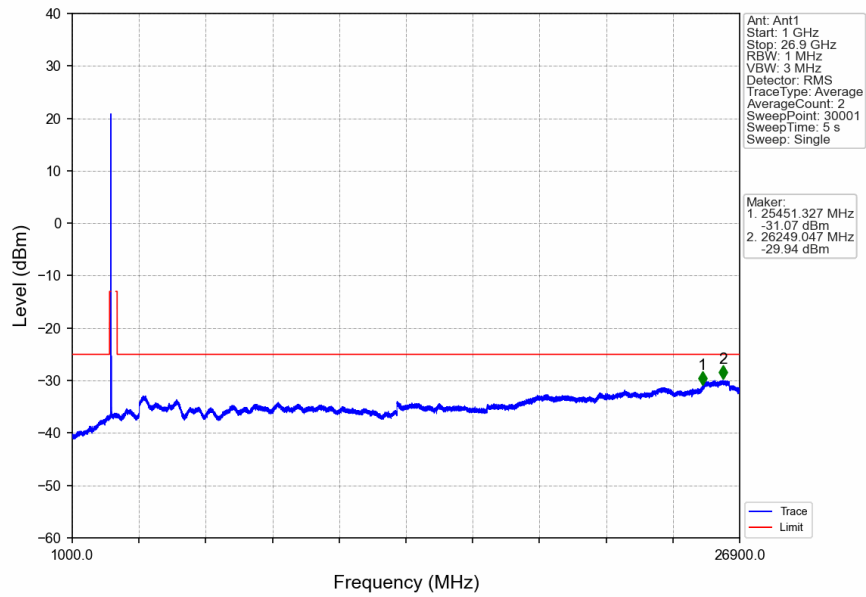
n41_30kHz_SISO_NTNV_50MHz_CP-OFDM QPSK_2521.02MHz_Inner_1RB_Left
