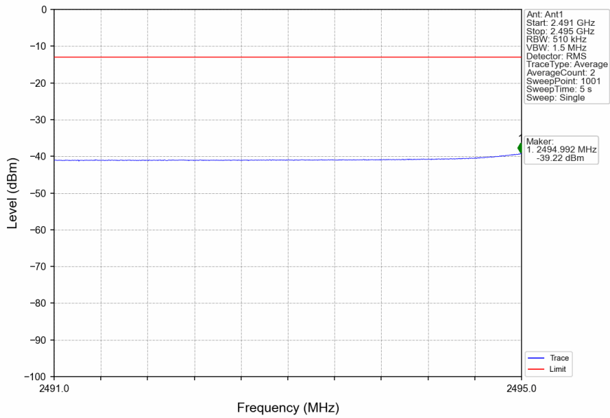
n41_30kHz_SISO_NTNV_60MHz_DFT-s-OFDM_QPSK_2526MHz_Inner_1RB_Left
