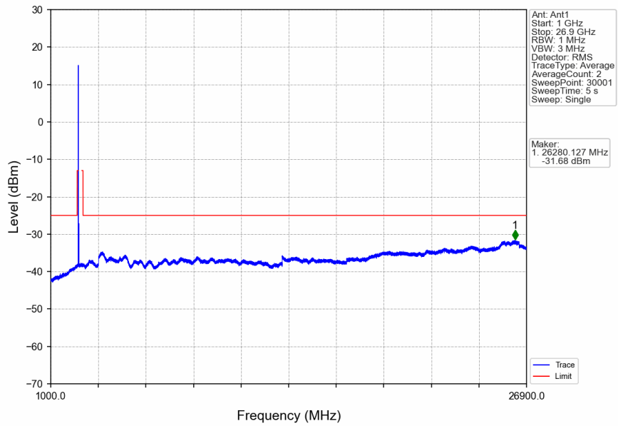
n41_30kHz_SISO_NTNV_60MHz_DFT-s-OFDM_QPSK_2526MHz_Edge_1RB_Left
