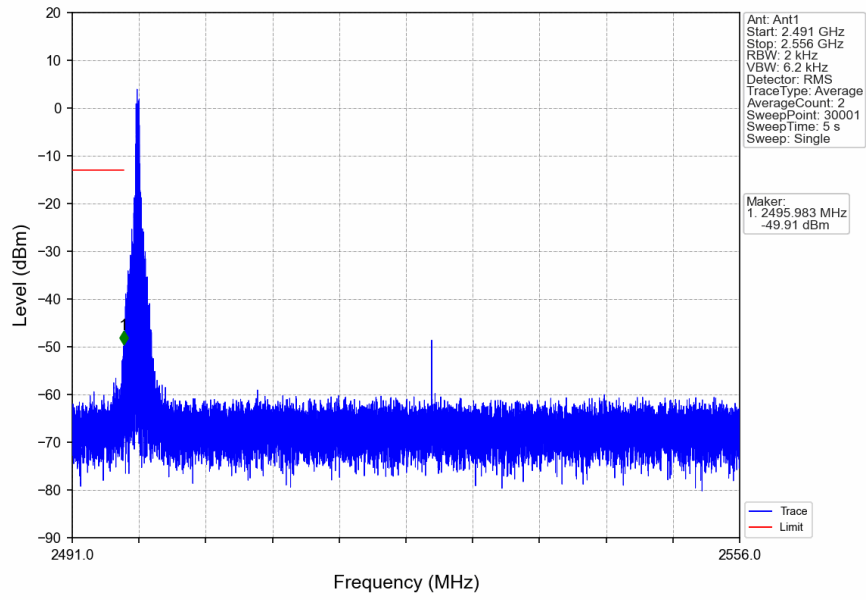
n41_30kHz_SISO_NTNV_60MHz_DFT-s-OFDM_QPSK_2526MHz_Inner_1RB_Left
