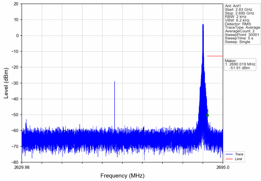
n41_30kHz_SISO_NTNV_60MHz_DFT-s-OFDM PI/2 BPSK_2659.98MHz_Inner_1RB_Right
