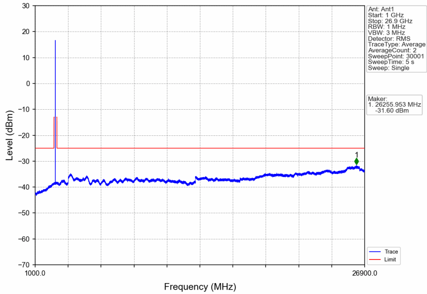
n41_30kHz_SISO_NTNV_20MHz_CP-OFDM QPSK_2592.99MHz_Edge_1RB_Left
