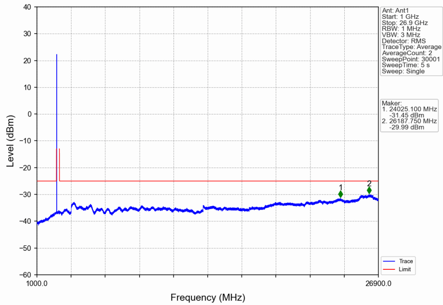
n41_30kHz_SISO_NTNV_20MHz_CP-OFDM QPSK_2506.02MHz_Inner_1RB_Left
