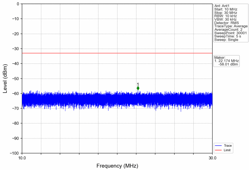
n41_30kHz_SISO_NTNV_20MHz_CP-OFDM QPSK_2506.02MHz_Edge_1RB_Left
