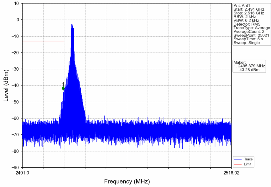
n41_30kHz_SISO_NTNV_20MHz_CP-OFDM_QPSK_2506.02MHz_Edge_1RB_Left
