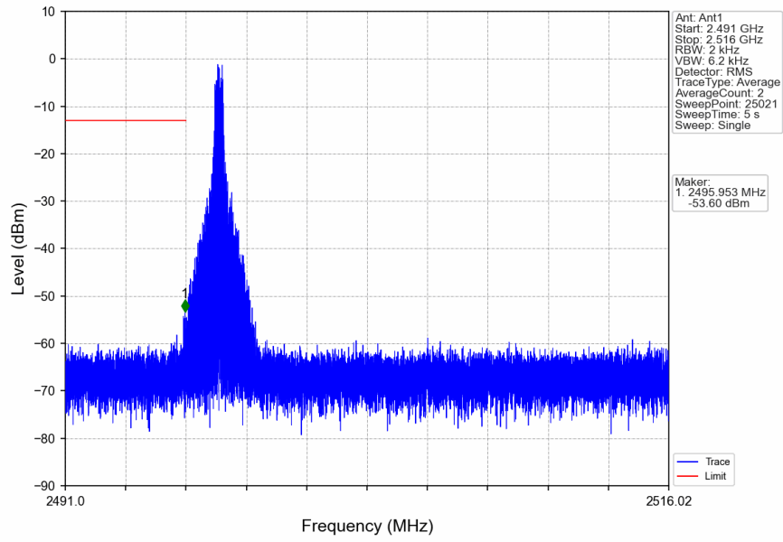
n41_30kHz_SISO_NTNV_20MHz_CP-OFDM QPSK_2506.02MHz_Inner_1RB_Left
