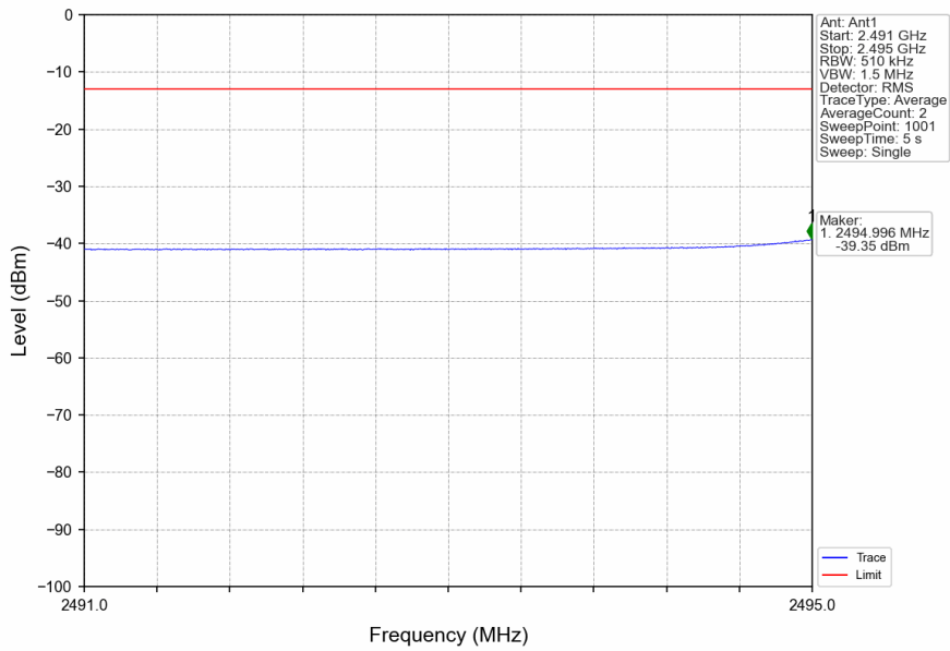
n41_30kHz_SISO_NTNV_20MHz_CP-OFDM QPSK_2506.02MHz_Inner_1RB_Left
