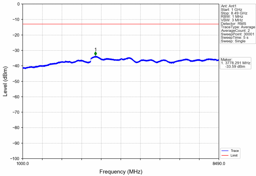
n5_15kHz_SISO_NTNV_20MHz_CP-OFDM QPSK_834MHz_Inner_1RB_Left
