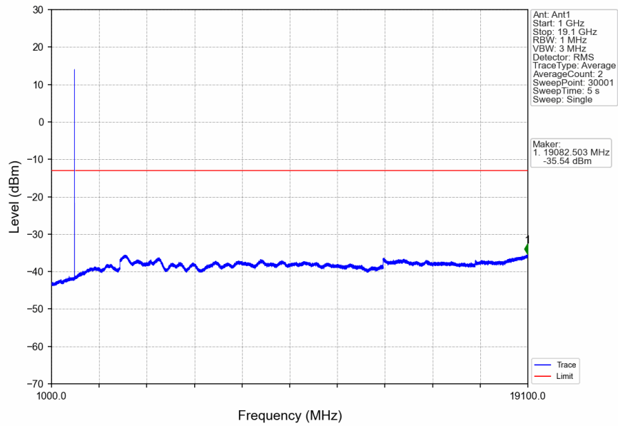
n2_15kHz_SISO_NTNV_20MHz_CP-OFDM QPSK_1880MHz_Edge_1RB_Left
