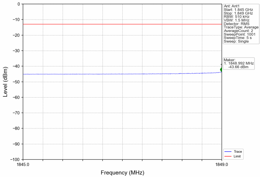
n2_15kHz_SISO_NTNV_20MHz_CP-OFDM QPSK_1860MHz_Inner_1RB_Left
