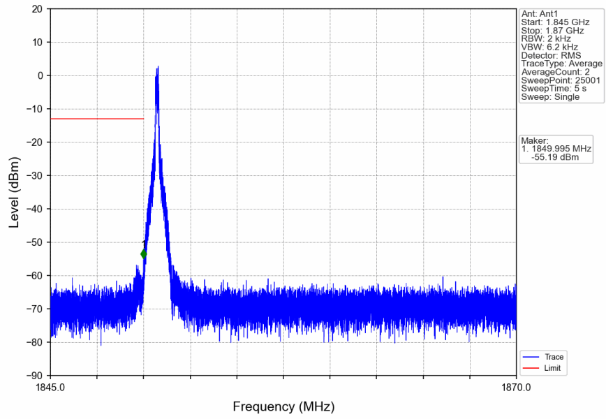
n2_15kHz_SISO_NTNV_20MHz_CP-OFDM QPSK_1860MHz_Inner_1RB_Left
