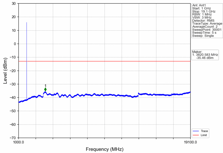
n2_15kHz_SISO_NTNV_20MHz_DFT-s-OFDM QPSK_1860MHz_Inner_1RB_Left
