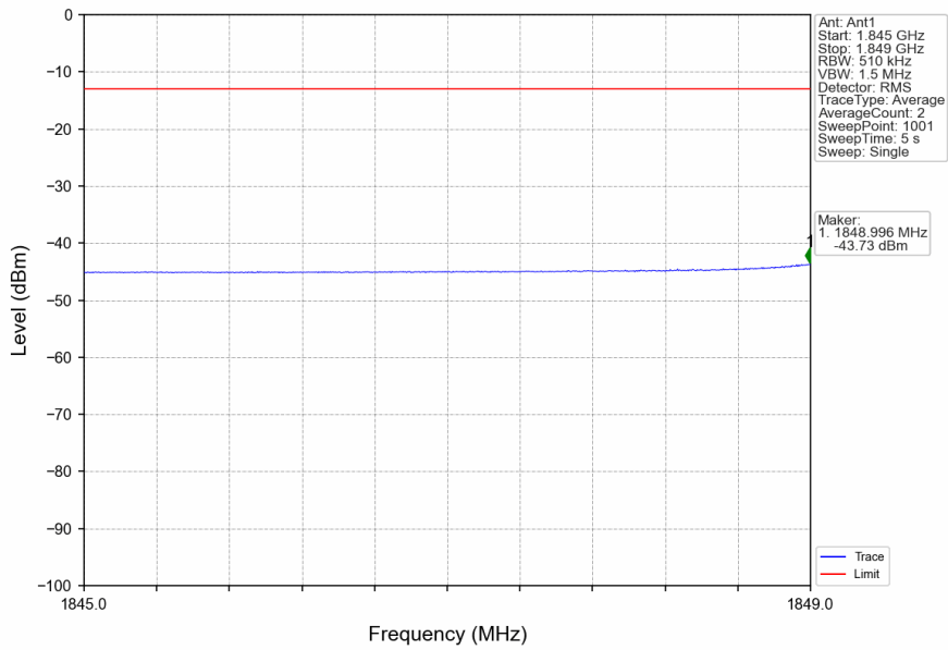
n2_15kHz_SISO_NTNV_20MHz_DFT-s-OFDM QPSK_1860MHz_Inner_1RB_Left
