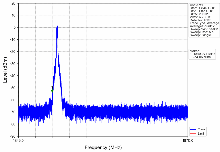
n2_15kHz_SISO_NTNV_20MHz_DFT-s-OFDM QPSK_1860MHz_Inner_1RB_Left
