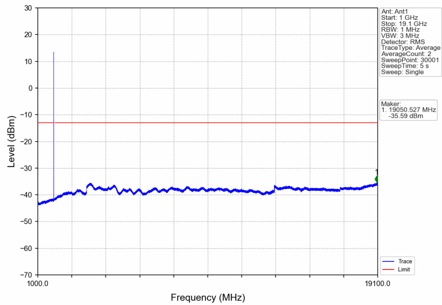
n2_15kHz_SISO_NTNV_20MHz_CP-OFDM_QPSK_1860MHz_Edge_1RB_Left
