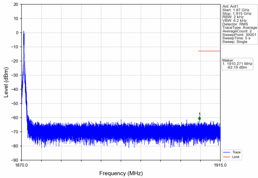
n2_15kHz_SISO_NTNV_20MHz_DFT-s-OFDM QPSK_1880MHz_Edge_1RB_Left
