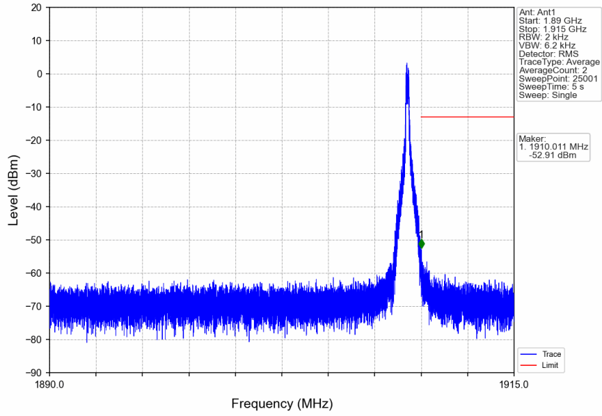
n2_15kHz_SISO_NTNV_20MHz_DFT-s-OFDM QPSK_1900MHz_Inner_1RB_Right
