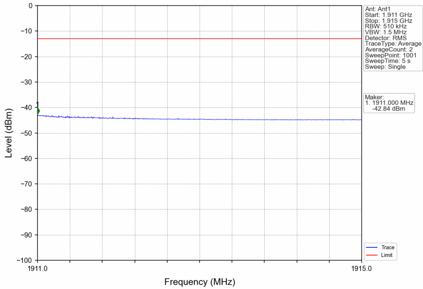
n2_15kHz_SISO_NTNV_20MHz_DFT-s-OFDM QPSK_1900MHz_Inner_1RB_Right
