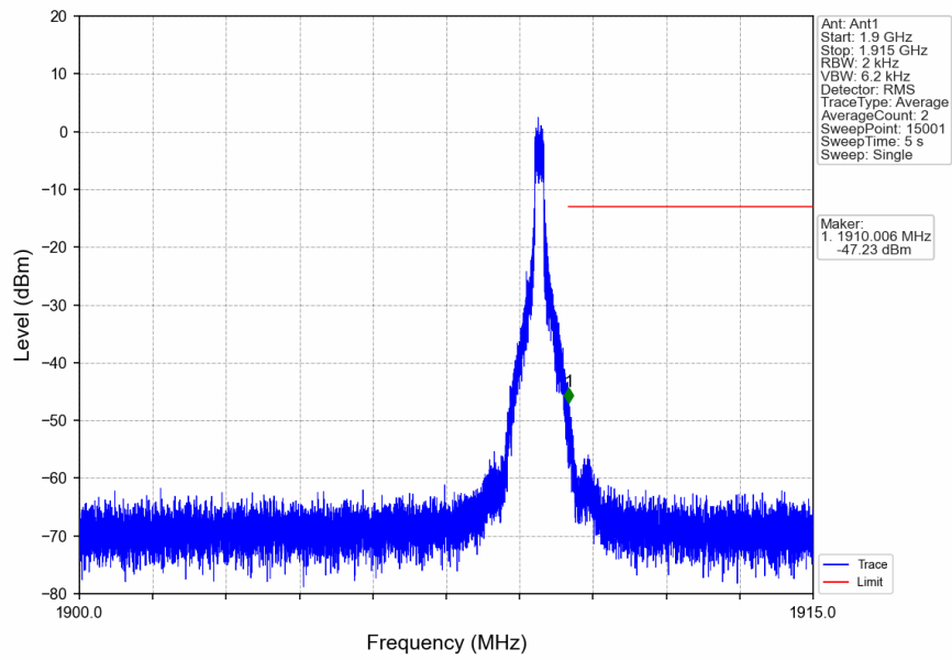
n2_15kHz_SISO_NTNV_10MHz_CP-OFDM QPSK_1905MHz_Inner_1RB_Right
