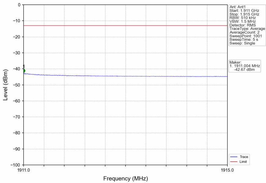
n2_15kHz_SISO_NTNV_10MHz_CP-OFDM QPSK_1905MHz_Inner_1RB_Right
