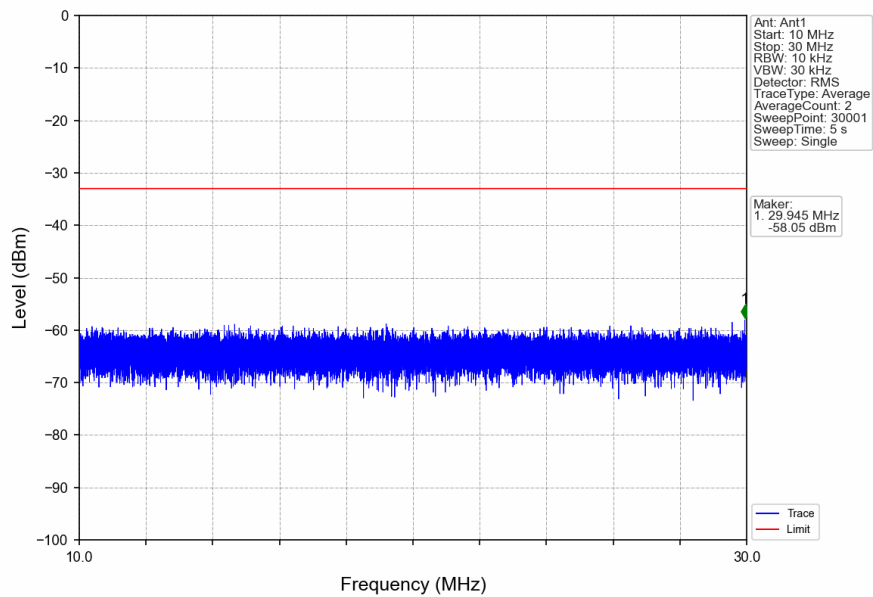
n2_15kHz_SISO_NTNV_10MHz_DFT-s-OFDM QPSK_1855MHz_Edge_1RB_Left
