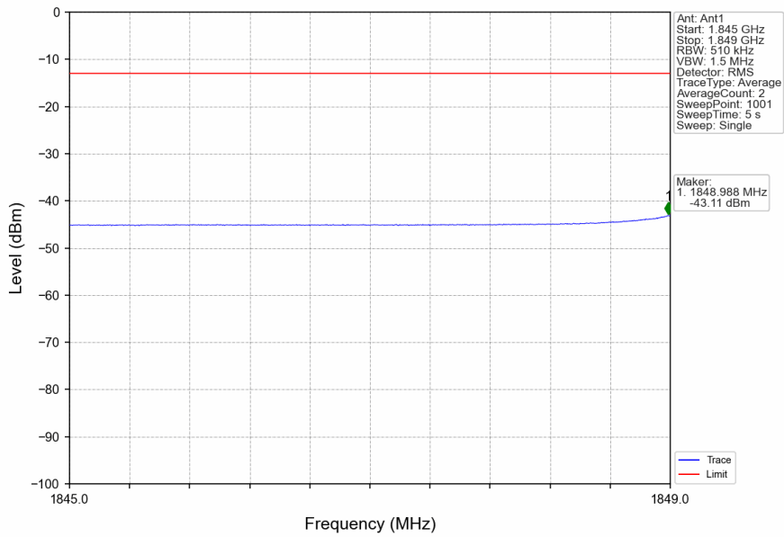
n2_15kHz_SISO_NTNV_10MHz_CP-OFDM QPSK_1855MHz_Edge_1RB_Left
