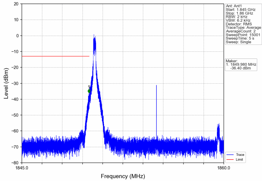
n2_15kHz_SISO_NTNV_10MHz_CP-OFDM QPSK_1855MHz_Edge_1RB_Left
