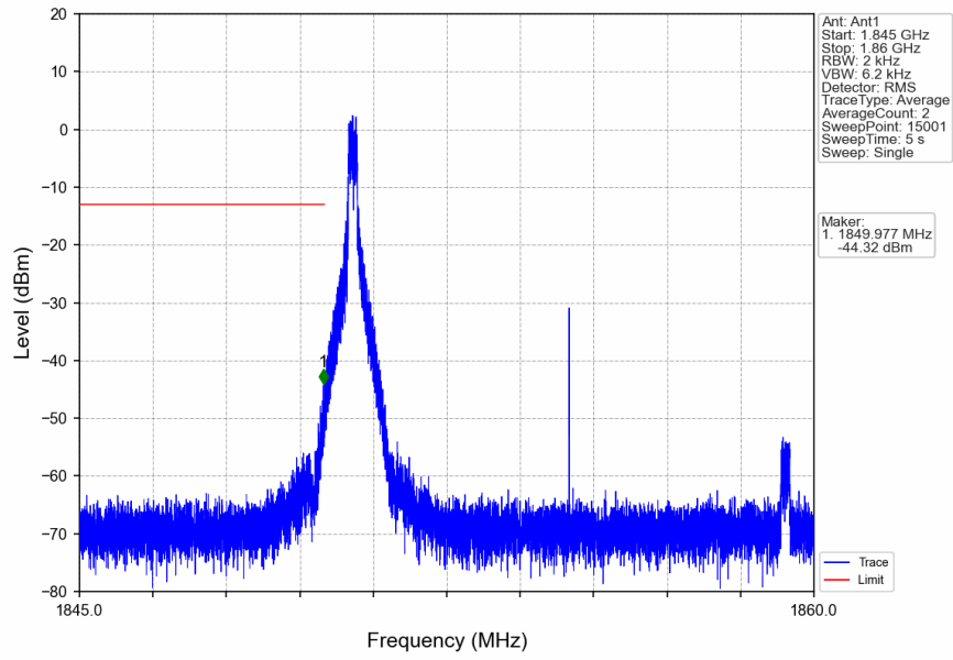
n2_15kHz_SISO_NTNV_10MHz_DFT-s-OFDM QPSK_1855MHz_Inner_1RB_Left
