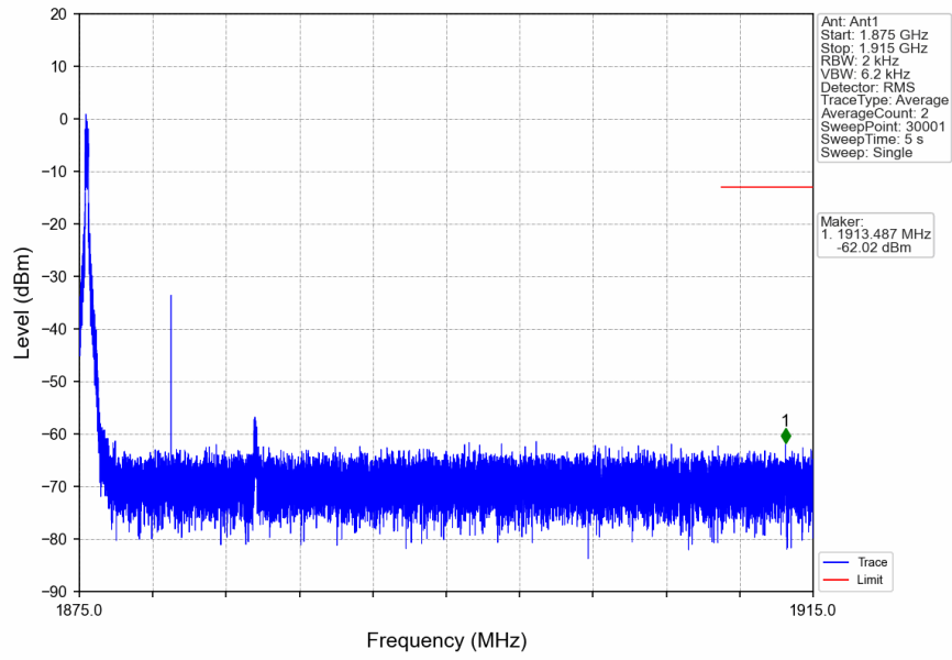
n2_15kHz_SISO_NTNV_10MHz_CP-OFDM QPSK_1880MHz_Edge_1RB_Left
