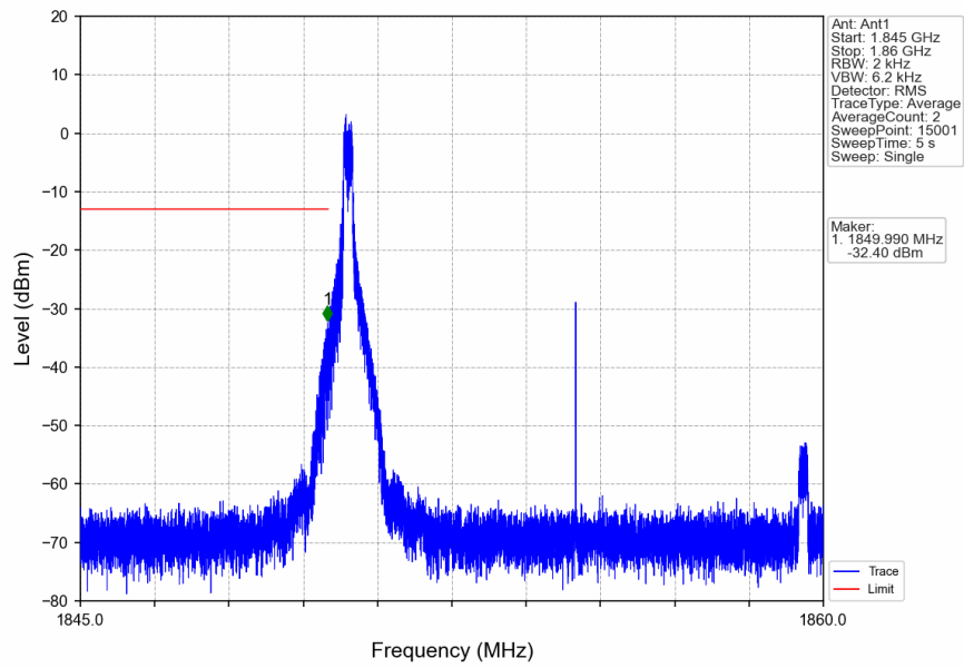
n2_15kHz_SISO_NTNV_10MHz_DFT-s-OFDM_QPSK_1855MHz_Edge_1RB_Left
