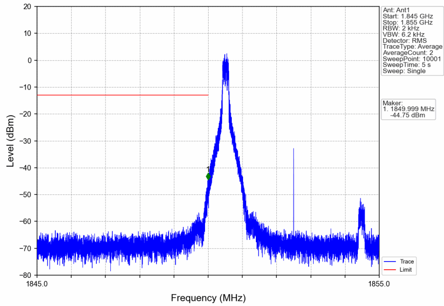
n2_15kHz_SISO_NTNV_5MHz_DFT-s-OFDM QPSK_1852.5MHz_Inner_1RB_Left
