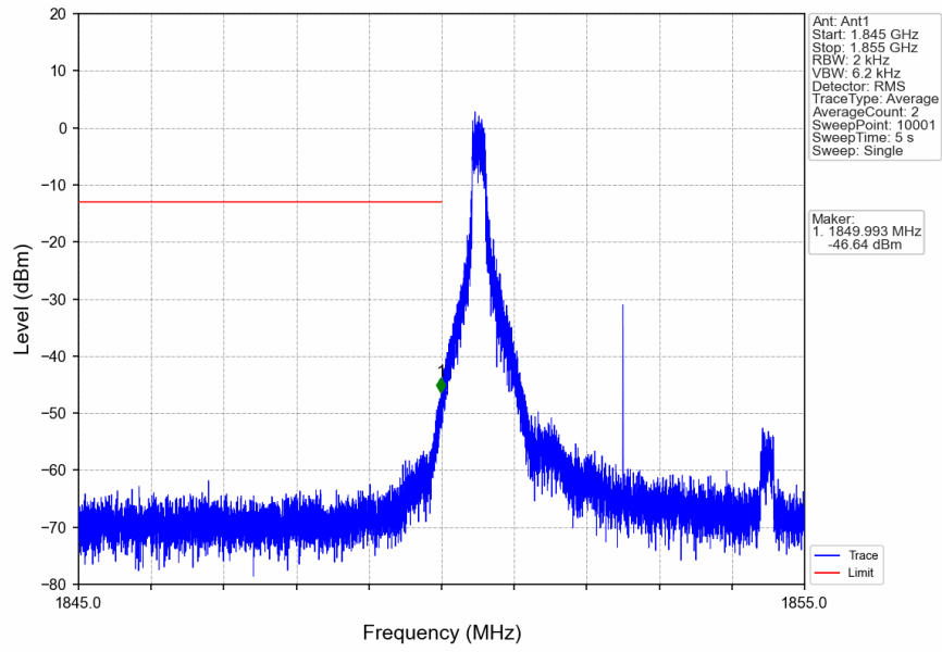
n2_15kHz_SISO_NTNV_5MHz_CP-OFDM QPSK_1852.5MHz_Inner_1RB_Left
