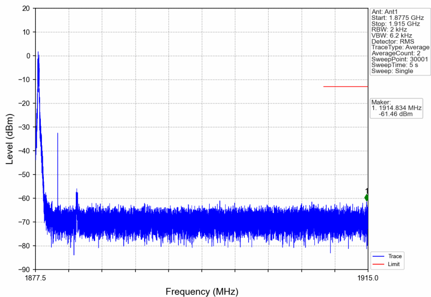
n2_15kHz_SISO_NTNV_5MHz_CP-OFDM QPSK_1880MHz_Edge_1RB_Left
