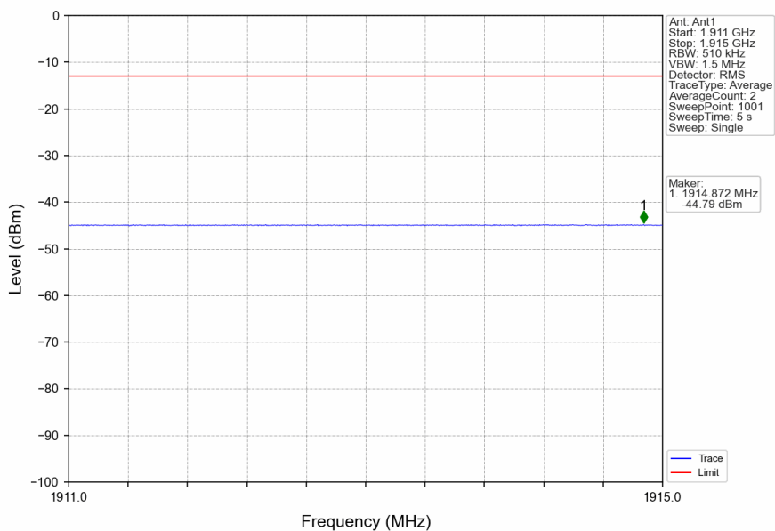
n2_15kHz_SISO_NTNV_5MHz_CP-OFDM QPSK_1880MHz_Edge_1RB_Left
