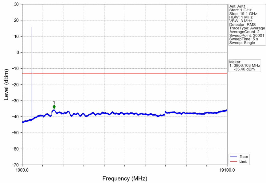
n2_15kHz_SISO_NTNV_5MHz_CP-OFDM QPSK_1852.5MHz_Inner_1RB_Left
