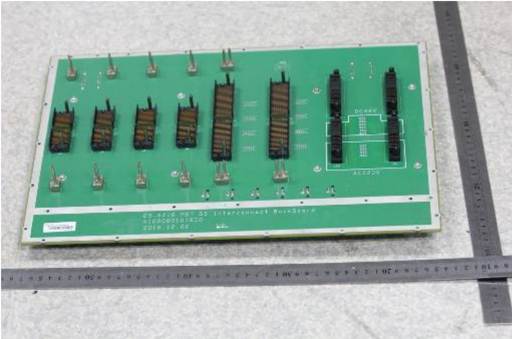
EUT – ICB Top View
