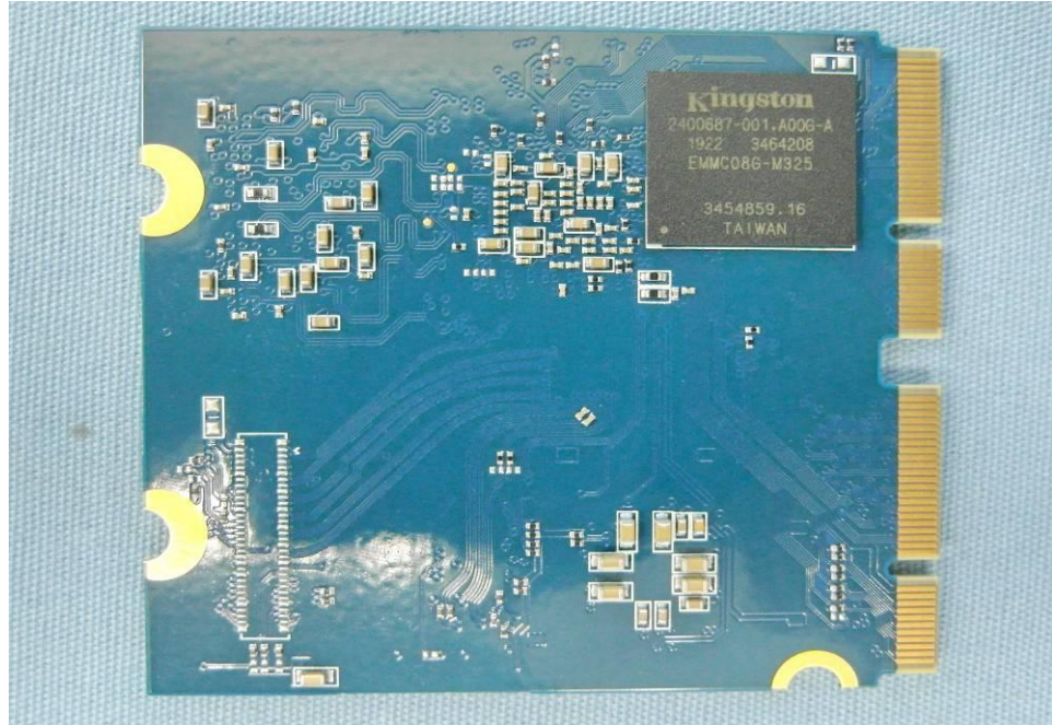
EUT Photo (3)
