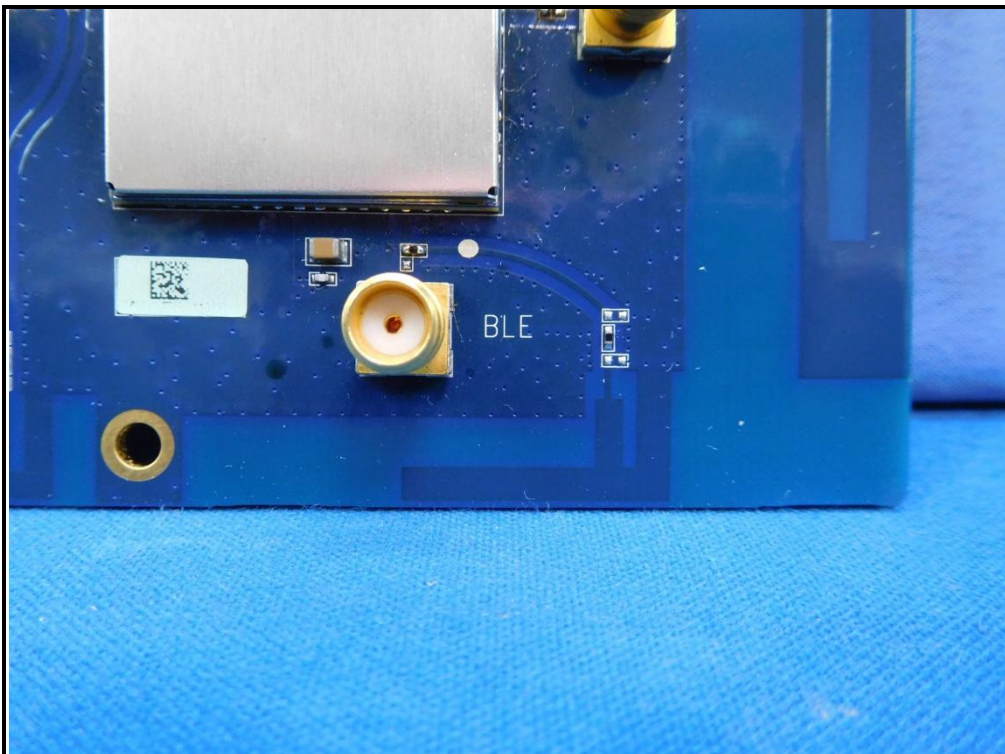
BLE antenna
