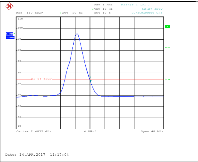
Band Edge, Right Side (Average - Horizontal)
