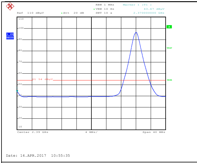
Band Edge, Left Side (Average - Horizontal)
