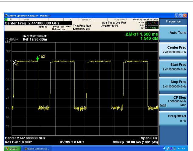
Modulation: \pi/4 DQPSK 2DH3 2441
