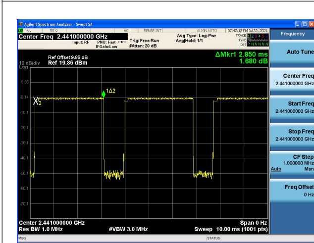
Modulation: \pi/4 DQPSK 2DH5 2441
