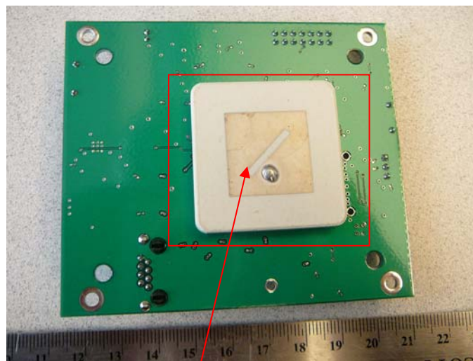
Antenna
