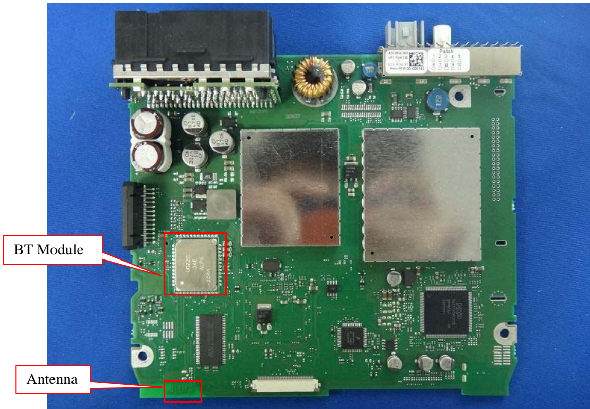
(17) EUT Photo
